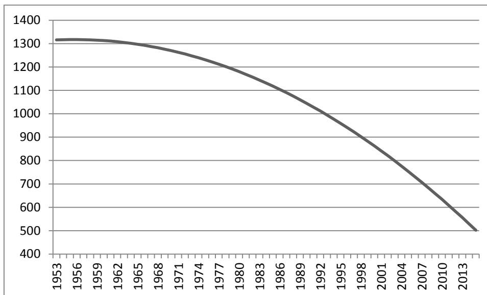
Графикон 10. Годишњи пронос наноса у Љештарској долини
