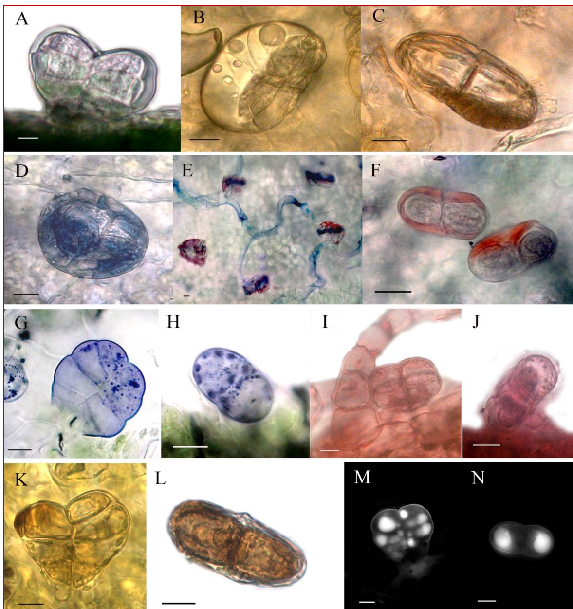
Slika 4.10. Histoheimska karakterizacija žlezdanih trihoma T. vulgare . (A) nebojena biserijatna trihoma sa vidljivim subkutikularnim prostorom; (B i C) pozitivna reakcija na hematoksilen-Sudan red 7B bojenje; (D) pozitivna reakcija na Sudan black B bojenje; (E i F) pozitivna reakcija na Nil blue bojenje; (G i H) pozitivna reakcija na NADI bojenje, (I i J) pozitivna reakcija na PAS bojenje: (K i L) pozitivna reakcija na bojenje Wagner reagensom. Bar=10 \mu m.
