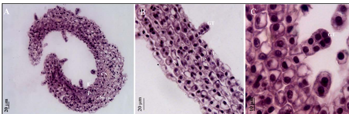
Slika 4.9. Poprečni presek lista T. vulgare . (A-C). CN-centralni nerv; E-epidermis; P-palisadni mezofil; S-sunderasti mezofil; GT-glandularna trihoma.
