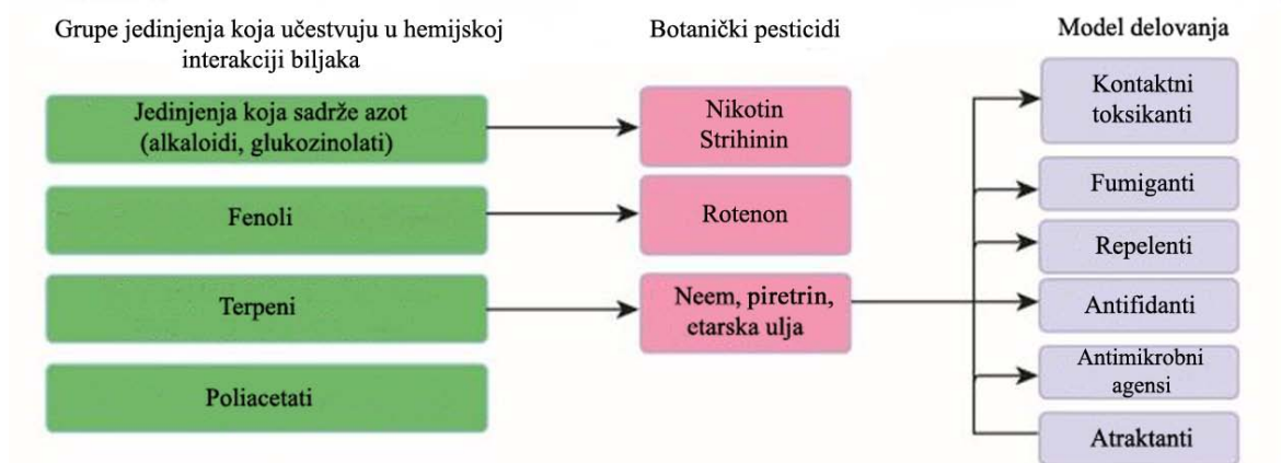
Slika 1.9. Grupe biljnih jedinjenja koje se koriste kao botanički pesticidi i njihovi modeli delovanja.
