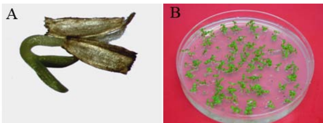
Slika 4.4. Iskljano seme T. vulgare posmatrano pod binokulranom lupom (A), klijanci (B).
