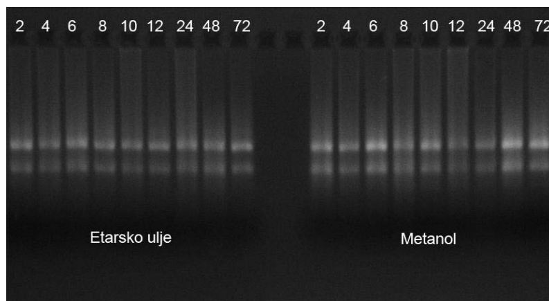
Slika 4.21. RNK izolovane iz izdanaka krompira tretiranog etarskim uljem T. vulgare ili metanolom tokom 2, 4, 6, 8, 10, 12, 24, 48 i 72 h. Na 1,2% agarozni gel nanet je po 1 \mu g ukupnih RNK za svaki uzorak.
