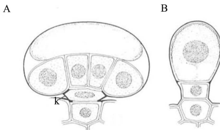
Slika 1.1. Struktura glandularnih trihoma: peltatna trihoma sa sekrecionim materijalom u subkutikularnom prostoru (A); kapitatna trihoma (B). k-kutikula. (Fahn, 1988)
