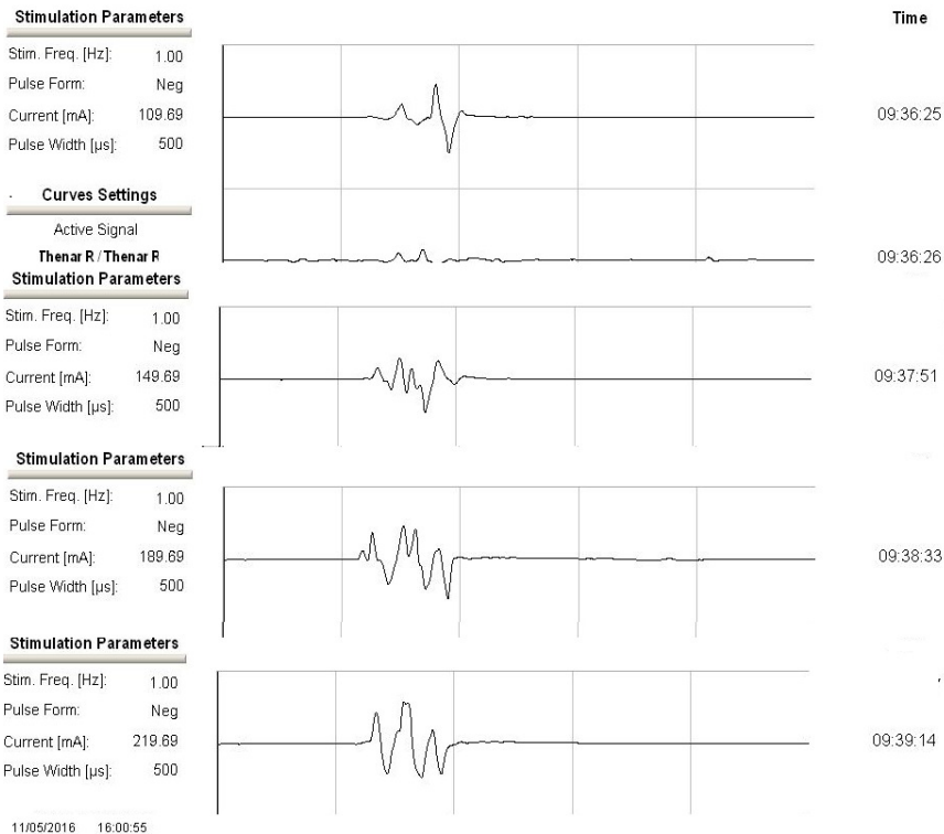
Слика 20. ДС м. 26 год: Повећање прага за десни АПБ у 9.36
