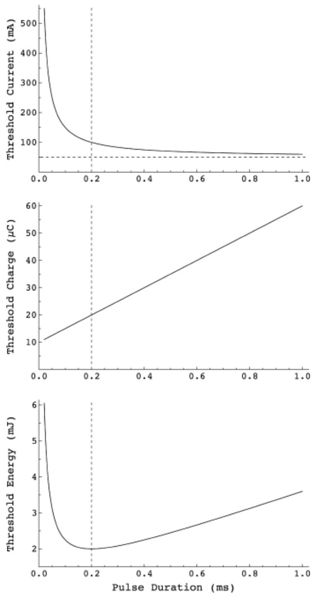
Слика 23. Струјни праг, набој и енергија импулса дужине 0.02–1.0 ms за реобазу од 50 mA (хоризонтална испрекидана линија), хронаксију 0.2 ms (вертикалне испрекидане линије) и отпор 1 k \Omega . Преузето уз дозволу издавача Elsevier Ltd.; MacDonald и сар. , 2013. ©2013.
