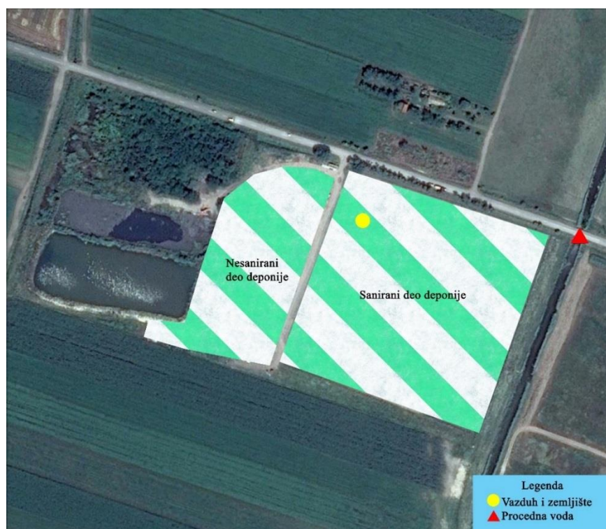
Slika 3.14 Lokacije uzorkovanja na deponiji komunalnog otpada u Temerinu
