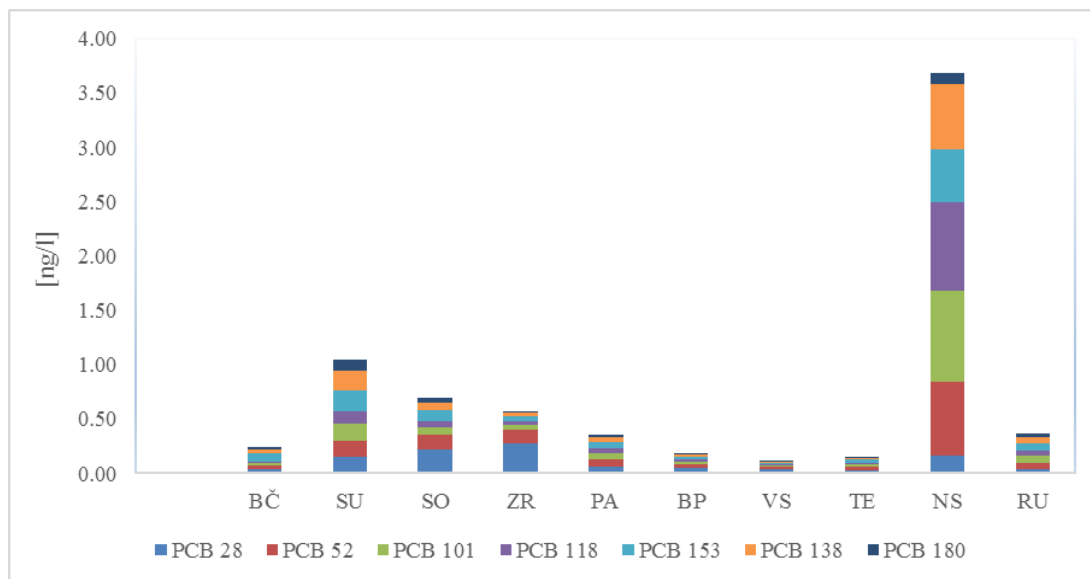
Dijagram 4.9 Koncentracijski nivoi PCB u tečnoj fazi procednih voda sa ispitivanih deponija komunalnog otpada
