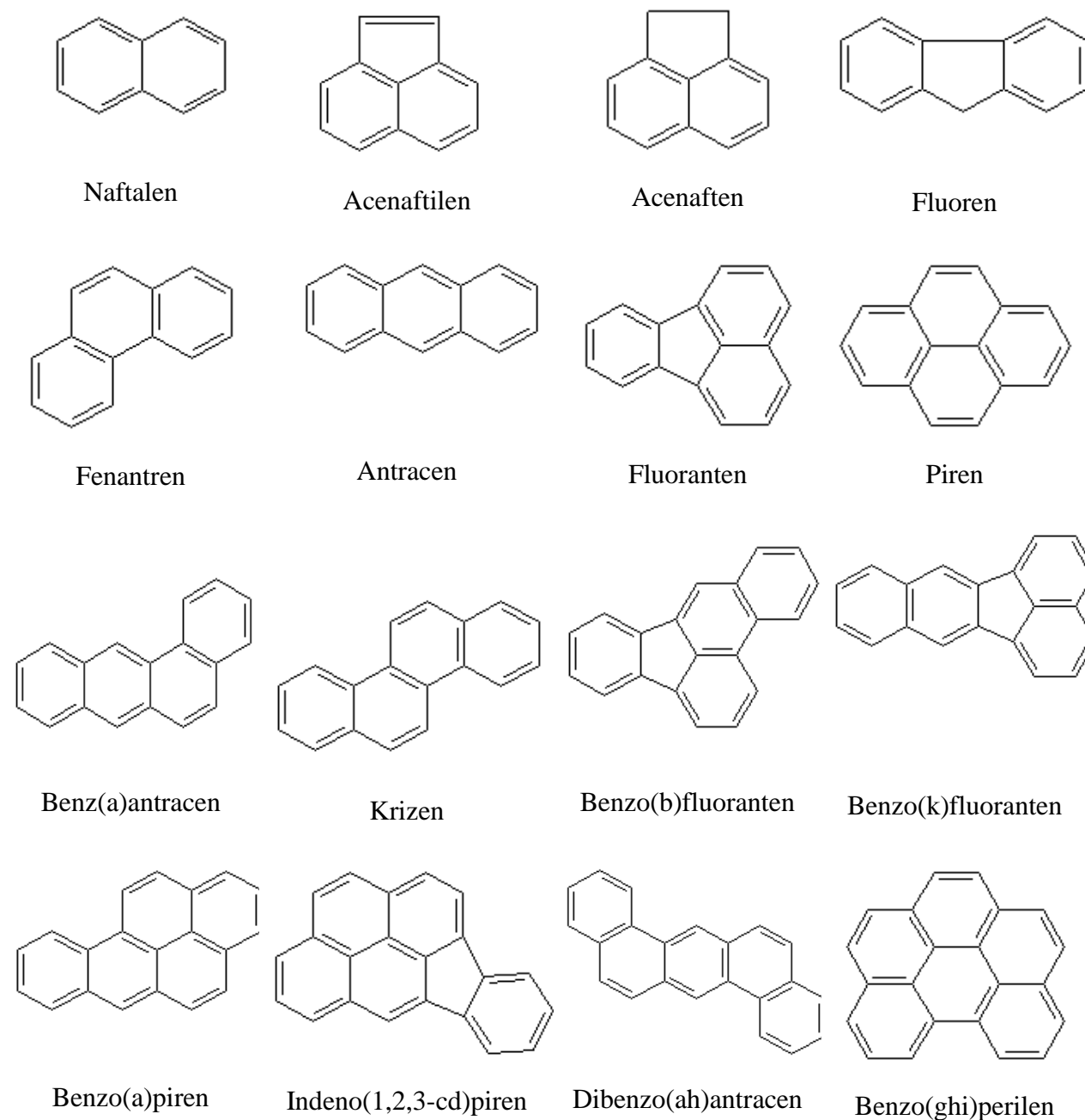
Slika 2.1 Strukturne formule 16 prioriternih PAH (Radonić, 2009)
