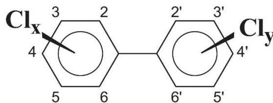
Slika 2.2 Opšta strukturalna formula PCB (Stokholmska konvencija)
