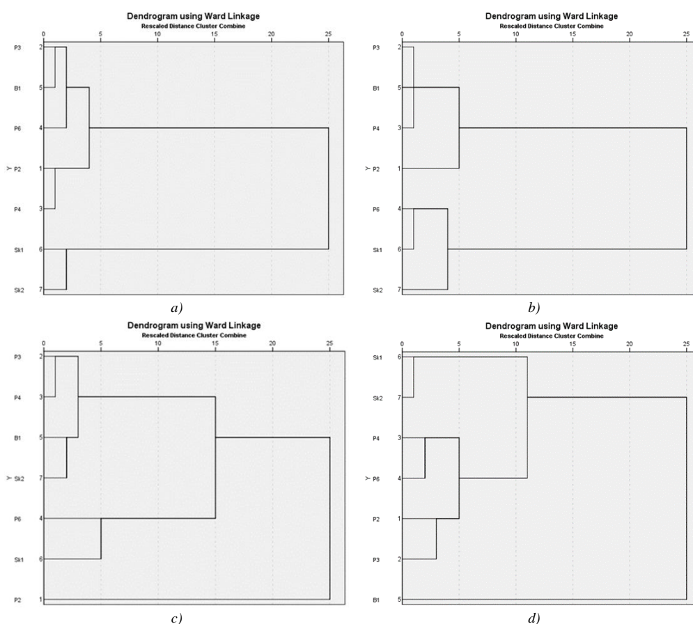
Slika 4.2 Klaster dendrogrami ispitivanih lokacija na deponiji komunalnog otpada u Novom Sadu dobijeni komparacijom sa glavnim komponentama a) PC 1, b) PC 2, c) PC 3 i d) PC 4
