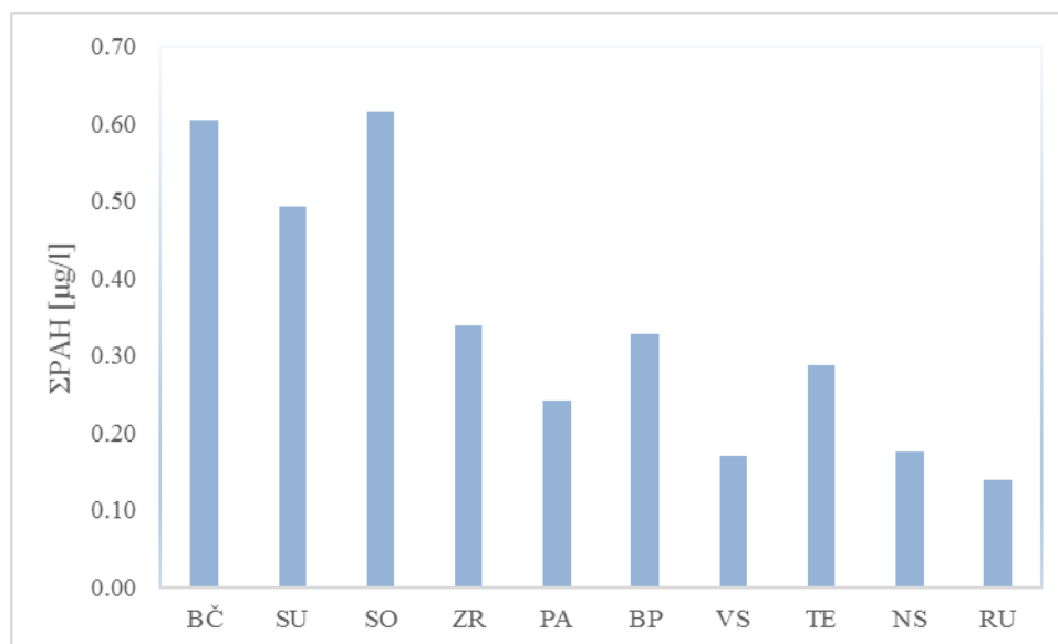
Dijagram 4.1 Ukupan sadržaj PAH u procednim vodama na ispitivanim deponijama komunalnog otpada
