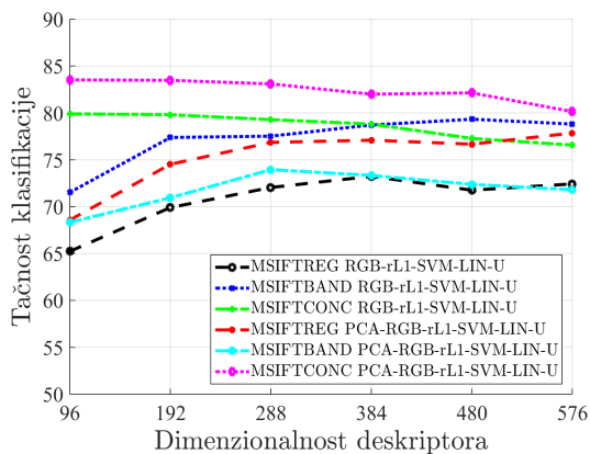
(a) UCM baza, SIFT deskriptor
