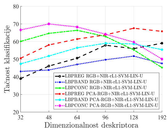
(f) NirScene baza, LBP deskriptor
