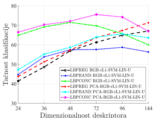
(e) UCM baza, LBP deskriptor
