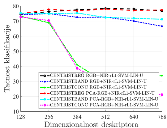
(d) NirScene baza, CENTRIST deskriptor
