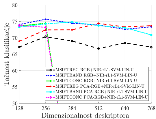
(b) NirScene baza, SIFT deskriptor
