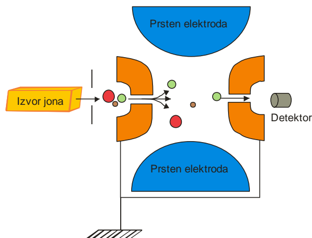
Slika 11. Shematski prikaz jon trap analizatora.
