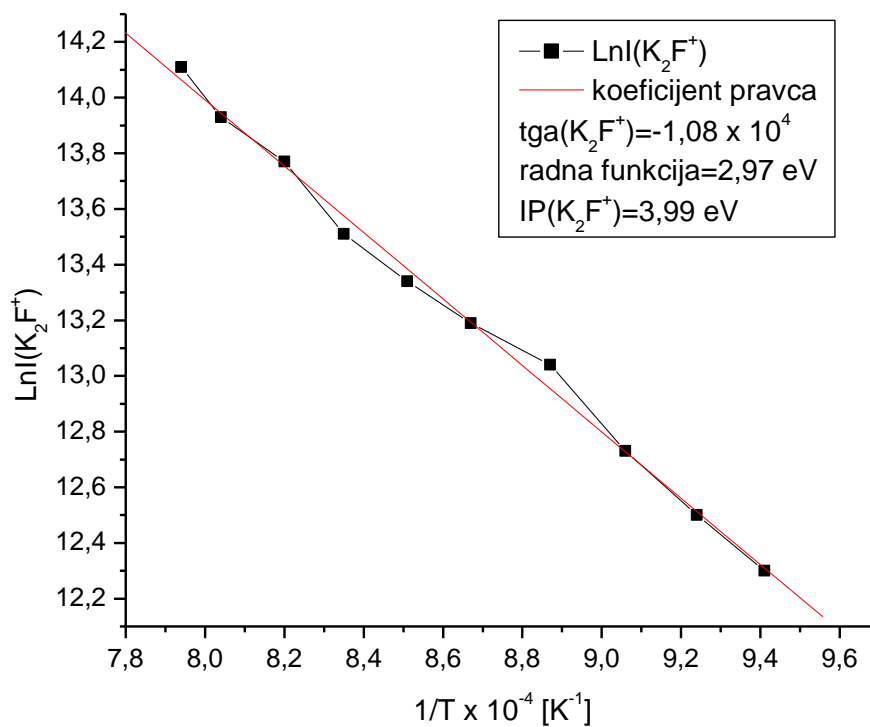
Slika 27. Eksperimentalna vrednost intenziteta jonske struje klastera \text{K}_2\text{F}^+ merena na različitim temperaturama jonizacije.
