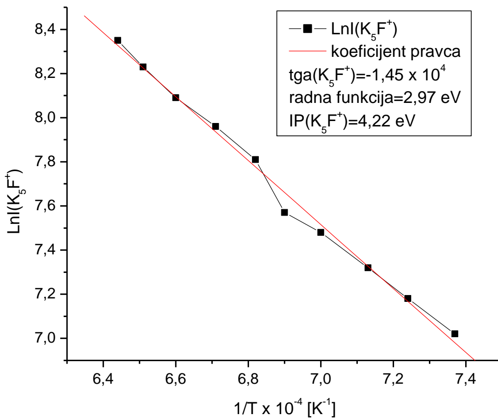
Slika 30. Eksperimentalna vrednost intenziteta jonske struje klastera K_5F^+ merena na različitim temperaturama jonizacije.
