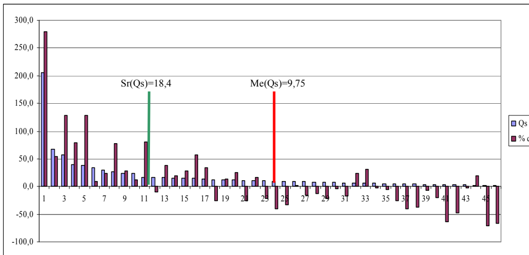
Grafik 14. Rangiranje godina po vrednosti pronosa suspendovanog nanosa (Qs) i procentualno odstupanje specifičnog oticaja (% q) od medijalne vrednosti na profilu Dimitrovgrad.
