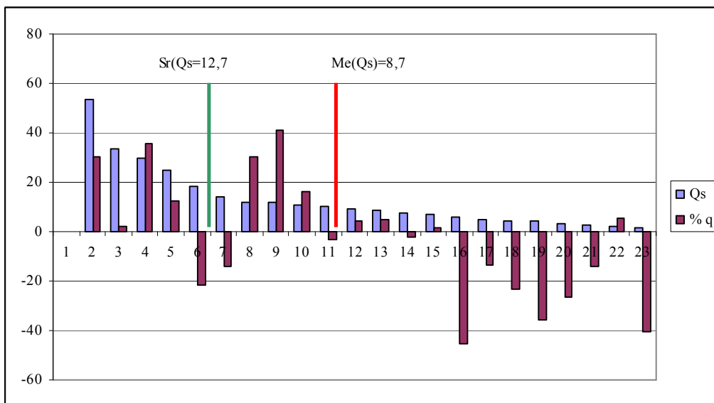
Grafik 16. Rangiranje godina po vrednosti pronosa suspendovanog nanosa (Qs) i procentualno odstupanje specifičnog oticaja (% q) od medijalne vrednosti na profilu Braćeveci.
