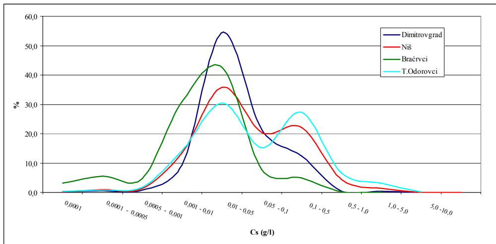
Grafik 50. Procentualna distribucija koncentracija suspendovanog nanosa Cs (g/l).
