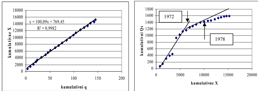
Grafik 29. Kumulativni dvostruku mas plot dijagram na nivou vremenske serije 1964-1985 -profil Trnski Odorovci
