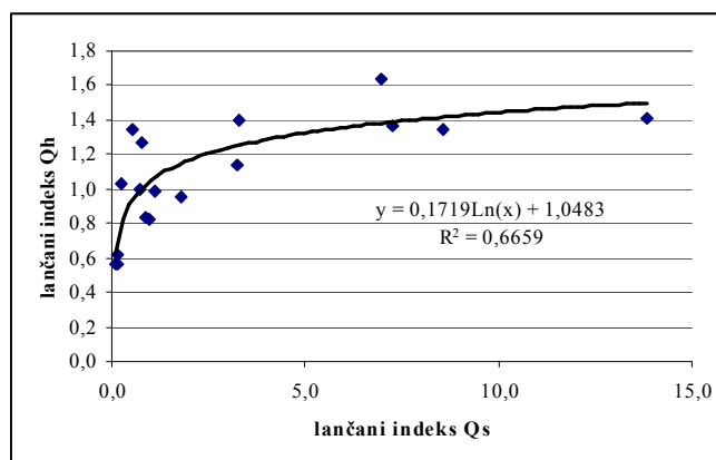
Grafik 68. Odnos između lančanih indeksa pronosa suspendovanog (Qs) i hemijskog rastvorenog (Qh)nanosa.
