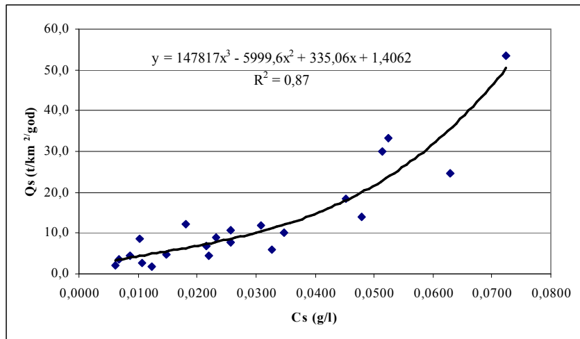
Grafik 20. Odnos izmedju srednje godišnje koncentracije suspendovanog nanosa ( C_s ) i godišnjeg specifičnog pronosa suspendovanog nanosa ( Q_s ) - profil Braćeveci.
