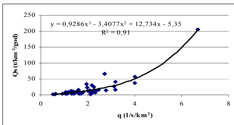
Grafik 10. Odnos izmedju srednje godišnjeg specifičnog oticaja ( q ) i godišnjeg specifičnog pronosa suspendovanog nanosa ( Q_s ) na profilu Dimitrovgrad.
