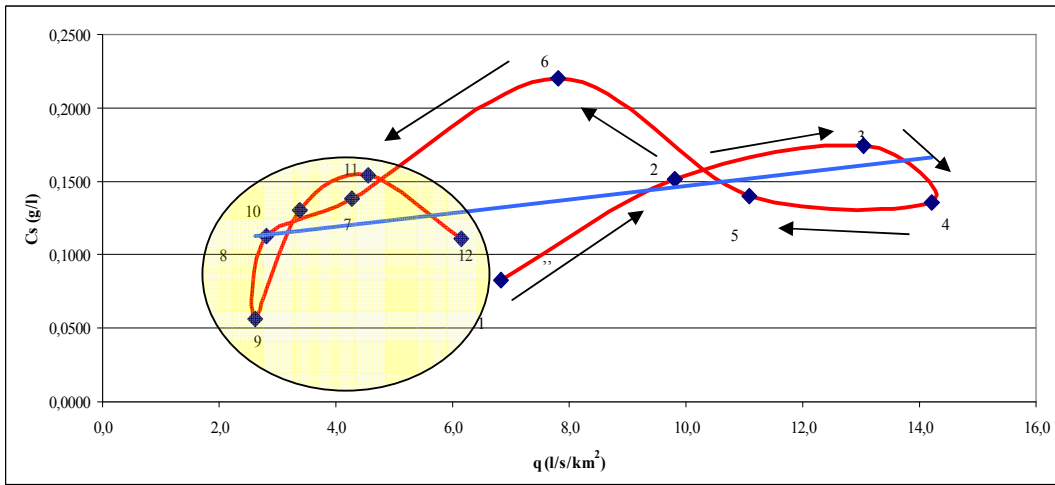
Grafik 46. Srednja godišnja histerezis petlja - profil Niš
