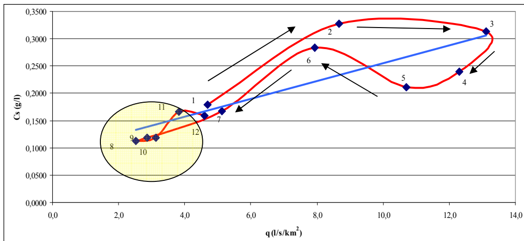
Grafik 48. Srednja godišnja histerezis petlja - profil Trnski Odorovci.
