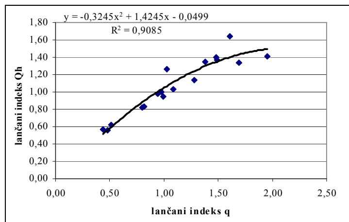
Grafik 67. Odnos između lančanih indeksa specifičnih oticaja (q) i lančanih indeksa pronosa hemijskog rastvorenog nanosa (Qh).
