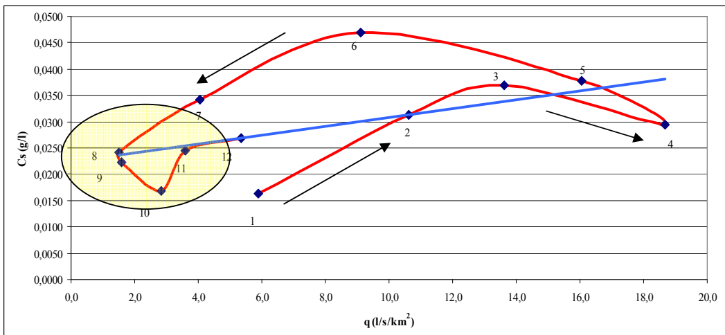
Grafik 47. Srednja godišnja histerezis petlja - profil Braćeveci.
