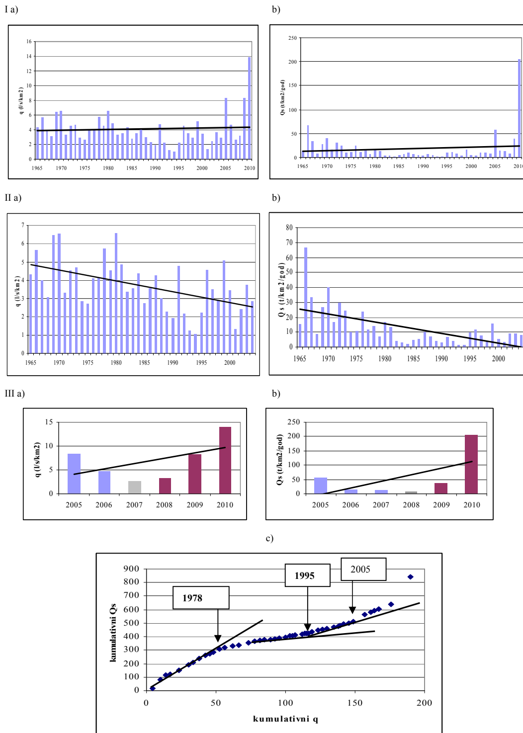
Grafik 22. Dugoročni trendovi specifičnog oticaja (a) i specifičnog pronosa nanosa (b) povezanih kumulativnim dvostrukim mas plot dijagramom (c) - profil Dimitrovgrad.
