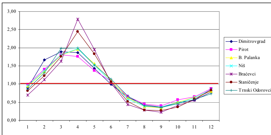
Grafik 7. Hidrogrami reka u slivu Nišave.
