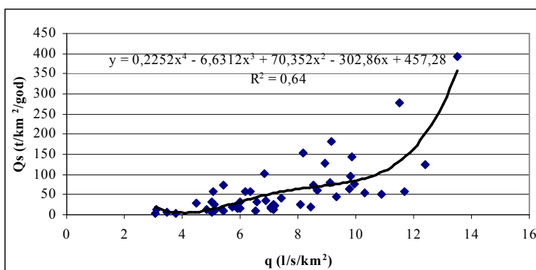
Grafik 11. Odnos između srednjeg godišnjeg specifičnog oticaja ( q ) i godišnjeg specifičnog pronosa suspendovanog nanosa ( Q_s ) na profilu Niš.
