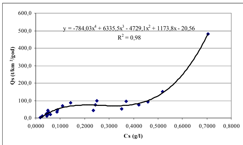
Grafik 20. Odnos izmedju srednje godišnje koncentracije suspendovanog nanosa ( C_s ) i godišnjeg specifičnog pronosa suspendovanog nanosa ( Q_s ) - profil Braćeveci.
