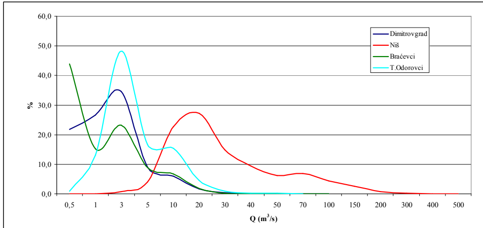
Grafik 49. Procentualna distribucija proticaja Q (m 3 /s).
