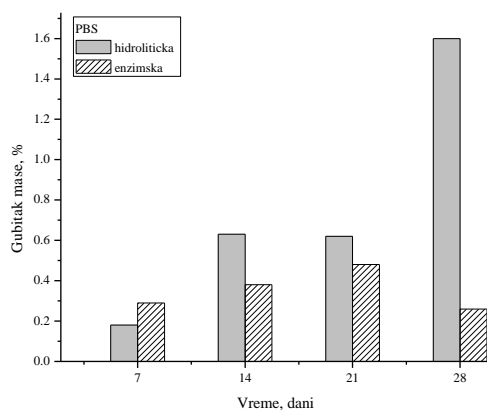
Slika 7.6.1. Hidrolitička i enzimska degradacija homopolimera PBS
