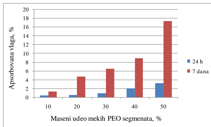
Slika 3.25 Procenat apsorbovane vlage u kopolimerima u zavisnosti od udela mekih PEO segmenata tokom 24 h i 7 dana
