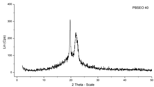
Slika 7.3.10. WAXS difraktogram kopolimera PBSE0 40
