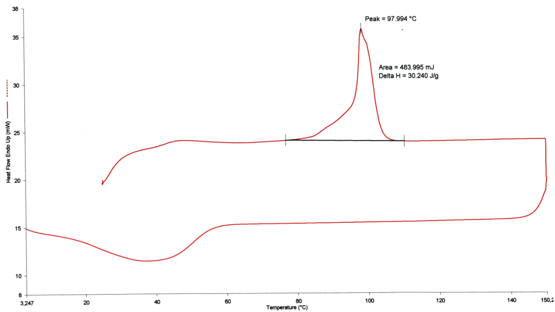
Slika 7.2.11. DSC krive grejanja (prvi prolaz) i hlađenja kopolimera PBSTMO 50
