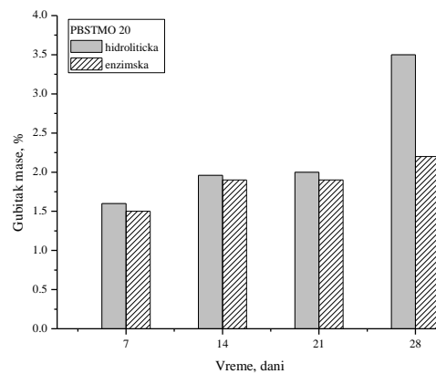
Slika 7.7.3. Hidrolitička i enzimska degradacija kopolimera PBSTMO 20
