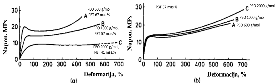
Slika 1.21 Zavisnost napon deformacija poli(estar etara) sa razliĉitim molarnim masama PEO (600, 1000 i 2000) i masenim udelima PBT: a) 67 mas.% (A), 57 mas.% (B) i 41 mas.% (C); b) 57 mas.% (A, B i C)
