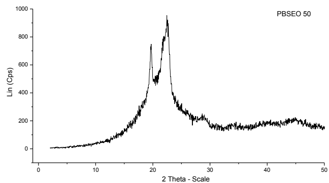
Slika 7.3.11. WAXS difraktogram kopolimera PBSE0 50
