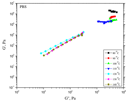
Slika 7.5.1. Zavisnost G' od G'' homopolimera PBS pri različitim temperaturama
