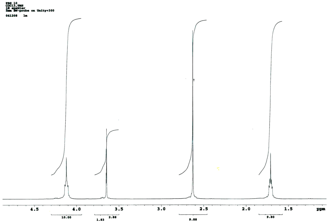
Slika 7.1.7. ^1\text{H} NMR spektar kopolimera PBSE0 10
