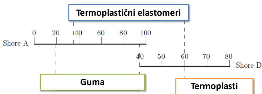
Slika 1.9 Skala tvrdoće po Shore -u za termoplaste, gumu i termoplastične polimere [107]
