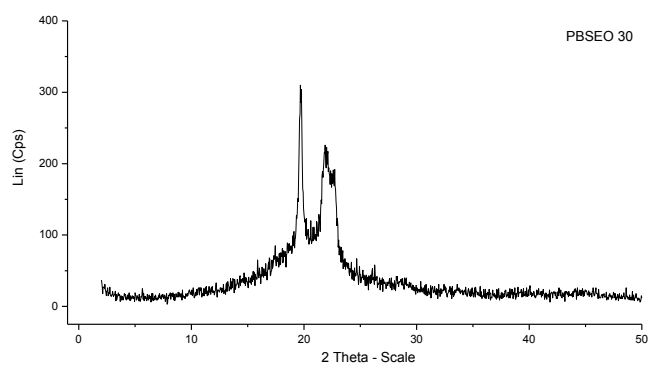
Slika 7.3.9. WAXS difraktogram kopolimera PBSE0 30
