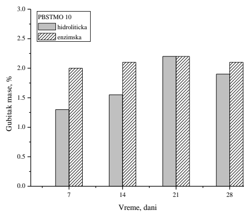
Slika 7.6.2. Hidrolitička i enzimska degradacija kopolimera PBSTMO 10
