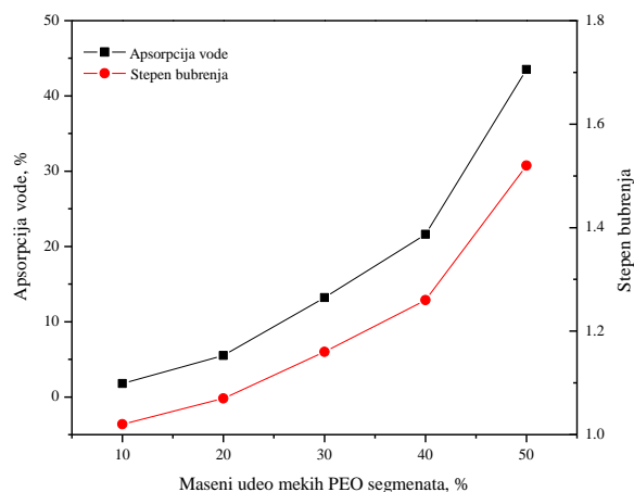
Slika 3.24 Procenat apsorbovane vode i ravnotežni stepen bubrenja kopolimera sa promenom udela mekih PEO segmenata u toku 24 h
