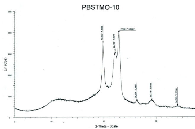
Slika 7.3.2. WAXS difraktogram kopolimera PBSTMO 10
