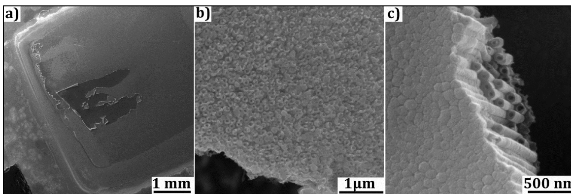
Slika 45. Izrazito oštećen anodizirani transparentni film na FTO staklu: a) mala površina filma je ostala na FTO staklu, b) poprečni presek nanocevi slikano na raslojenom filmu i c) konično dno nanocevi sa heksagonalnom geometrijom.
