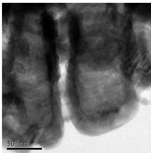
Slika 25. HRTEM analiziranog dela nanocevi NC250
