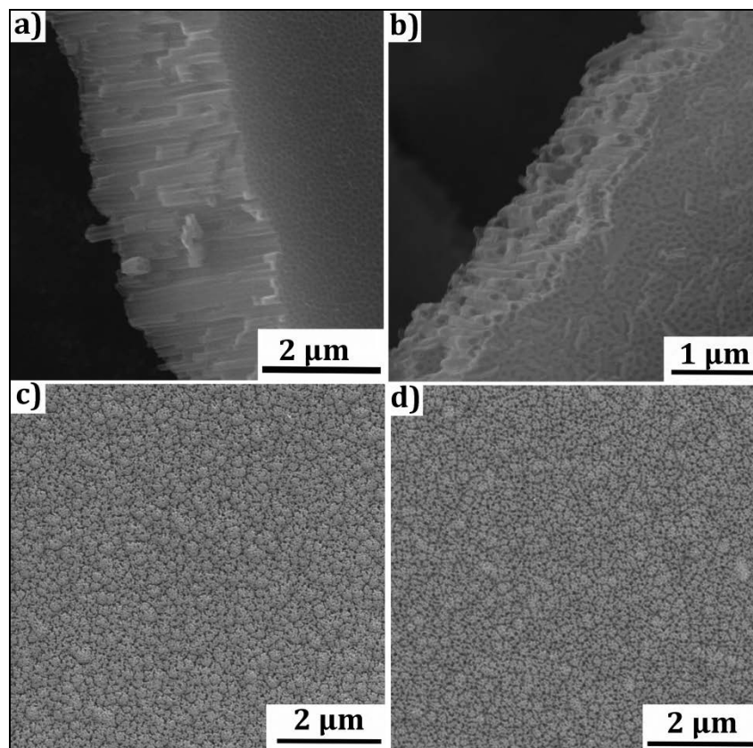
Slika 61. FESEM slike anodizovanih TiO 2 nanocevi: a) i b) pre žarenja (visina ~2,5 μm, prečnik ~60 nm), c) nakon žarenja u vazduhu, d) nakon žarenja u NH 3 .
