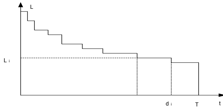
Slika 3.7. Aproximativna kriva trajanja potrošnje
