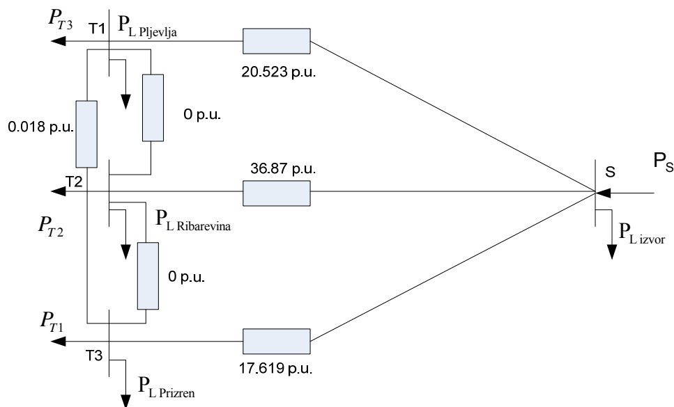
Slika 7.1. Ekvivalentna šema sistema Srbije
