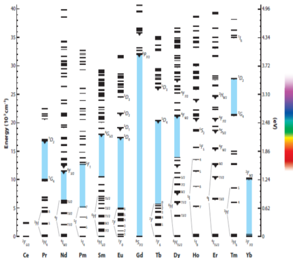
Slika 3.3. Diekov dijagram
