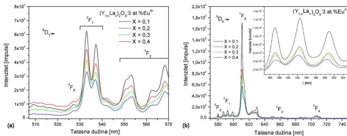
Slika 8.22. Emisioni spektri uzoraka (\text{Y}_{1-x}\text{La}_x)_2\text{O}_3:3 \text{ at}\% \text{Eu}^{3+} ( x = 0.1 - 0.4 ) snimani sa \lambda_{\text{exc}} = 393 \text{ nm} u oblastima: (a) 500–570 nm; (b) 570–750 nm. Štarkovo cepanje ^7\text{F}_1 nivoa je uvećano i ubačeno kao dodatak na slici (b)
