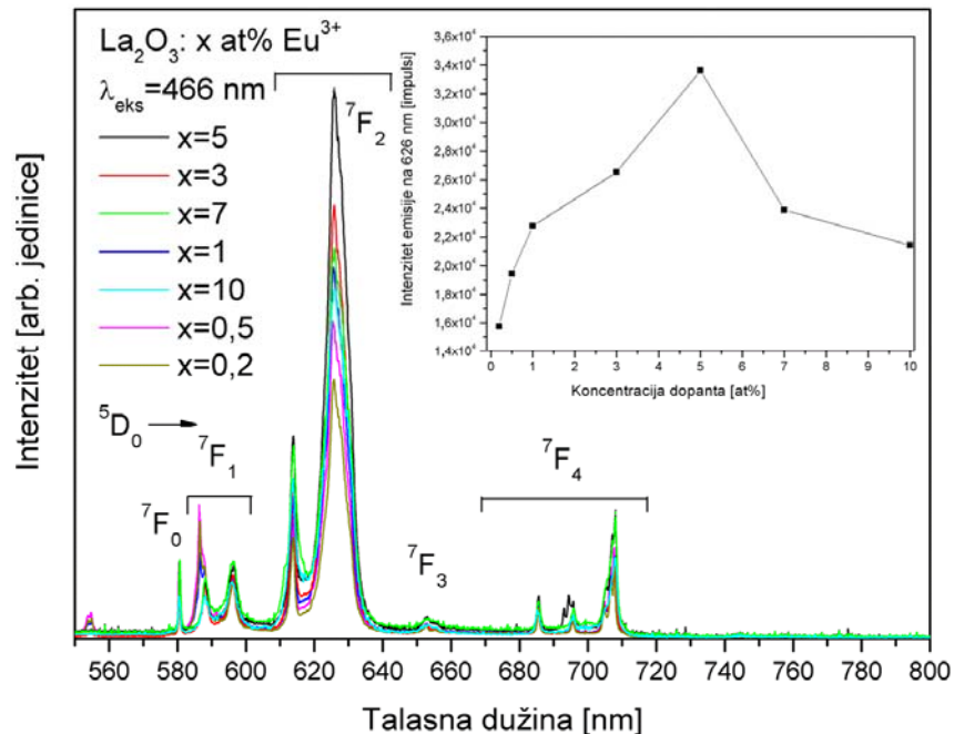
Slika 8.12. Emisioni spektri uzoraka \text{La}_2\text{O}_3: x \text{ at}\% \text{Eu}^{3+} ( x = 0,2; 0,5; 1; 3; 5; 7 i 10 ), \lambda_{\text{eks}} = 466 \text{ nm} , snimani na sobnoj temperaturi, sa ubačenim delom zavisnosti intenziteta emisije od koncentracije dopanta
