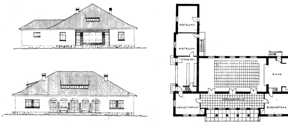
Слика 5.11 - Задружни дом тип 1, архитект Димитрије Маринковић.
