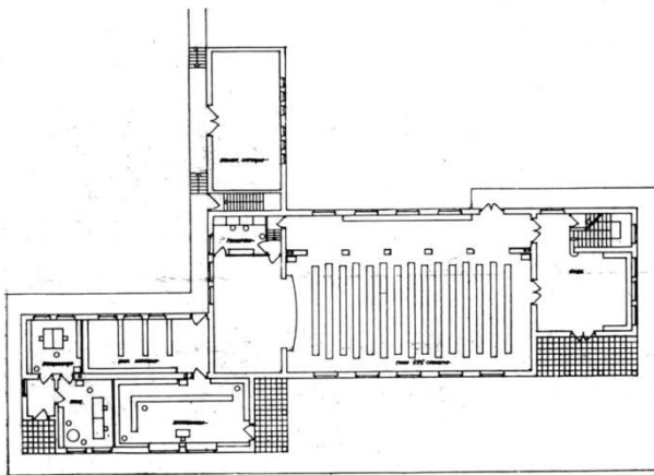
План prizemlja • План нижњег етажa • Plan du rez-de-chaussée
