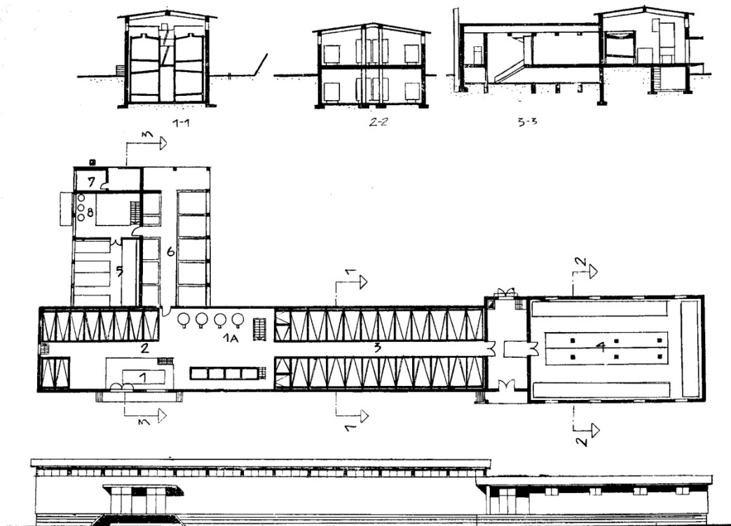
Слика 5. 33 – Полуукопани подрум за вино у селу Рајац капацитета 150 вагона, Према пројекту „Инвест завода“ Београд. Бранислав Којић и Ђорђе Симоновић, Пољопривредне зграде и комплекси (Београд: Грађевинска књига, 1978), 163.
