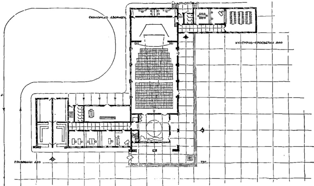
Слика 5.5 - Задружни дом тип 7, арх Никола Гавриловић. Milorad Macura, „Zadružni domovi na teritoriji NR Srbije“, Arhitektura, br. 11-12 (1948): 31.
