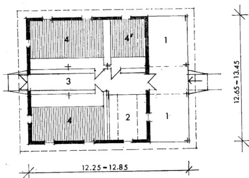
Слика 5. 41 – Стаја за тов 50 телаци до 220 кг тежине, Према типском пројекту бироа „Наш стан – ИАУС“ Београд
