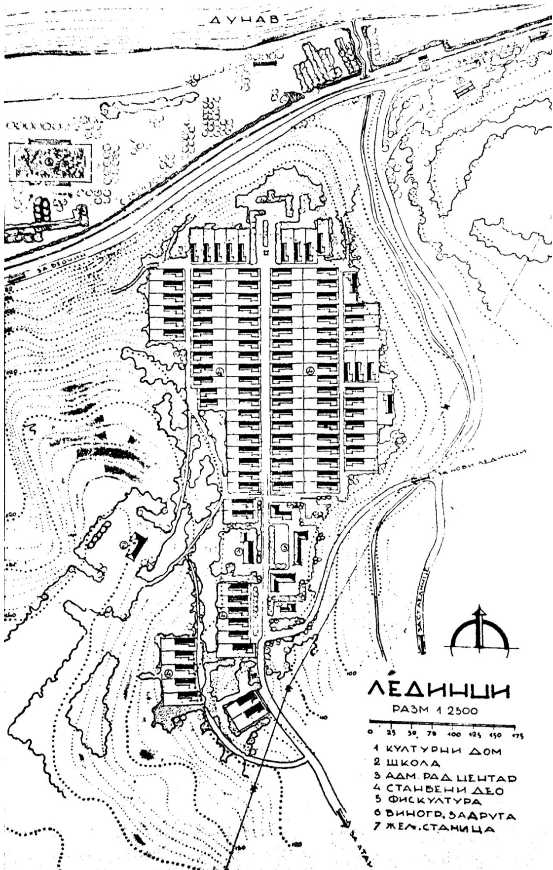
Слика 4.9 – Реконструкција сеоског насеља Лединци на Фрушкој Гори. Saša Sedlar, „Pitanje planske izgradnje sela u Srbiji“, Tehnika , br.1 (1946):130.
