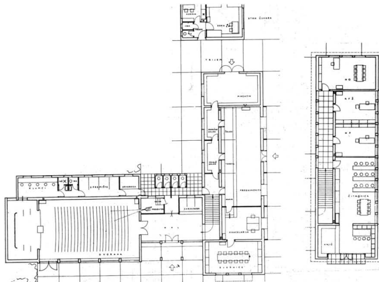
Слика 5.8 - Задружни дом тип 9, арх Божидар Гушек. „Типови задружних домова у НРН“, Arhitektura , br. 7 (1948):15.
