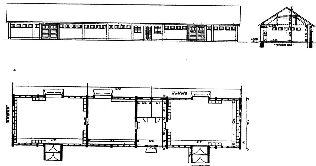
Слика 5. 37 – Типска стаја за подмладак коња до узраста од три године, Пројектант Р. Кадић, према пројектима пољопривредних зграда Министарства грађевина ФНРЈ, 1950.
