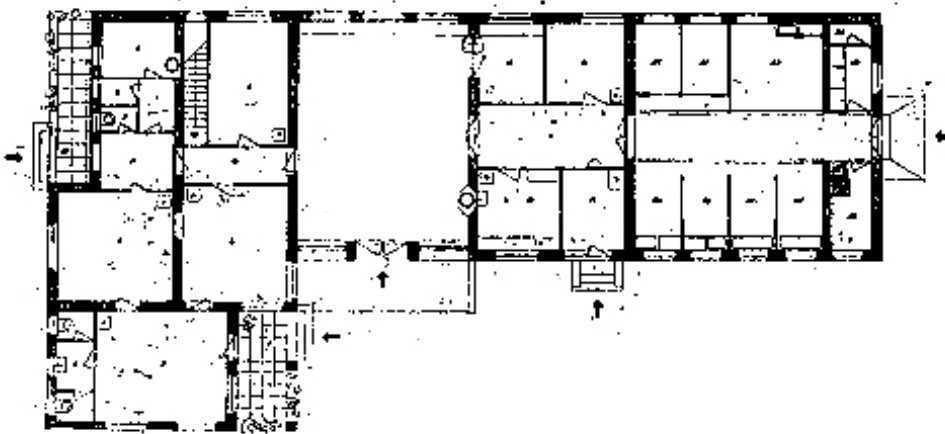
Слика 5. 64 – Тип ветеринарске амбуланте изведене у Запрешћу код Загреба. Zvonimir Crnokrak i Zvonimir Strunjak, „Veterinarske ambulante“, Urbanizam-arhitektura br. 9-12 (1951): 37.
