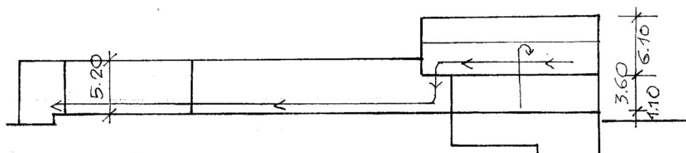
Слика 5. 35 б – Шематски приказ индустријског погона пекаре у Нишу капацитета 84 000 кг хлеба.
