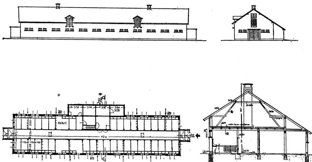
Слика 5. 38 – Типска коњушница за тридесет и осам радних грла са три бокса, са посебном спремницом хране и складиштем за зрнасту храну, Пројектант Р. Кадић, према пројектима пољопривредних зграда Министарства грађевина ФНРЈ, 1950.
