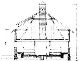
Слика 5. 61 – Тип стаје за телад са кравама хранилицама, Пројектант: Звонимир Црнокрак. Zvonimir Crnokrak „Staje za goveda“, Urbanizam-Arhitektura , br. 9-12 (1951): 19.
