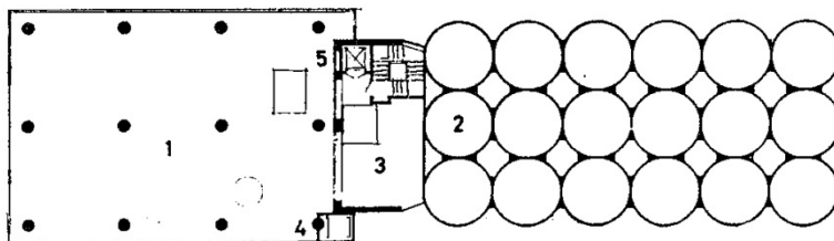
Слика 5.1 г – Силос у Сенти. Бранислав Којић и Ђорђе Симоновић, Пољопривредне зграде и комплекси (Београд: Грађевинска књига, 1978), 76.
