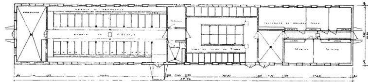
Слика 5. 61 – Тип стаје за телад са кравама хранилицама, Пројектант: Звонимир Црнокрак. Zvonimir Crnokrak „Staje za goveda“, Urbanizam-Arhitektura , br. 9-12 (1951): 19.
