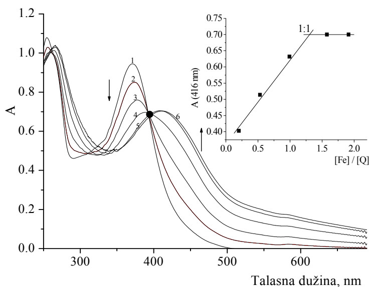
Slika 4.3. Apsorpcioni spektri kvercetina i nagrađenih kompleksa pri različitim moljskim odnosima kvercetin: gvožđe(III) na pH = 7: (1) 1:0; (2) 1:0,20; (3) 1:0,53; (4) 1:0,10; (5) 1:1,57; (6) 1:1,91. Gore: apsorbancija kompleksa na 416 nm u funkciji odnosa koncentracija [\text{Fe}]/[\text{Q}] [214]
