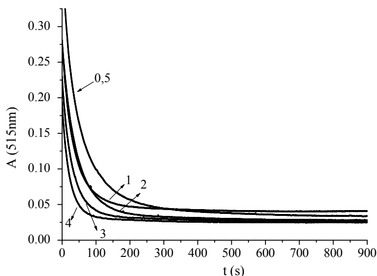
Slika 4.47. Zavisnost apsorbancije rastvora DPPH (50 \mu M) od vremena pri različitim molskim odnosima baikalein/DPPH (molski odnosi prikazani na slici)
