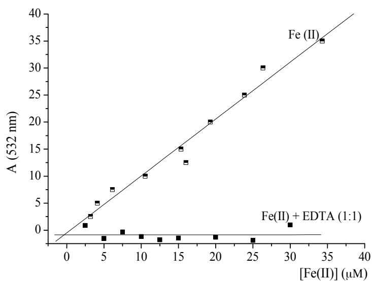
Slika 4.51. Grafik zavisnosti absorbancije malonaldehid-TBA kompleksa na 532 nm u funkciji različitih koncentracija gvožđe(II) jona u odsustvu i prisustvu ekvimolarnih koncentracija EDTA [216]
