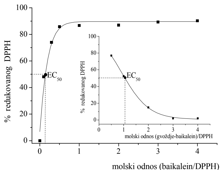
Slika 4.49. Zavisnost procenta redukovanoг DPPH u funkciji molskog odnosa baikalein/DPPH ([DPPH] = 50 \mu\text{M} ). Umetnuta slika: Zavisnost procenta redukovanoг DPPH u funkciji molskog odnosa (gvoždje- baikalein)/DPPH ([DPPH] = 50 \mu\text{M} )
