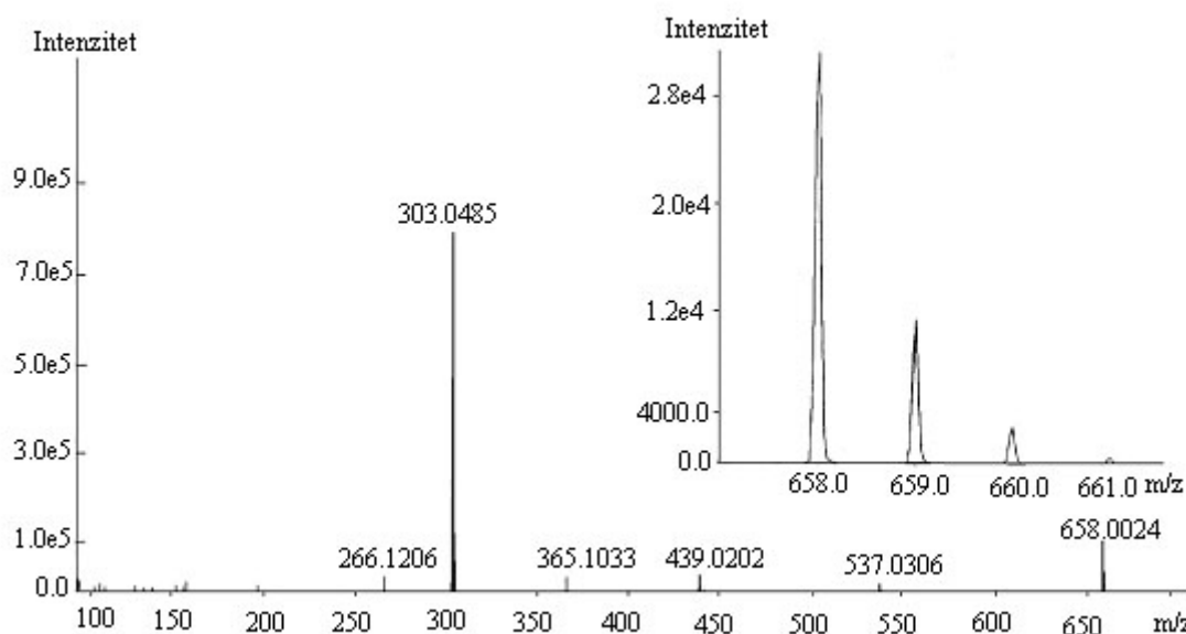
Slika 4.18. Maseni spektri kompleksa gvožđe(III)-kvercetin u smeši voda-metanol (1:1). Gore: izotopski sastav linije na m/z = 658 [214]
