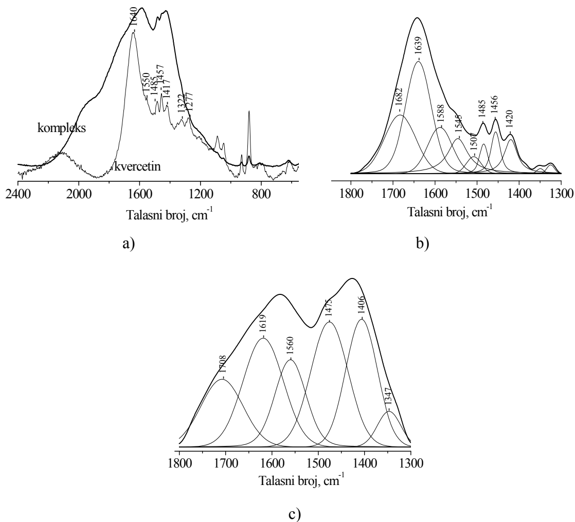
Slika 4.22. Ramanski spektr kvercetina i kompleksa gvožđe(III)-kvercetin na pH = 4 (a); razloženi spektr kvercetina na pH = 4 (b); razložen spektr kompleksa gvožđe(III)-kvercetin (1:2) na pH = 4 (c) [214]
