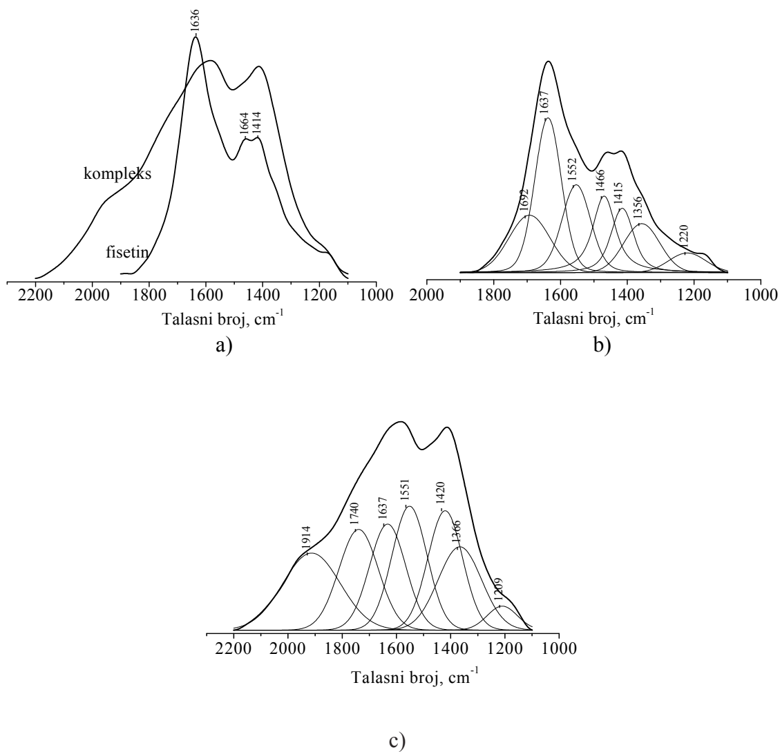
Slika 4.25. Ramanski spektar fisetina i kompleksa gvožđe(III)-fisetin na \text{pH} = 9 (a); razložen spektar fisetina na \text{pH}=9 (b); razložen spektar kompleksa gvožđe(III)-fisetin (1:1) na \text{pH} = 9 (c) [215]
