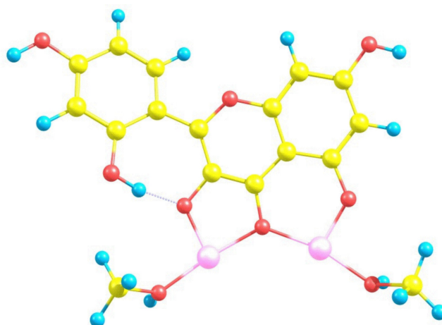
Slika 4.34. Geometrijski optimizovana struktura gvožđe(II)-morin kompleksa (2:1) i izračunati elektronski spektar [216]
