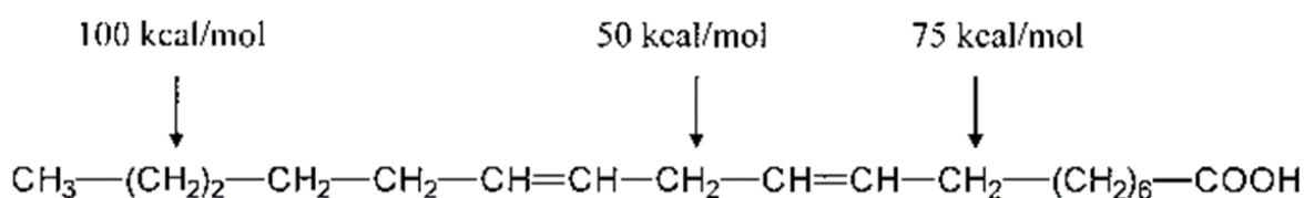
Slika 4. Energija potrebna za uklanjanje atoma vodonika u zavisnosti od njegovog položaja u molekulu masne kiseline [26].
