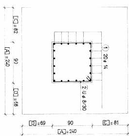
ПРЕГЛЕД 2-2
