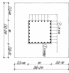
ПРЕСЕК 2.2
