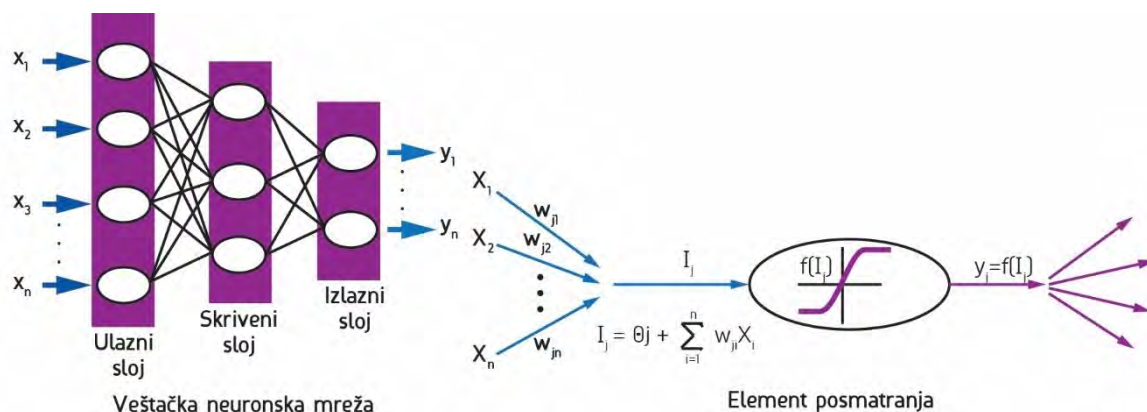
Slika 2.31 Tipična struktura i funkcionisanje veštačke neuronske mreže
