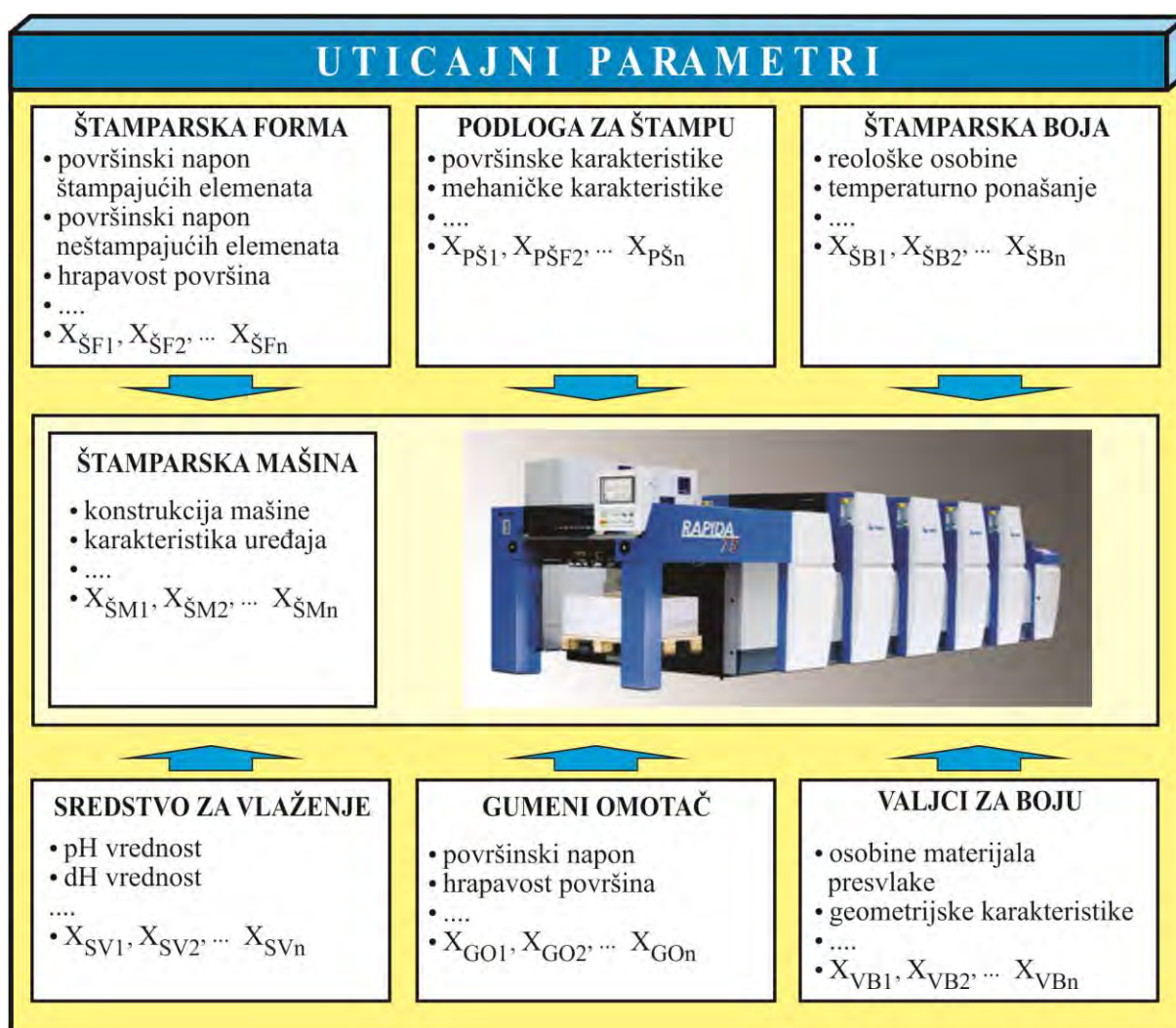
Slika 4.2 Osnova modela za razvoj savremenog sistema za identifikaciju procesnih parametara ofset štampe
