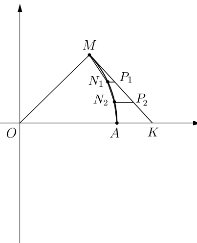
Slika 46 – Aproksimacija luka
