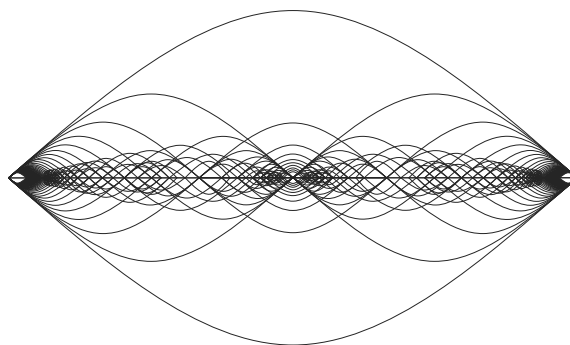
Slika 41 – Lambdome
