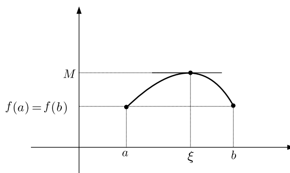
Slika 3 – Rolova teorema
