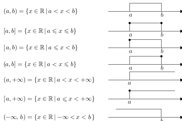
Slika 11 – Intervali
