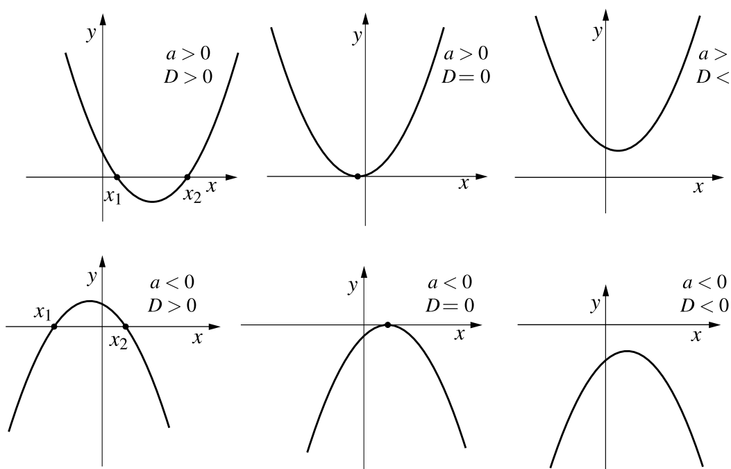
Slika 16 – Grafik kvadratne funkcije (šest slučajeva)
