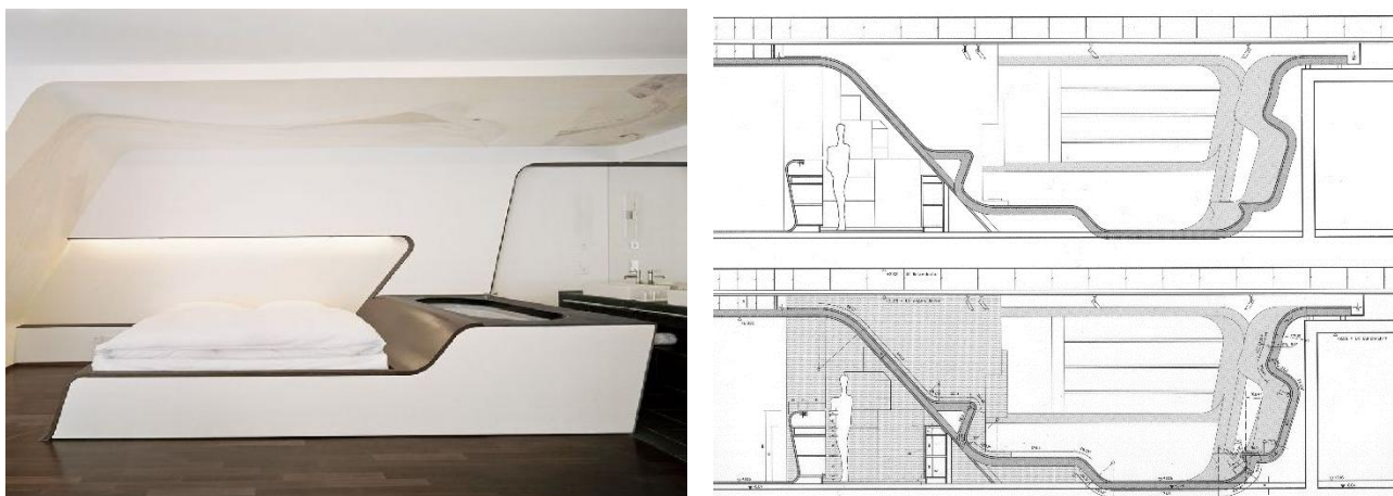
Ilustracija 4.5.11 a) enterijer sobe; b) parcijalni presezi kroz zakrivljenu monolitnu površinu u prizemlju. Izvor: (Minguet, 2009)
