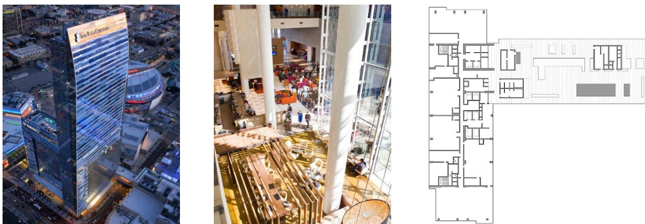
Ilustracija 4.3.7 a) spoljašnji izgled; b) hol JW Marriott hotela; c) osnova 26. Sprata. Izvor: (Penner, et al., 2013)
