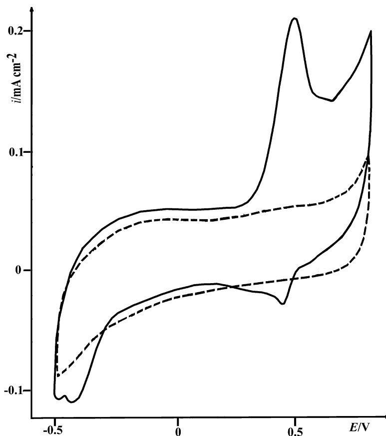
Slika 49. Ciklični voltamogrami ugljenične staklene elektrode u 0,05 M NaHCO 3 (isprekidana linija) i nakon dodatka Ni(II) kompleksa (puna linija), koncentracija 2,0 \times 10^{-2} mg·cm -3 , brzina promene potencijala: 50 mV s -1 .
