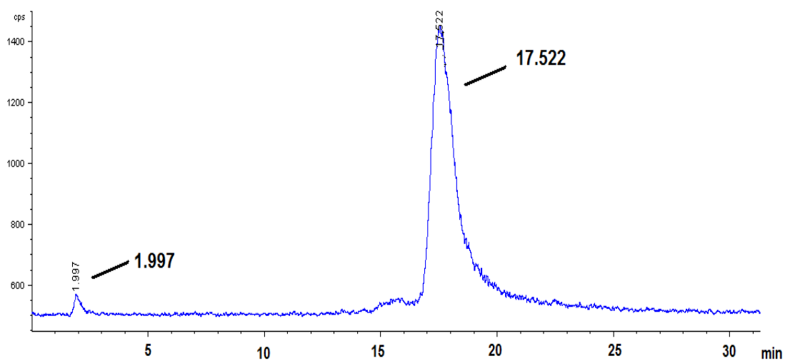
Slika 27. HPLC radiohromatogram ^{99m}\text{Tc} -L-2 kompleksa 1 h nakon obeležavanja
