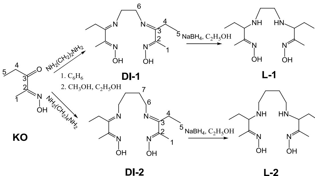
Šema 1. Sintetski put za jedinjenja L-1 i L-2
