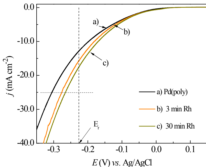
Slika 3.50. Polarizacione krive za izdvajanje vodonika na Pd(poly) i Rh/Pd(poly) elektrodama snimljene u rastvoru 0.5 M H 2 SO 4 pri brzini promene potencijala od 10 mV/s.
