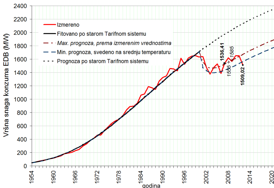
Slika IX.3 Prognoza godišnjeg vršnog opterećenja integralnog konzumnog područja EDB do 2021. i ostvarena vršna opterećenja, bez direktnih potrošača, do zimske sezone 2012/13.
