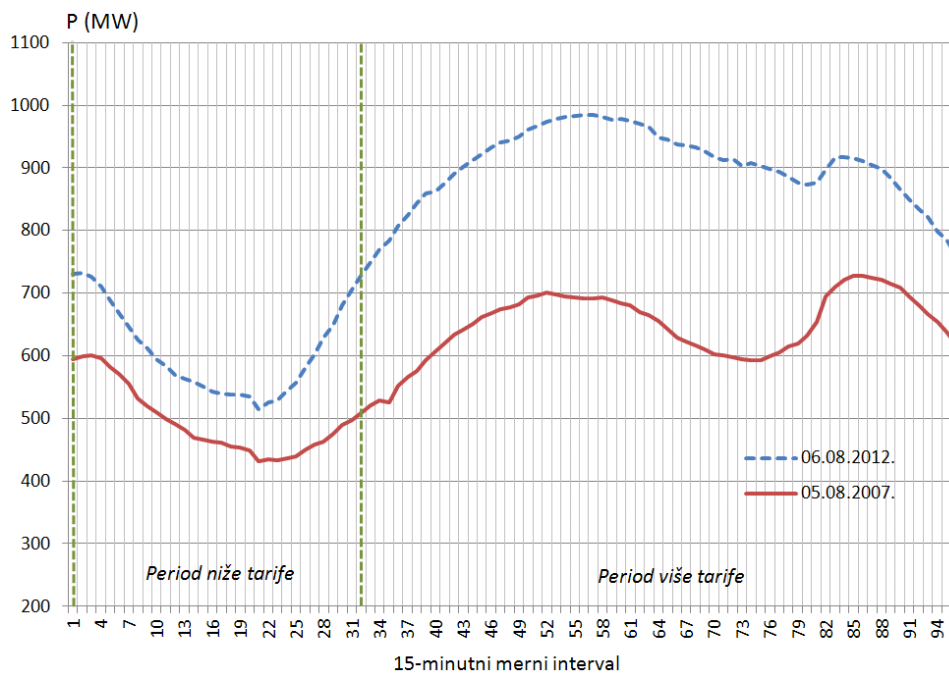
Slika V.16 Par dnevnih dijagrama opterećenja za približno isti datum u leto 2012. i 2007, sa oprečnim meteorološkim prilikama
