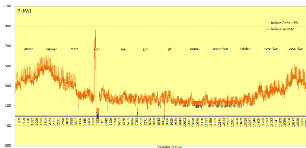
Slika VII.14 Smanjenje varijacija opterećenja kombinovanom primenom varijante 1 DSM programa i 300 PV panela
