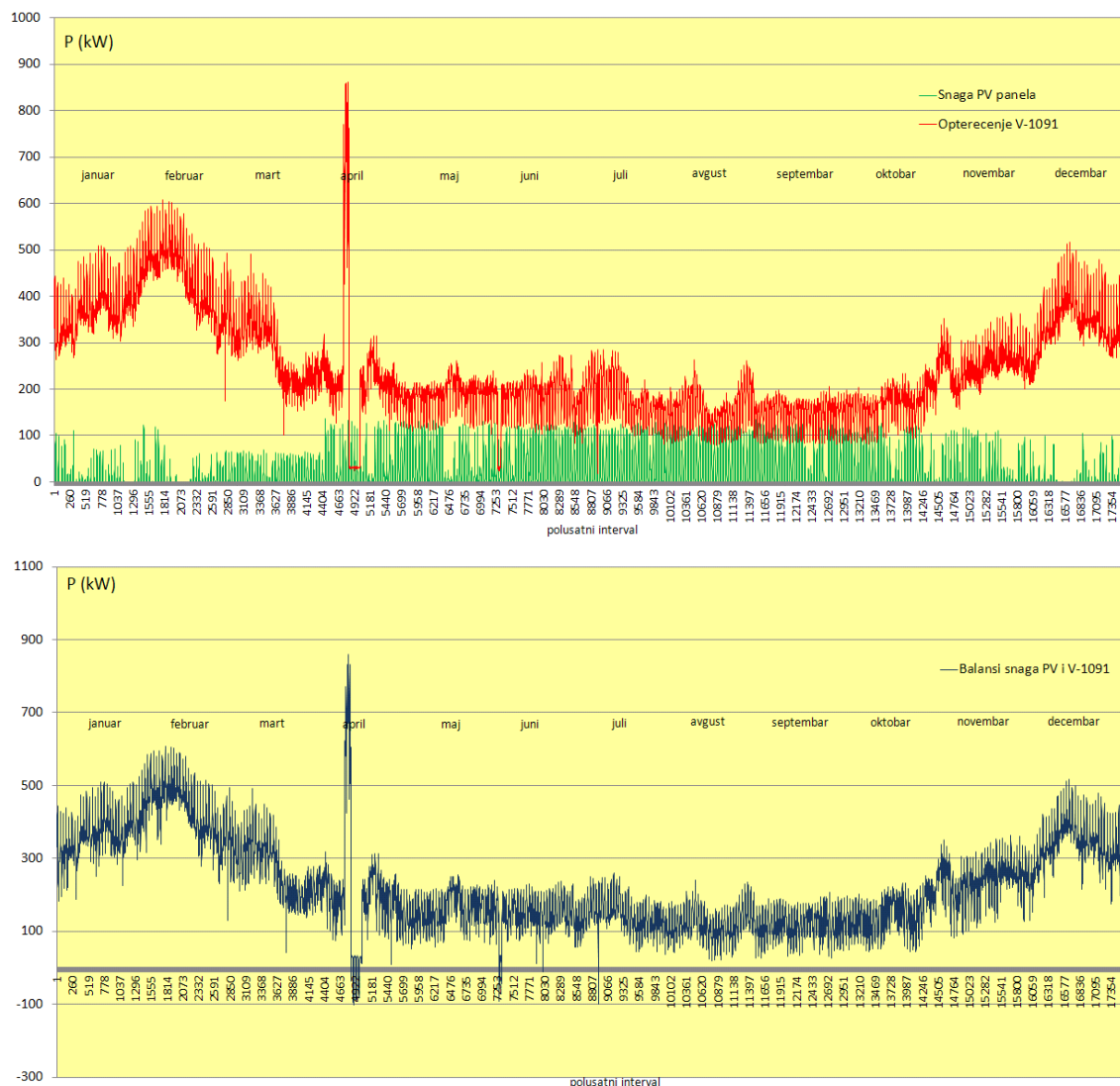
Slika VII.4 Snage potrošnje V-1091 i proizvodnje iz 600 PV-panela snage po 250 W (gornji grafici) i ukupna, balansirana snaga „na pragu“ TS V-1091 (donji grafik)
