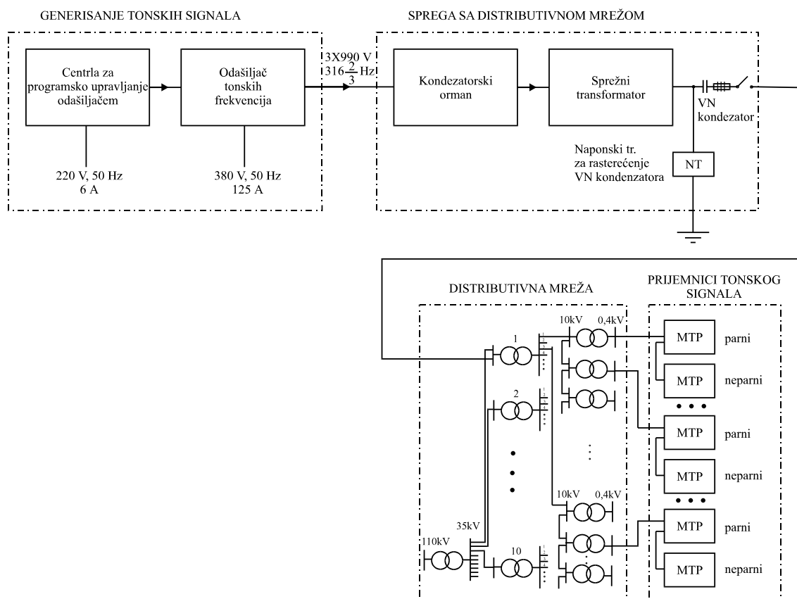
Slika III.11 Blok-šema sistema mrežne ton-frekventne komande (MTK) u Smederevskoj Palanci, sa načinom razvrstavanja potrošača u dve grupe (prema parnim i neparnim kućnim brojevima); /izvor: [III.3]/
