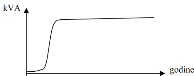
Slika IX.6 Tipična dinamika opterećivanja konzumnog područja TS SN/NN
