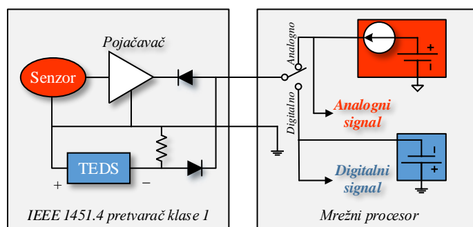
Slika 4.7. Povezivanje pretvarača korišćenjem mešovitog interfejsa klase 1 [21]
