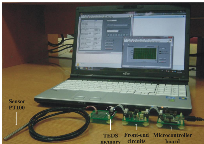
Slika 5.11. Realizovani sistem za testiranje Plug and Play temperaturnog senzora
