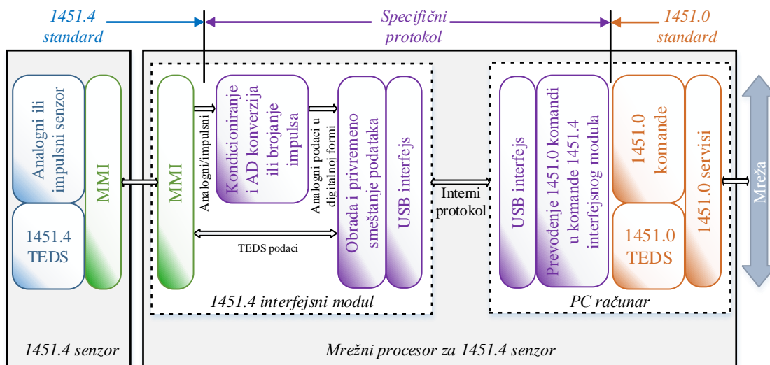
Slika 5.8. Koncepcija 1451.4 mrežnog procesora
