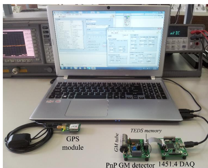
Slika 5.16. Realizovani sistem za testiranje Plug and Play GM detektora
