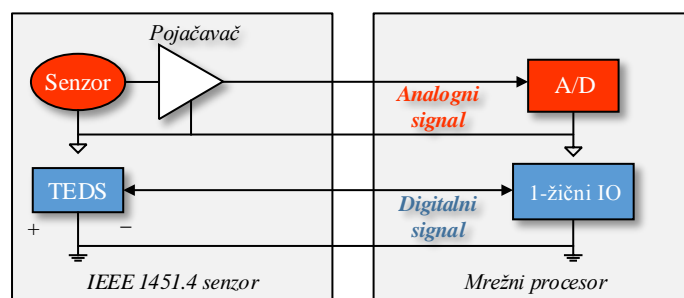
Slika 4.8. Povezivanje pretvarača korišćenjem mešovitog interfejsa klase 2 [21]
