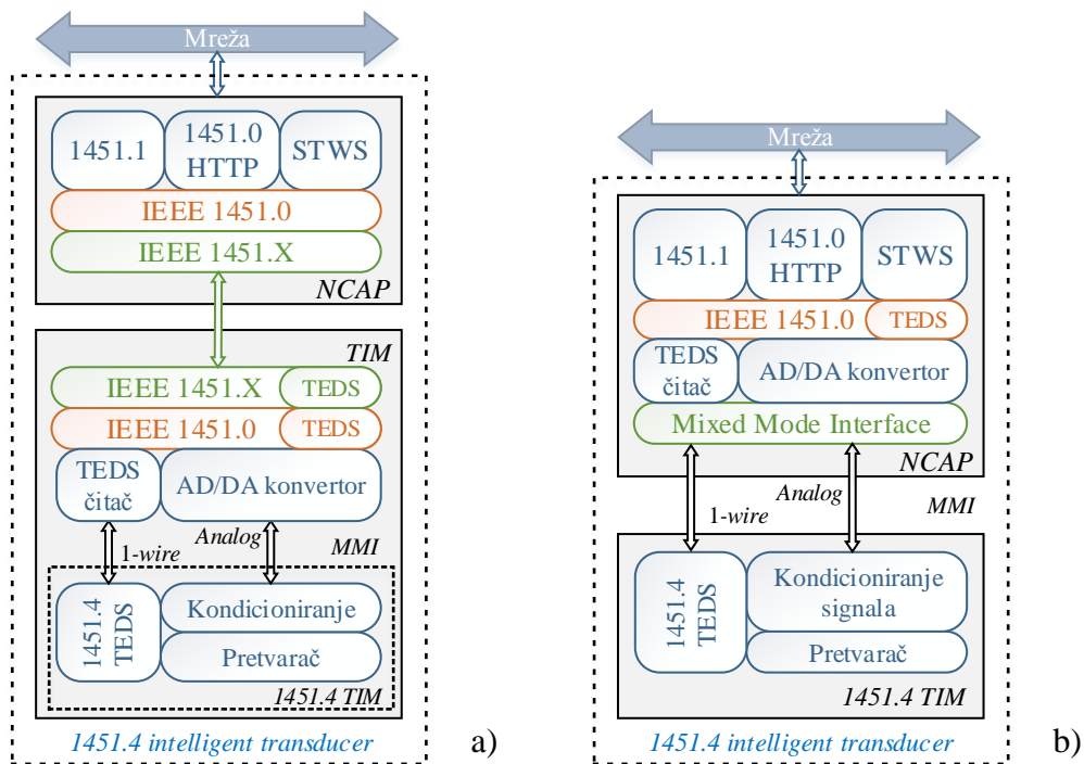
Slika 5.7. Model mrežnog povezivanja 1451.4 pretvarača: prema standardu 1451.0 (a) i prema predlogu iz [15] (b)
