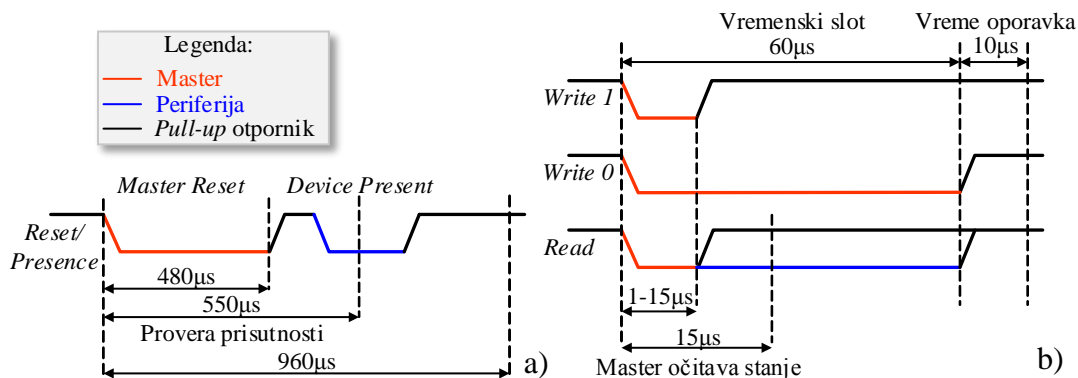
Slika 4.10. Vremenski dijagram osnovnih signala na jednožičnoj magistrali
