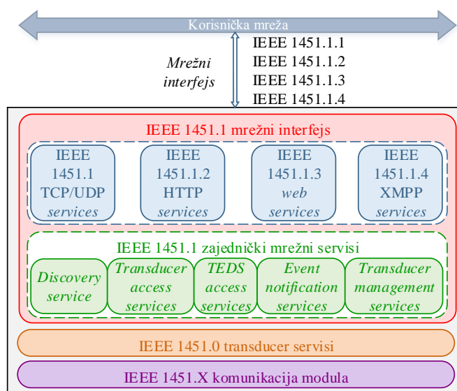
Slika 4.5. Mrežni interfejs prema modifikovanom IEEE 1451.1 standardu [20]
