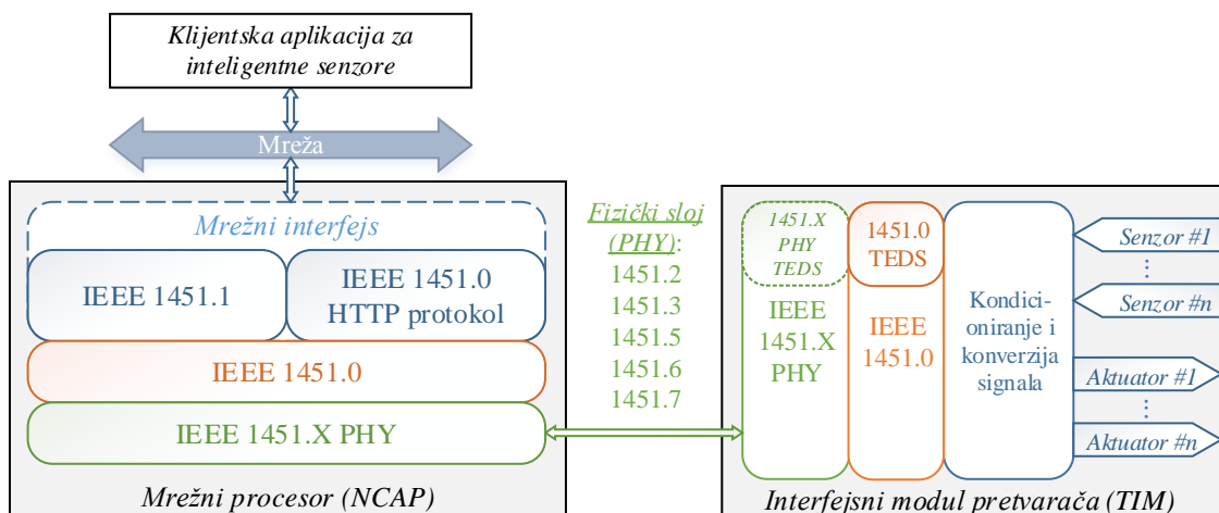
Slika 3.8. Model mrežnog povezivanja pretvarača prema IEEE 1451 standardu
