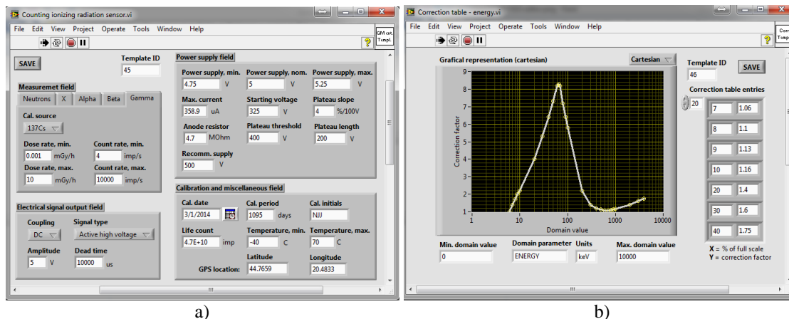
Slika 5.17. Grafički interfejs za unos parametara GM detektora prema šablonu: Counting ionizing radiation sensor (a) i Correction table (b)
