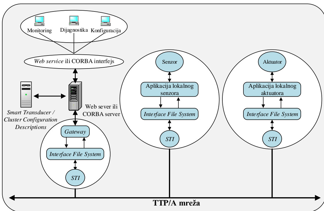
Slika 3.11. Arhitektura za konfiguraciju i menadžment sistema zasnovanog na TTP/A Fieldbus protokolu [84]
