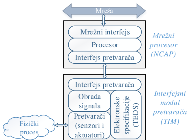
Slika 3.6. Model inteligentnog mrežnog pretvarača prema IEEE 1451 standardu
