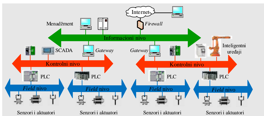
Slika 3.3. Arhitektura industrijske komunikacione mreže
