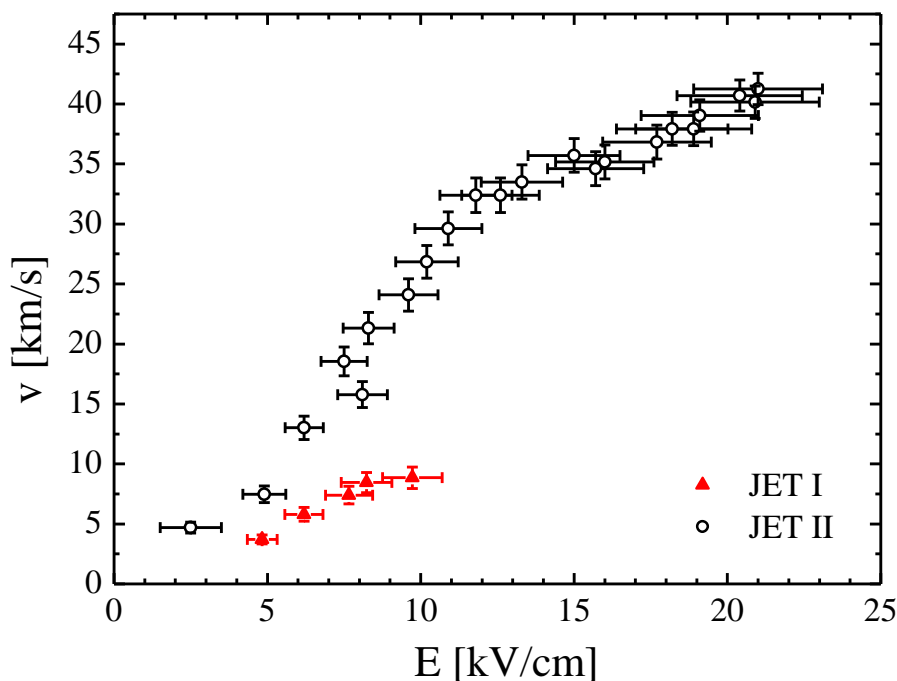
Слика 3.33: Зависност брзине плазменог метка, односно стримера у хелијуму од јачине електричног поља за оба плазмена млаза [264].
