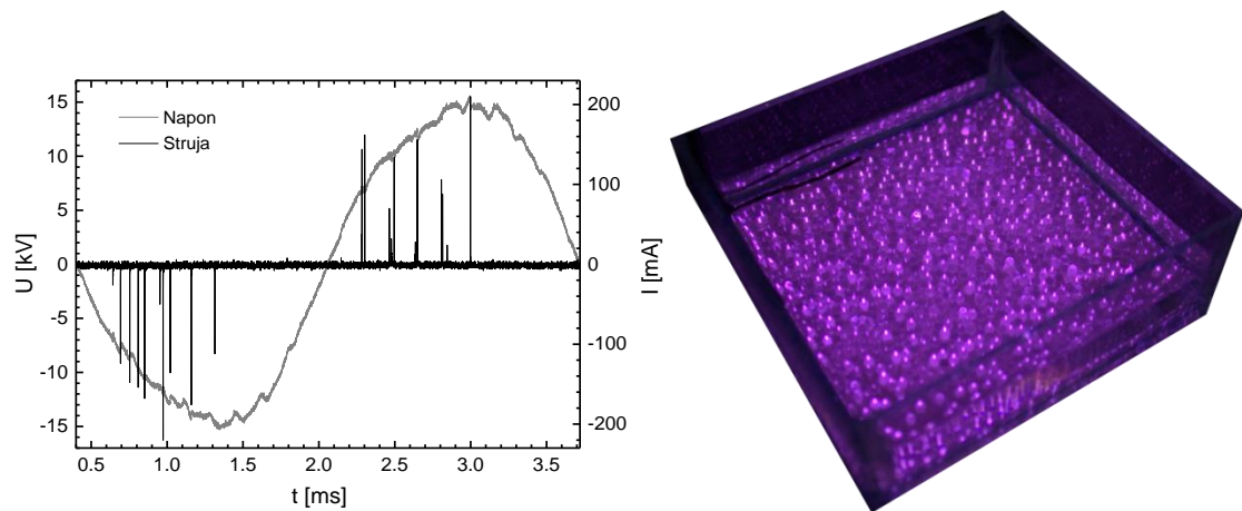
Слика 1.7: Струјни и напонски сигнали филаментарног пражњења и поглед на овакво пражњење кроз транспарентну электроду (Снимљено у Лабораторији за Физику и технологију плазме на Физичком факултету).
