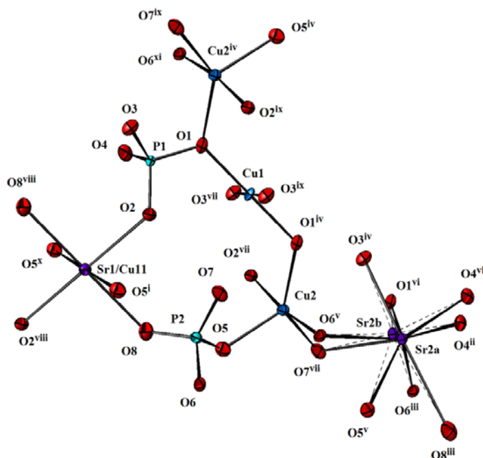
Slika 42. Deo strukture \text{SrCuP} sa šemom obeležavanja atoma. Termalni elipsoidi nacrtani su sa verovatnoćom od 50 %. Veze \text{Sr2b}-\text{O} predstavljene su tačkastim linijama. Simetrijski kodovi: (i) x, y+1, z ; (ii) x-1/2, -y-1/2, z-1/2 ; (iii) -x+1/2, y-3/2, -z-1/2 ; (iv) -x, -y, -z ; (v) -x+1/2, y-1/2, -z-1/2 ; (vi) -x, -y-1, -z ; (vii) x, y-1, z ; (viii) -x+1, -y+1, -z ; (ix) -x, -y+1, -z ; (x) -x+1, -y, -z ; (xi) x-1/2, -y+1/2, z+1/2 .
