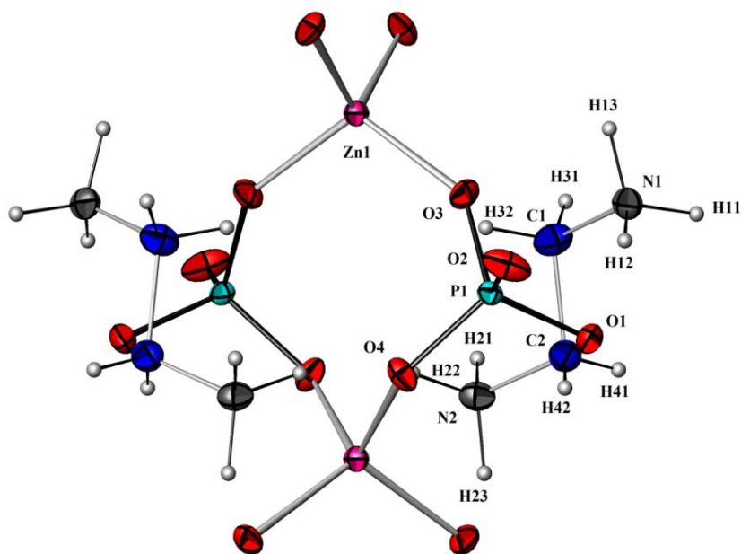
Slika 30. Projekcija u ac -ravni 4 M prstena i katjona \text{H}_2\text{en}^{2+} sa oznakama atoma u strukturi \text{ZnP}_2\text{O}_8 . Tetraedri \text{ZnO}_4 i \text{PO}_4 formiraju \text{ZnP}_2\text{O}_8^{4-} -lanac koji se pruža duž pravca [001] ( a -osa je horizontalna). Termalni elipsoidi nacrtani su sa verovatnoćom od 50 %, a sfere H atoma proizvoljnog su radijusa.
