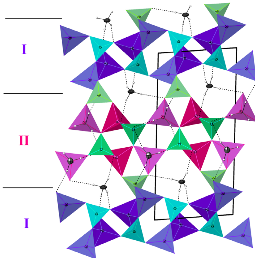
Slika 35. Projekcija strukture Zn_4P_3 duž [100] ( c -osa je vertikalna) koja prikazuje ZnO_4 , PO_4 i ZnO_3(NH_3) u pseudosloju I (ljubičast je ZnO_4 , a tirkizni PO_4 ) i u pseudosloju II (ružičasti su ZnO_4 i ZnO_3(NH_3) , a zeleni PO_4 ). U kanalima su smešteni NH_4^+ -joni. Sfere za N_2 i H proizvoljnog su radijusa. Isprekidane linije predstavljaju vodonične veze.
