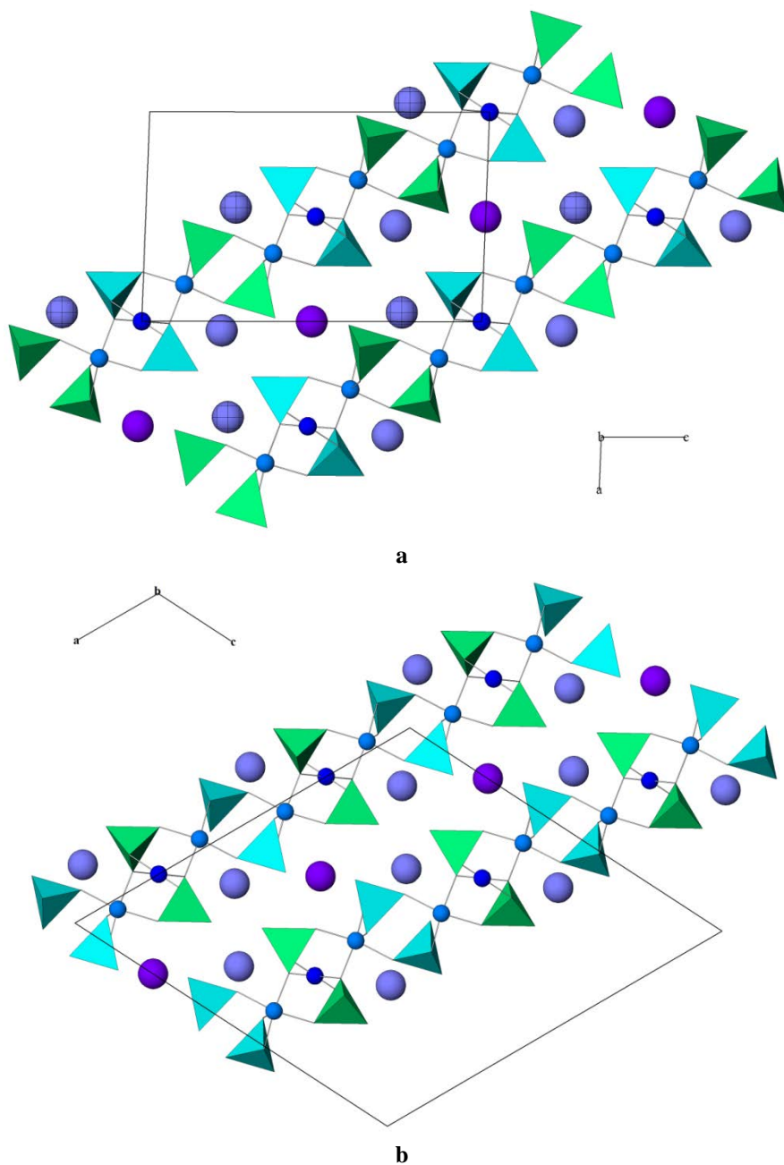
Slika 43. Redosled slaganja slojeva u: a) SrCuP i b) neizotipskom \text{Sr}_3\text{Cu}_3(\text{PO}_4)_4 (Effenberger, 1999) prikazano duž b -ose. Ljubičaste sfere predstavljaju atome stroncijuma: tamne Sr1/Cu11 i Sr1, a svetle Sr2 (šrafirane predstavljaju Sr2b položaj), tamno plave sfere predstavljaju Cu1, a svetlo plave Cu2 atome, koordinacioni tetraedri \text{P1O}_4 su tirkizni, a \text{P2O}_4 su zeleni.
