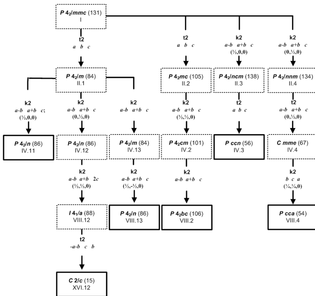
Slika 22. Bernighausenovo stablo prikazuje odnose supergrupa/subgrupa među jedinjenjima DFT-tipa. Prostorne grupe date u zacrtnjenim okvirima odgovaraju stvarnim kristalnim strukturama, dok prostorne grupe date u tačkastim okvirima odgovaraju međukoracima potrebnim za izvođenje subgrupa. Pomeranje ishodišta dato je u koordinatnom sistemu prostorne grupe više simetrije.
