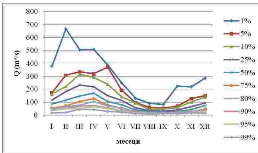
Сл.70 - Унутаргодишња расподела протицаја Јужне Мораве у Мојсињу на основу месечних квантила
