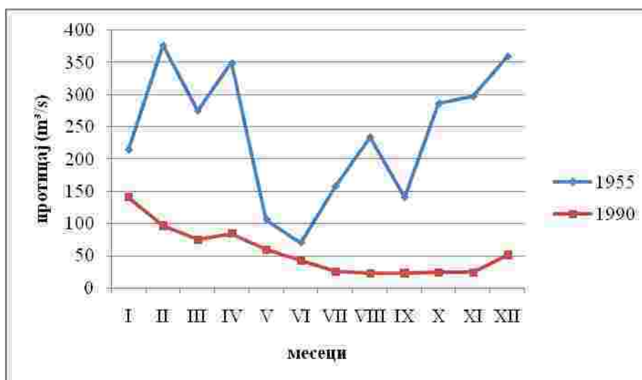
Сл. 76 - Средњи месечни протицаји Западне Мораве код Јасике једне веома водне и веома сушне године
