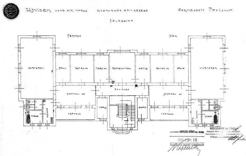
Сл. 102: Ђерђ Копечек, Велика градска болница у Новом Саду 1912. Основа приземља Клинике за хирургију. Извор: ТАСГ 6/ПК
