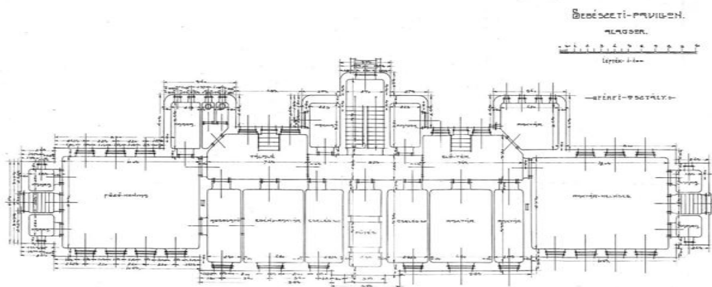
Сл. 101: Ђерђ Копечек, Велика градска болница у Новом Саду 1912. Основа сутерена Клинике за хирургију. Извор: ТАСГ 6/ПК
