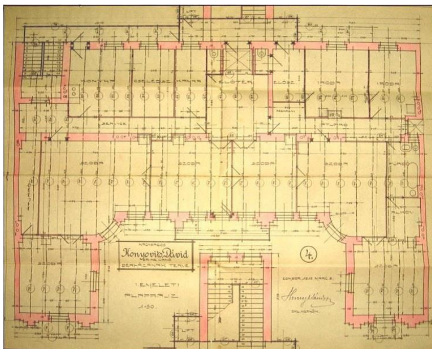
Сл. 150: ШандорХерцог, Коњовићева палата, основа спрата 1912.Извор: Историјски архив Сомбор, бр. 1041; Б. Јањушевић, Нав. дело , 170.
