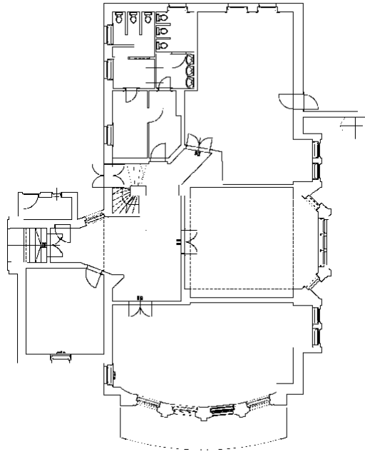
Сл. 179: Вила Линденић у Бачкој Паланци, почетак 20. века. Основа приземља. Извор: Покрајински завод за заштиту споменика културе, фотодокументација; Б. Јањушевић, Настанак и развој стамбених палата... , 197.
