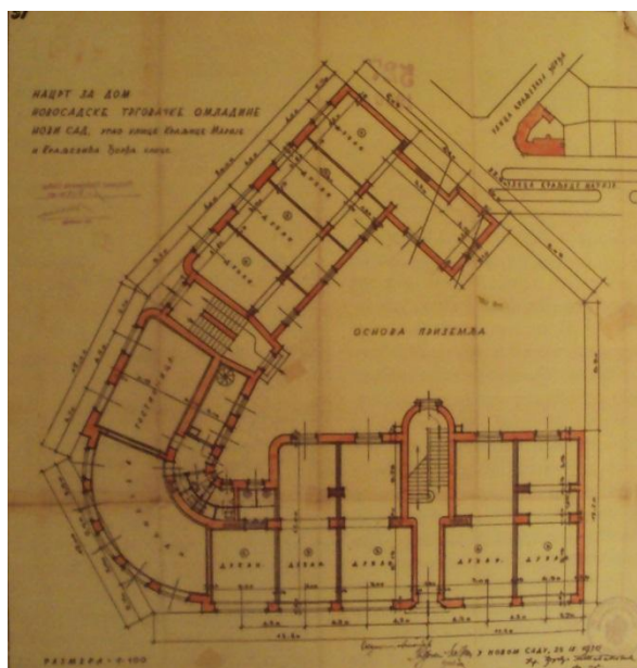
Сл. 485 и 486: Ђорђе Табаковић, Зграда Дома новосадске трговачке омладине, 1932. Извори: аутор рада и ТАСГ, 119, 527/1930.
