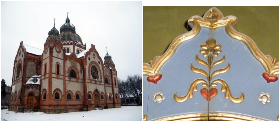
Сл. 41 и 42: Марсел Комор и Деже Јакоб, Синагога у Суботици, 1902. Извор:
