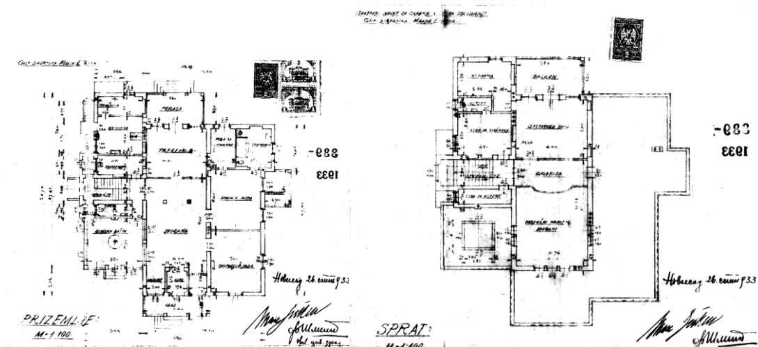
Сл. 761-765: Филип Шмит, Вила Ајкен у Новом Саду, 1933. Извор: аутор рада
