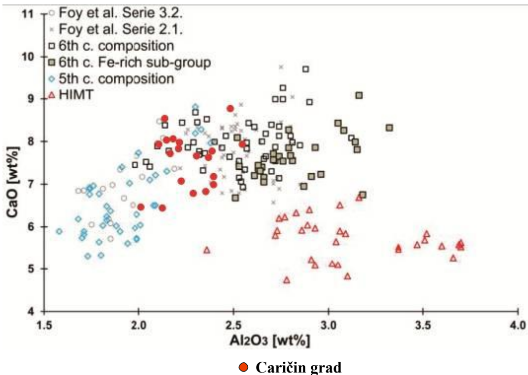
Grafikon 35. Poređenje odnosa \text{CaO}/\text{Al}_2\text{O}_3 u uzorcima sa Caričinog grada sa poznatim grupama stakla (5-6. vek) i HIMT staklom (podloga preuzeta iz: Cholakova et al. in press, Fig. 4)
