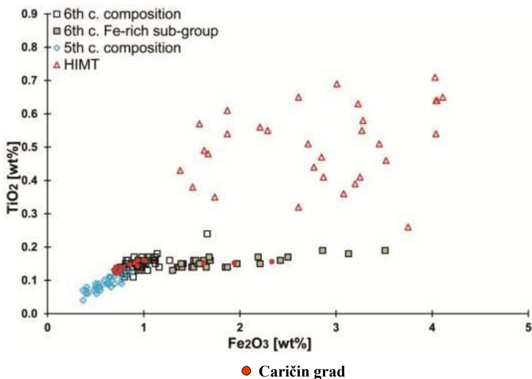
Grafikon 36. Poređenje odnosa \text{TiO}_2/\text{Fe}_2\text{O}_3 u uzorcima sa Caričinog grada sa poznatim grupama stakla (5-6. vek) i HIMT staklom (podloga preuzeta iz: Cholakova et al. in press, Fig. 6)
