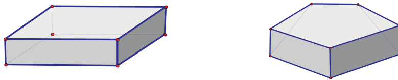
Слика 3.17: Комбинаторно различити политопа са истим f -векторима
