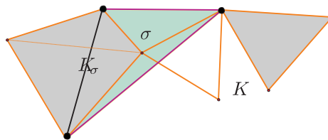
Слика 2.21: Пуни подкомплекс
