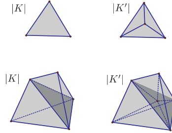
Слика 2.11: Подподеле симплицијалних комплекса
