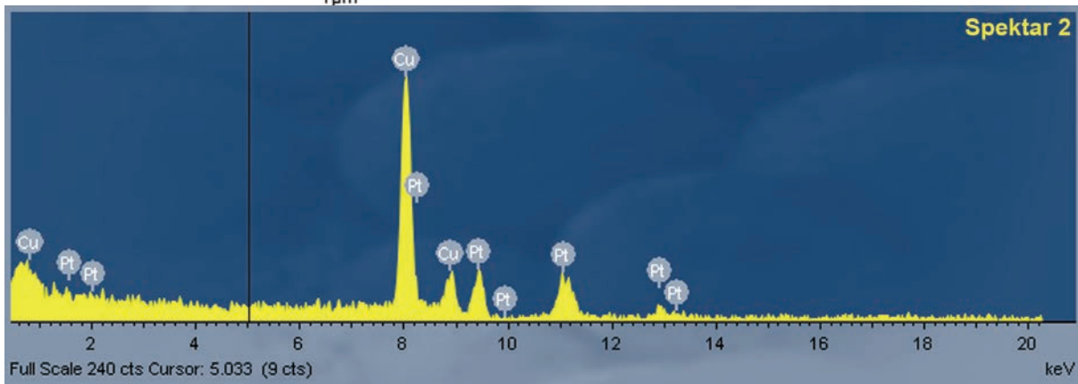
Slika D3. EDS spektar Pt/e-MWCNT.
