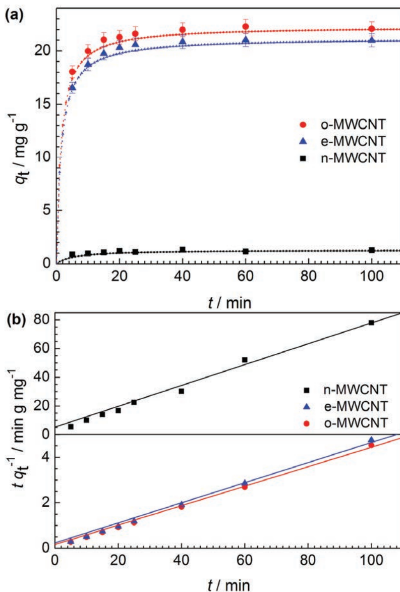
Slika 4.4. (a) Uticaj vremena na sorpcije Cd 2+ jona na n-MWCNT, o-MWCNT i e-MWCNT ( C[\text{Cd}^{2+}]_0 = 5 \text{ mg/l} , m/V = 100 \text{ mg/l} , pH 8, T = 25 \text{ }^\circ\text{C} . Linije: Kinetički model pseudo-drugog reda. (b) Linearizovani kinetički model pseudo-drugog reda za sorpcije Cd 2+ na n-MWCNT, o-MWCNT i e-MWCNT. ( C[\text{Cd}^{2+}]_0 = 5 \text{ mg/l} , m/V = 100 \text{ mg/l} , pH 8, T = 25 \text{ }^\circ\text{C} ).
