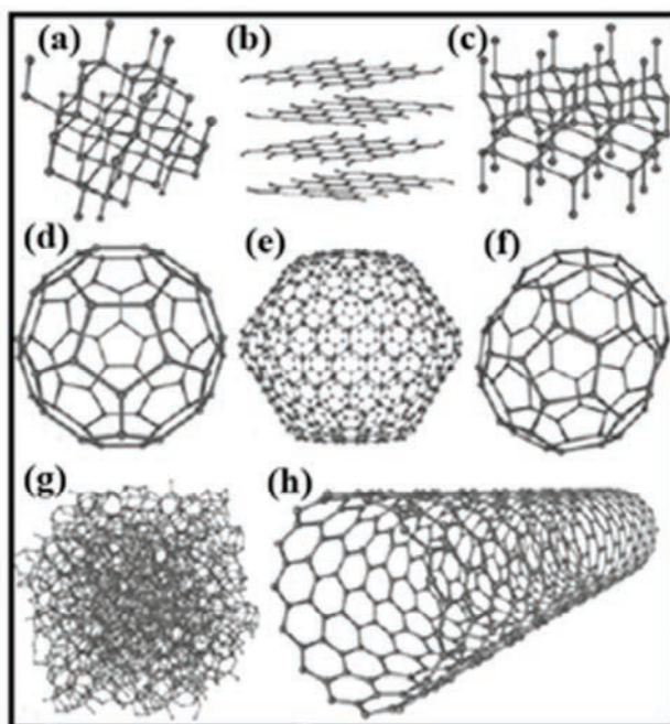
Slika 2.1. Alotropske modifikacije ugljenika: (a) dijamant, (b) grafit, (c) lonsdaleit, (d) C_{60} , (e) C_{540} , (f) C_{70} , (g) amorfni ugljenik i (h) ugljenična nanocev.
