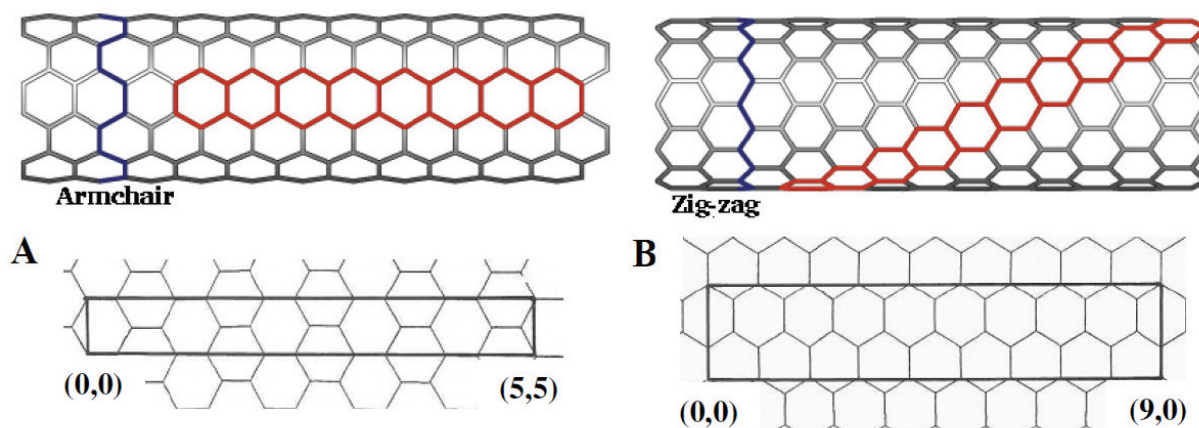
Slika 2.9. Jedinična ćelija (a) (5,5) „armchair“ nanocevi i (b) (9,0) „zig-zag“ nanocevi.
