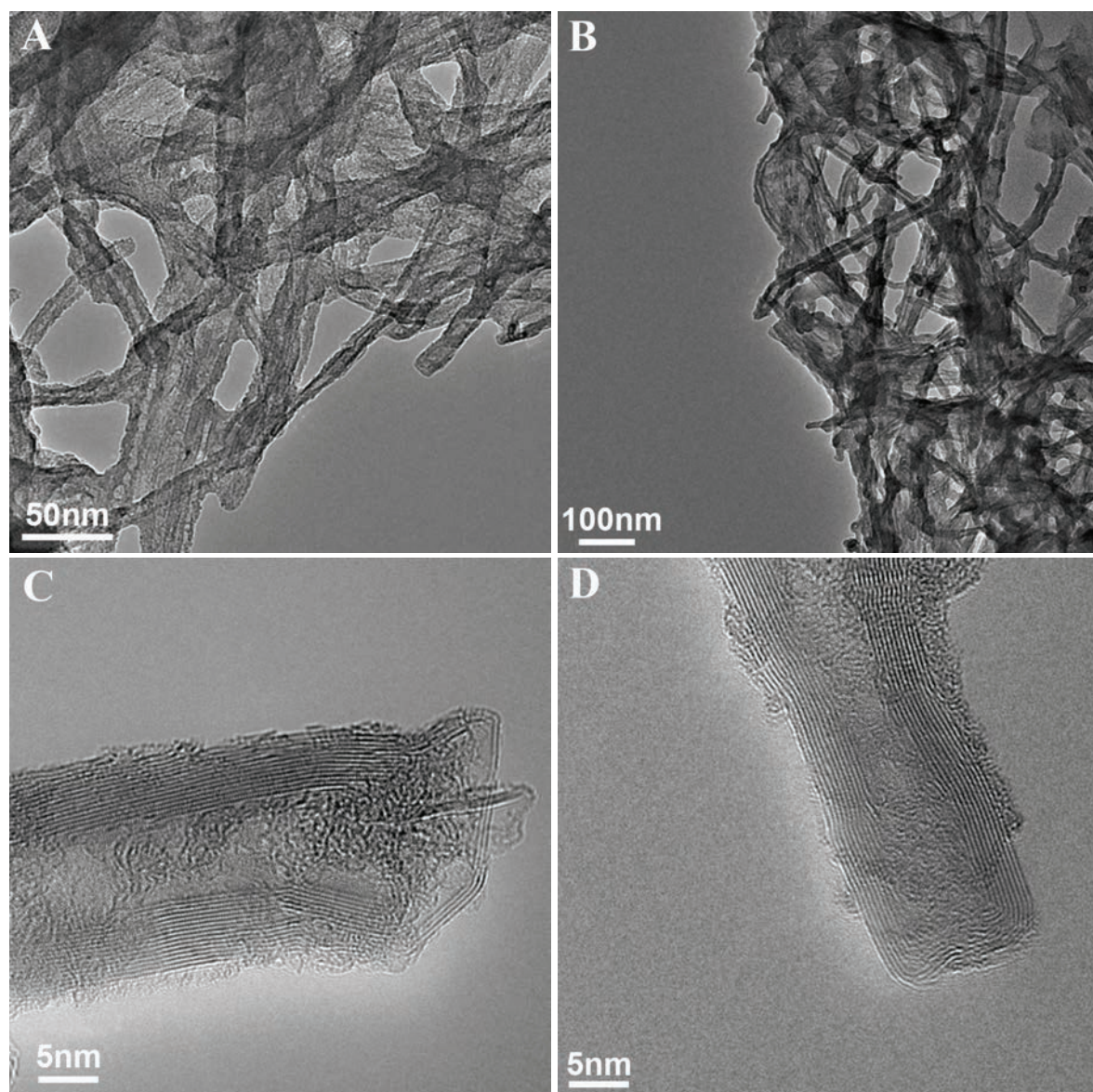
Slika B1. TEM slike e-MWCNT nakon adsorpcije Cd 2+ jona.
