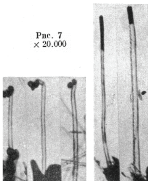
Slika 2.3. Primeri TEM slika ugljeničnih nanocevi koje su objavljene 1952 [10].
