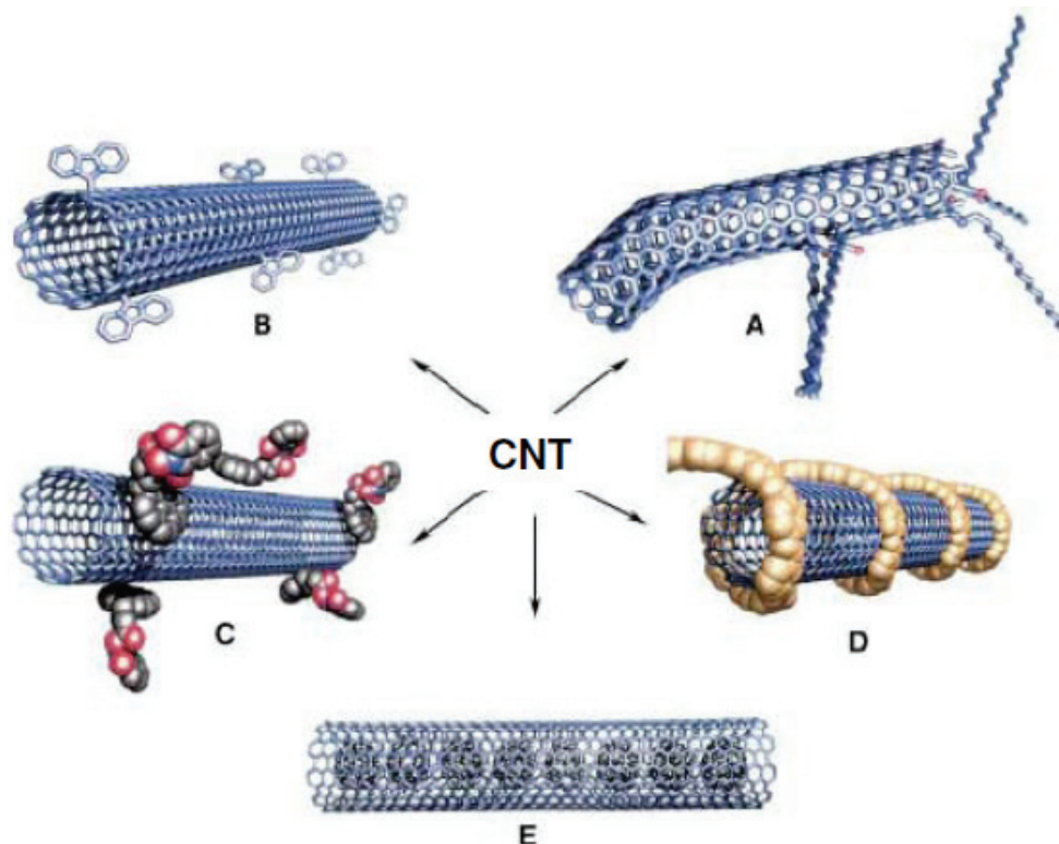
Slika 2.19. Mogućnosti funkcionalizacije CNT: (a) funkcionalizacija preko defektnih mesta, (b) kovalentna funkcionalizacija bočne strane, (c) nekovalentna funkcionalizacija surfaktantima, (d) nekovalentna egzohedralna funkcionalizacija sa polimerima, i (e) endohedralna funkcionalizacija [50].
