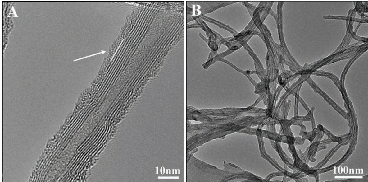
Slika 7.4. Reprezentativne TEM slike dap-MWCNT.
