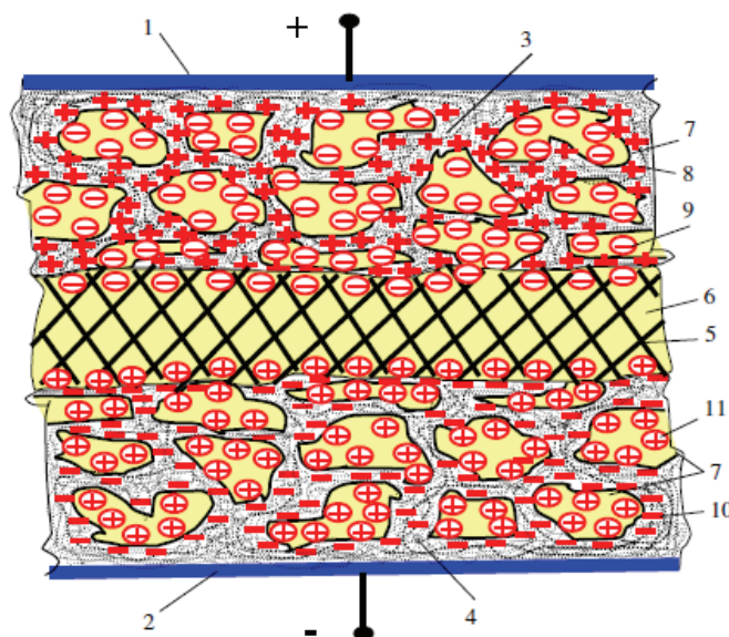
Slika 2.33. Šematski prikaz naelektrisanog superkondenzatora: 1 i 2 - strujni kolektori; 3 i 4 - elektrode; 5 - separator; 6 - elektrolit; 7 - pore u materijalu elektrode; 8 - pozitivno naelektrisanje; 9 - negativni jon; 10 - negativno naelektrisanje (elektroni); 11 - pozitivni jon [271].
