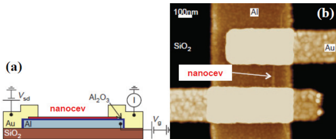
Slika 2.35. (a) Šematski prikaz CNT-FET-a. Poluprovodljiva nanocev koja je na vrhu izolacionog sloja aluminijum-oksida spojena je na oba kraja za elektrode zlata. Struja se kroz nanocev propušta primenom potencijala na aluminijumskom prekidačkom kolu, koje se nalazi ispod nanocevi i sloja aluminijum-oksida. V_{sd} je električni napon izvora, a V_g je napon prekidačkog kola. (b) STM slika SWCNT-FET-a prikazanog pod (a). Aluminijumski sloj je obložen aluminijum oksidom [284].
