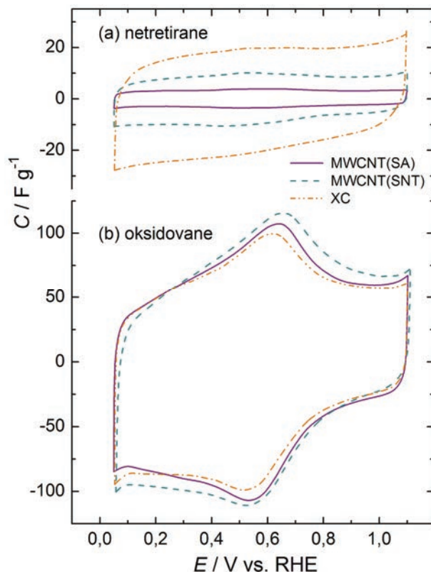
Slika 6.7. Kapacitivne potenciodinamičke krive (a) netretiranih i (b) oksidovanih MWCNT i XC snimljenih u 0,10 M \text{H}_2\text{SO}_4 pri 100 mV/s u atmosferi azota. Oksidacija je izvršena u smeši \text{H}_2\text{SO}_4 i \text{HNO}_3 (3:1).
