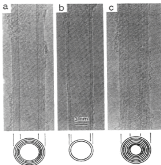
Slika 2.11. Višeslojne ugljenične nanocevi, prvi put snimljene pomoću TEM-a [5].
