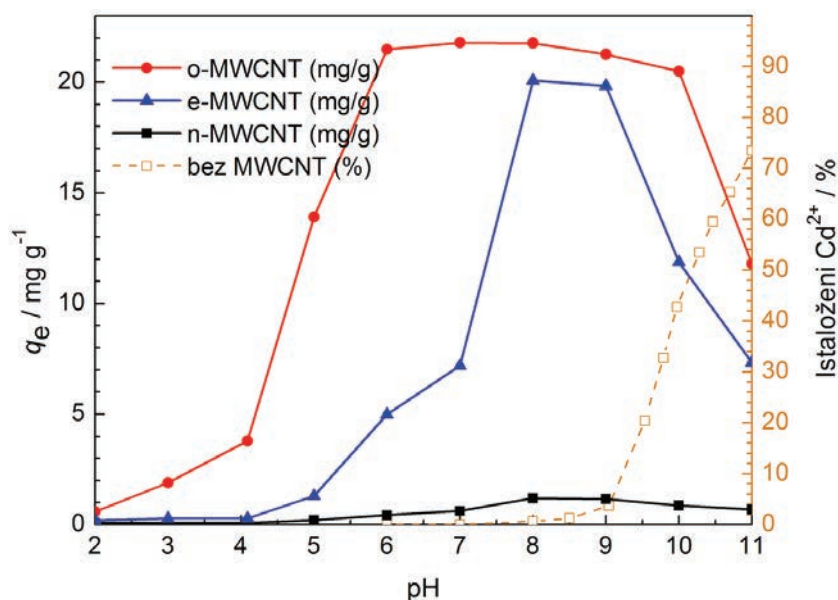
Slika 4.3. Uticaj pH vrednosti na adsorpciju \text{Cd}^{2+} jona na n-MWCNT, o-MWCNT i e-MWCNT (u mg/g). C[\text{Cd}^{2+}]_0 = 5 mg/l, m/V = 100 mg/l, T = 25 °C. Uticaj pH vrednosti na taloženje \text{Cd}^{2+} (u (%) u odnosu na ukupnu količinu \text{Cd}^{2+} ). C[\text{Cd}^{2+}]_0 = 5 mg/l, T = 25 °C.
