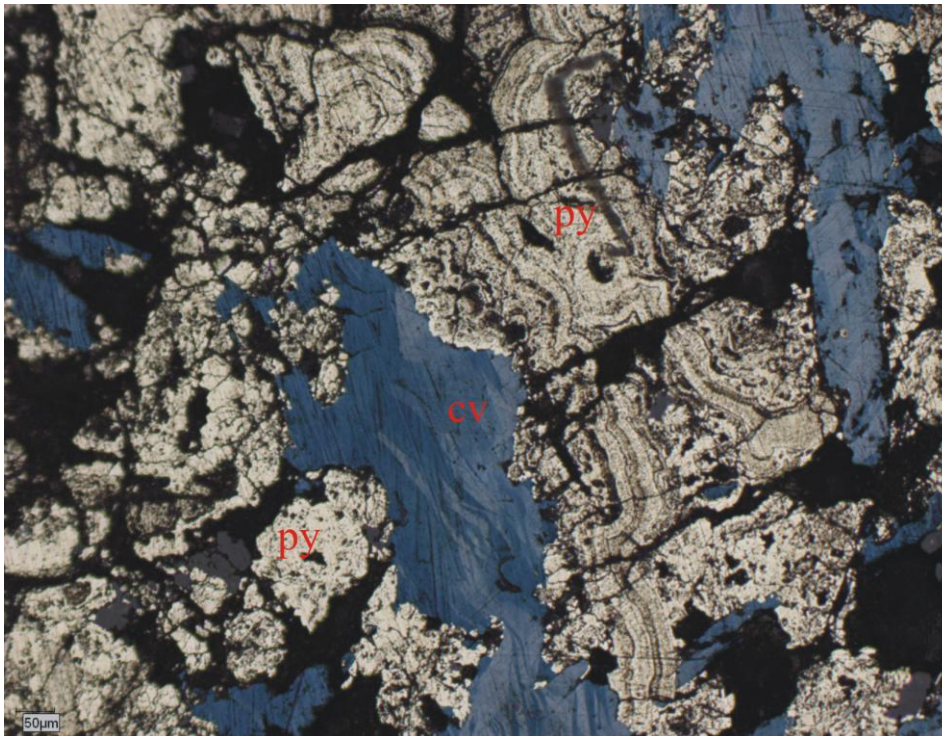
Слика 38a-3: Ковелин (cv) у средини жице са колоформним пиритом (py) око њега, одбијена светлост.
