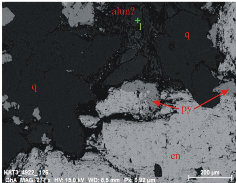
Слика ср051-5: Py-en жица са енаргитом (en), пиритом (py) и алунитом (alun) запуњава пукотине између зрна раног кварца (q), BSE слика направљена на SEM уређају.
