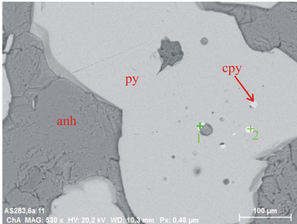
Слика ср119-1: Пирит са уклопљеним зрнима халкопирита (cру), борнита и халкозина у анхидритској жици (anh), BSE слика направљена на SEM уређају.
