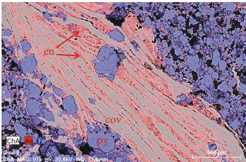
Слика ср012-5: Комбинована мапа елемената за арсен (As-црвено) и гвожђе (Fe- плаво), на којој се уочава жица са тракама ковелина (cov) и снаргита (en) која пролази кроз зрна раног пирита (пу), слика направљена на електронском микроскопу (SEM).
