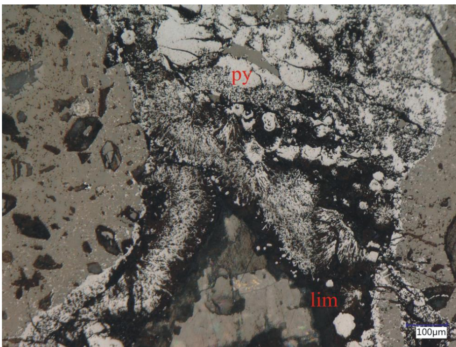
Слика ср061-6: Колоформни пирит (py) и лимонит (lim) у пукотинама у алтерисаном андезиту, одбијена светлост.
