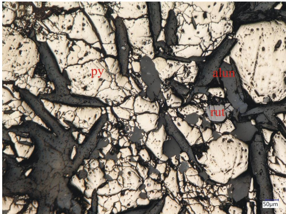
Слика ср127-2: Дугуљасти кристали алуниита (alun) у пукотинама око зрна пирита (py) и рутила (rut), одбијена светлост.
