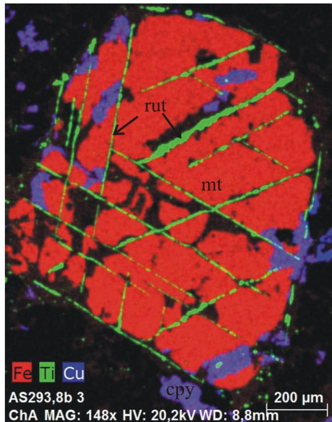
Слика ср084-5т: Комбинована мапа елемената, гвожђе (Fe-црвено), титанијум (Ti- зелено) и бакар (Cu- плаво), на којој се виде издвајања рутила (rut) у зрну магнетита (mt) са халкопиритом (сру) по ободу, мапа елемената направљена на SEM уређају.
