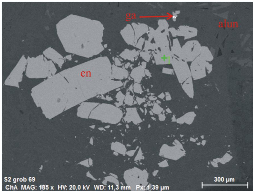
Слика ср063-3: Енарцит (en) са повећаном концентрацијом германијума и малим зрнима галенита (ga) у кварцно-алунитској (alun) жици, BSE слика направљена на SEM уређају.
