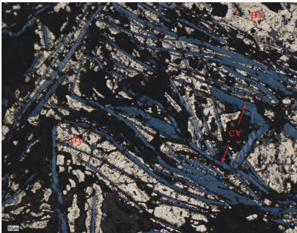
Слика 38a-4: Py-cov жице са ковелином (cv) у средини и пиритом (py) око ковелина, одбијена светлост.
