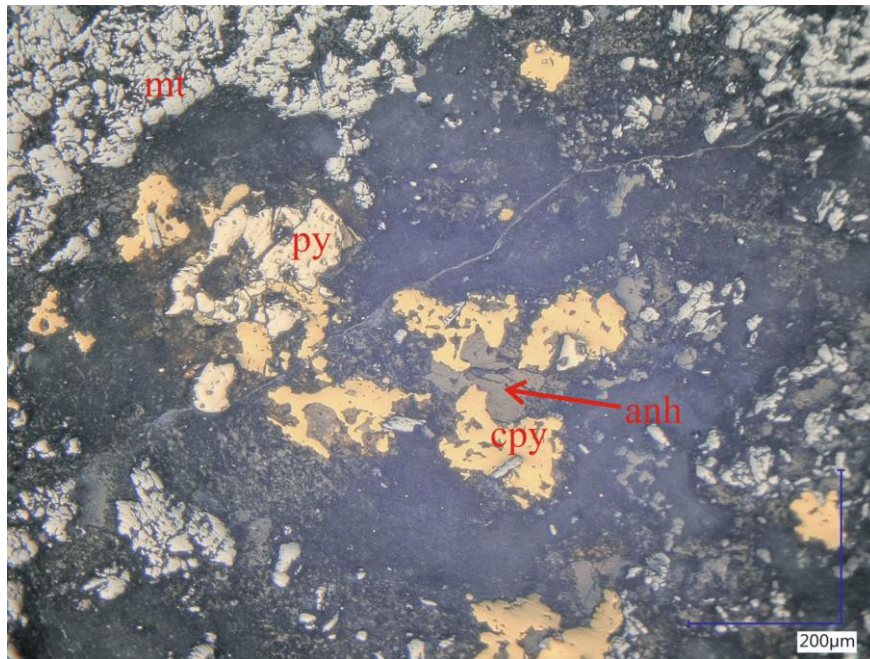
Слика ср137-1: Пирит (py) и халкопирит (sph) у алтерисаној стени поред магнетитске жице (mt), анхидрит (anh) запуњава пукотине око осталих минерала, одбијена светлост.
