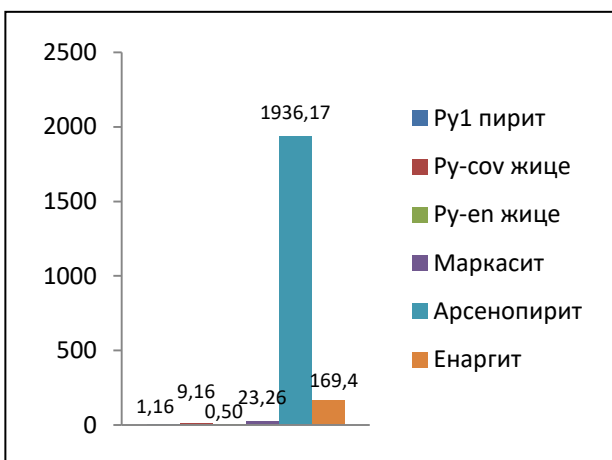
Слика 37: Просечне концентрације антимаона (ppm) у различитим сулфидним минералима.
