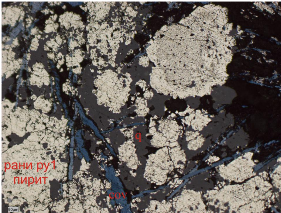
Слика 38a-1: Танке ковелинске жице (cov) пролазе кроз кварц (q) који садржи зрна раног пирита (py1), одбијена светлост.
