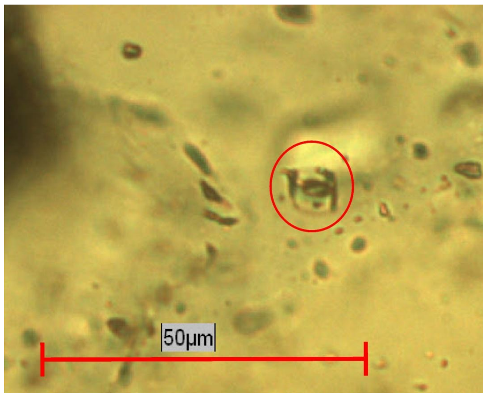
Слика 123-8: Инклузија са кристалима соли и неправидним (сулфидним) кристалом (тип 3) у кварцу, пропуштена светлост.
