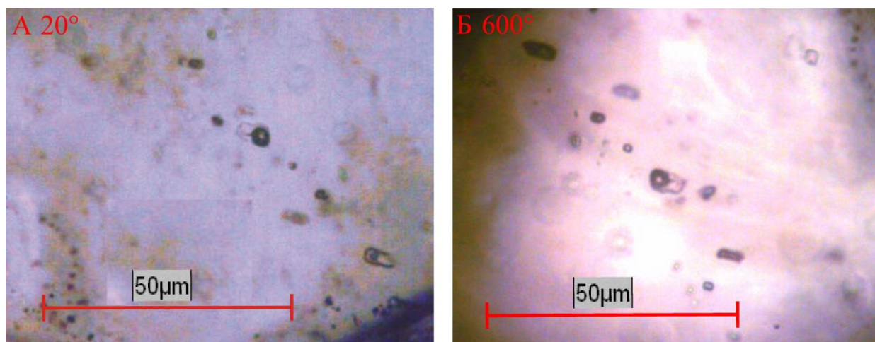
Слика 22: Фотографије инклузија типа 1 из узорка CP141
