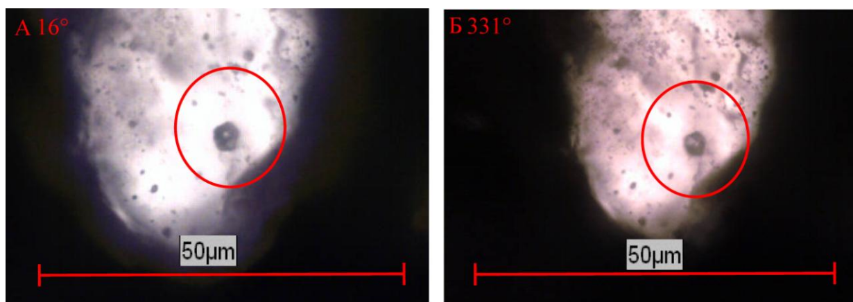
Слика 26: Фотомикрографије хомогенизације инклузије типа 4 из узорка CP096.
