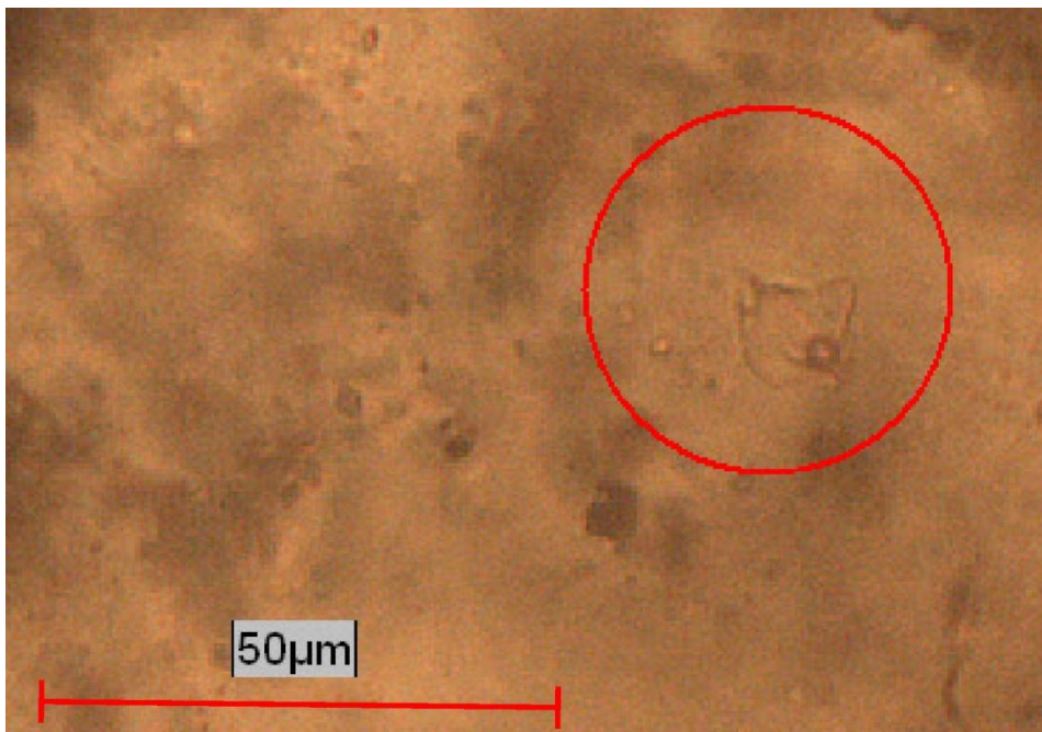
Слика 116-8: Нискотемпературна инклузија богата течносту (тип 7) са непровидним минералом у кварцу, пропуштена светлост.
