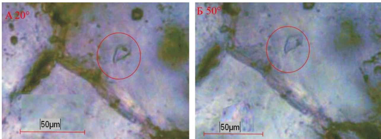
Слика 29: Фотографије хомогенизације инклузије типа 7 из узорка СР141. А) Инклузија на собној температури са течном и гасном фазом (мехуром). Б) Инклузија на температури од 50°C на којој је мехур потпуно смањен. Приказана инклузија је достигла тоталну хомогенизацију на 73°C.
