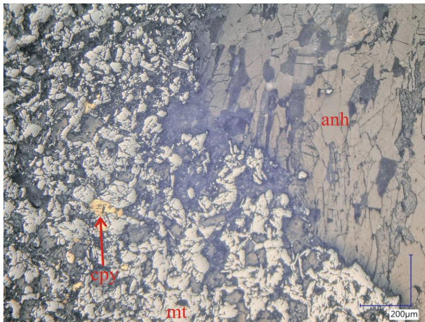
Слика ср137-3: Контактна зона магнетитске жице (mt) са халкопиритом (sph) и млађе анхидритске жице (anh), одбијена светлост.
