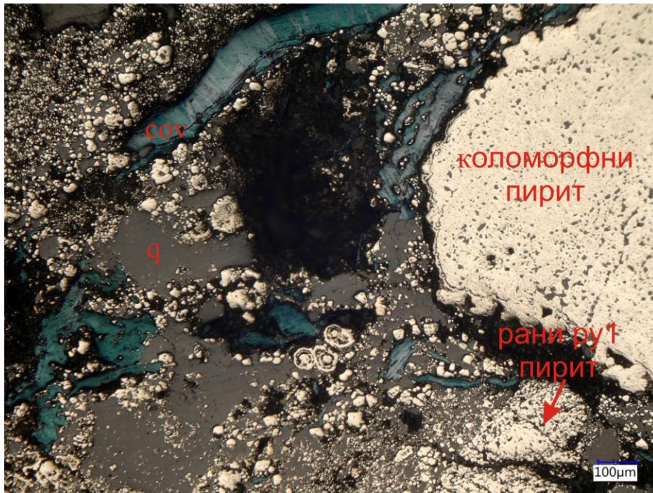
Слика ср012-4: Колоформни пирит (Pu) и ковелин (cov) око кварчне жице (q) са раним пиритом, одбијена светлост.
