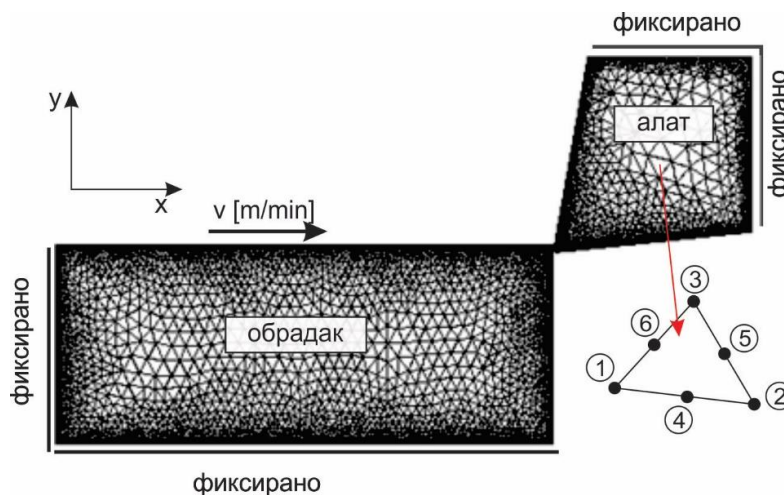
Слика 8.1. 2D модел са мрежом коначних елемената
