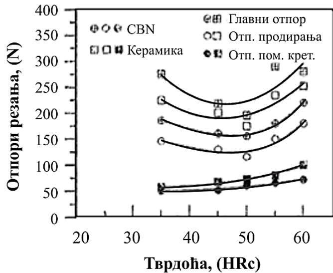
Слика 2.15. Промена компоненти отпора резања у функцији тврдоће материјала обраатка
