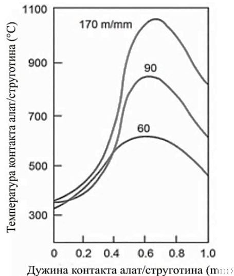
Слика 3.8. Расподела температуре на контактної површини алат/струготина
