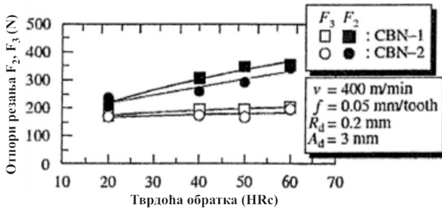
Слика 2.16. Промена компоненти отпора резања F_2 и F_3 у функцији тврдоће материјала обраатка
