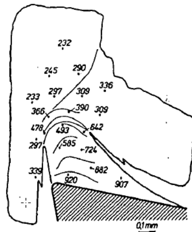
Слика 2.9. Тврдоћа сегмената насlage и предмета обраде, НВ [20]
