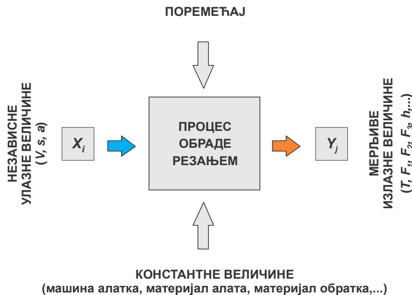
Слика 6.1. Шематски приказ процеса обраде резањем
