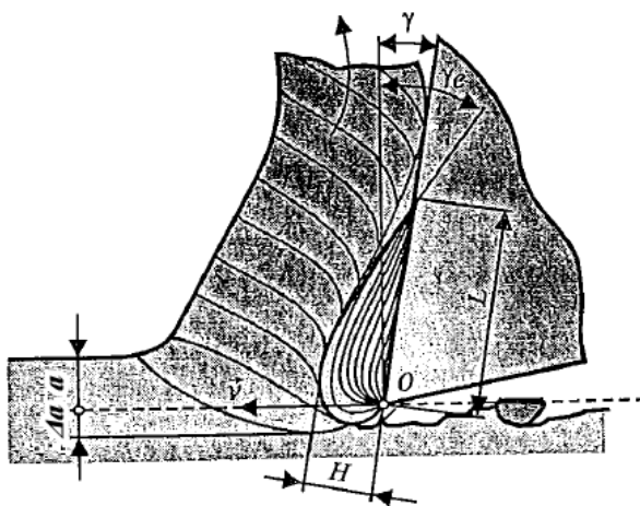
Слика 2.8. Промена геометрије на резном клину услед стварања насlage
