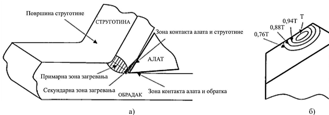
Слика 3.2. а) Зона загревања при машинској обради стругањем, б) Распоред температура на резном алату
