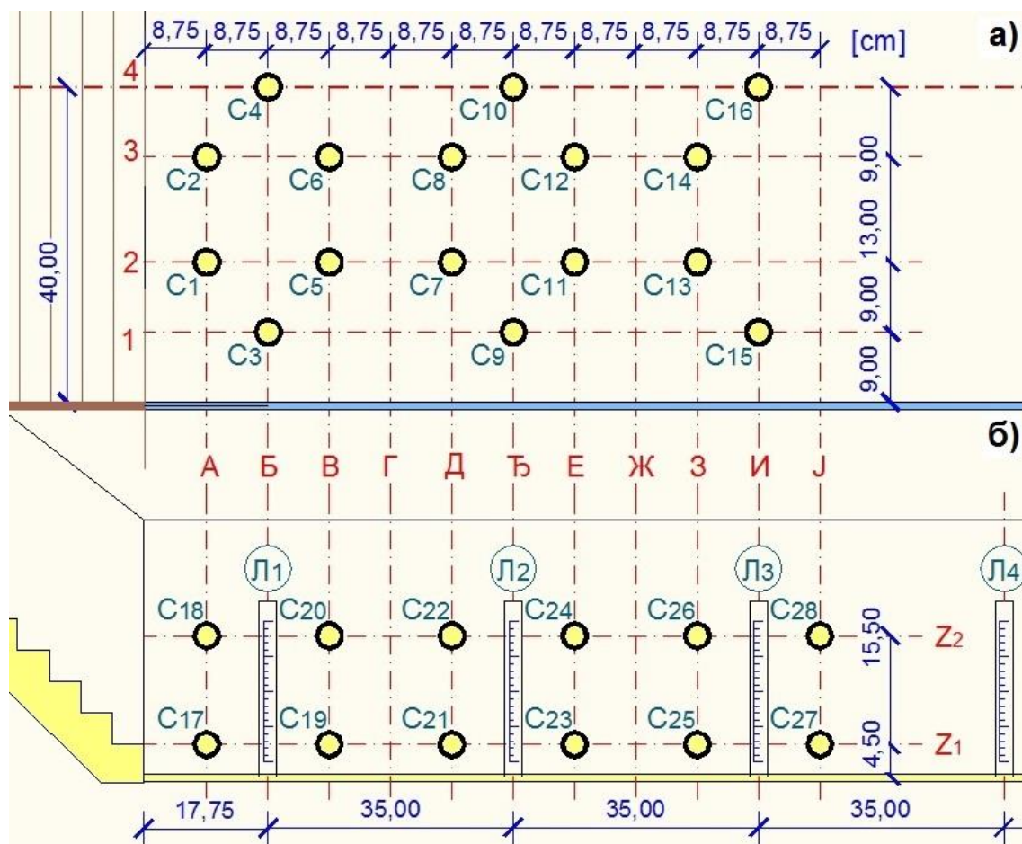
Слика 4.68 Распоред мерних сонди и лењира на моделу ГФ-1M
