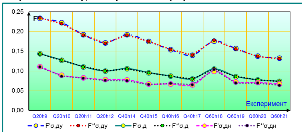
Слика 4.104 Слагање сила од пулзација ( F' ) добијених директном методом, са силама ( F^* ) добијеним под претпоставком о нормалној расподели на моделу ГФ-2М
