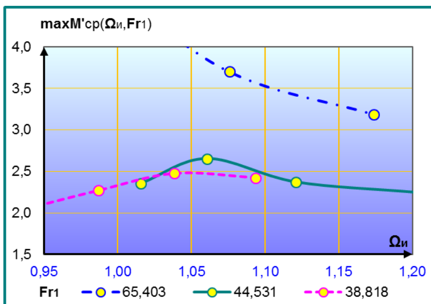
Слика 4.63 Промена максималног момента у уклештењу зида услед средњих притисака, у зависности од потопљености скока и Фрудовог броја на моделу ГФ-0V
