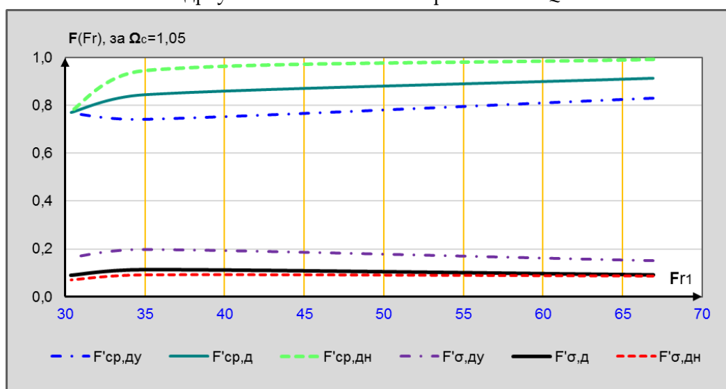
Слика 4.88 Промена утицаја у базену, при варијацији Фрудовога броја и истој потопљености хидрауличног скока у базену за модел ГФ-1V
