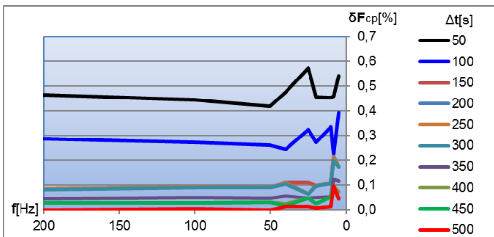
Слика 4.22 \delta F_{cp}(f) , са параметром \Delta t
