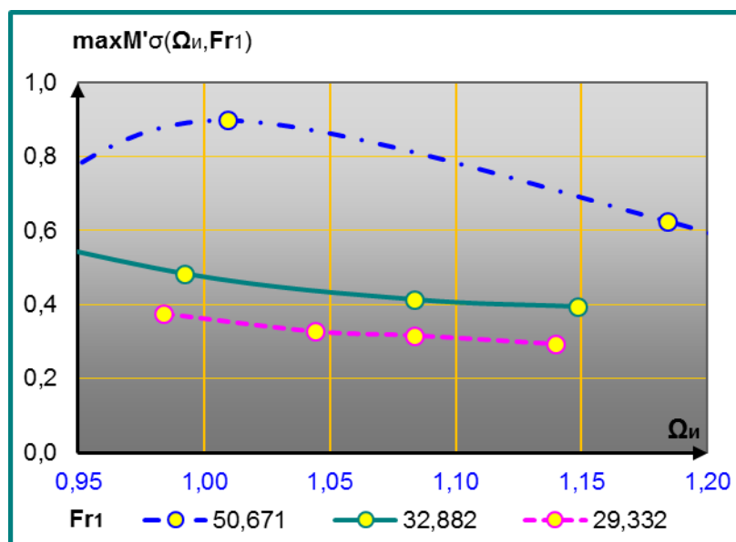
Слика 4.81 Промена максималног момента у уклештењу зида услед пулзација у зависности од потоппљености скока и Фрудовог броја на моделу ГФ-1М
