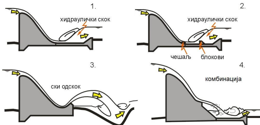
Слика 2.1 Најчешће диспозиције евакуационих органа, [12]
