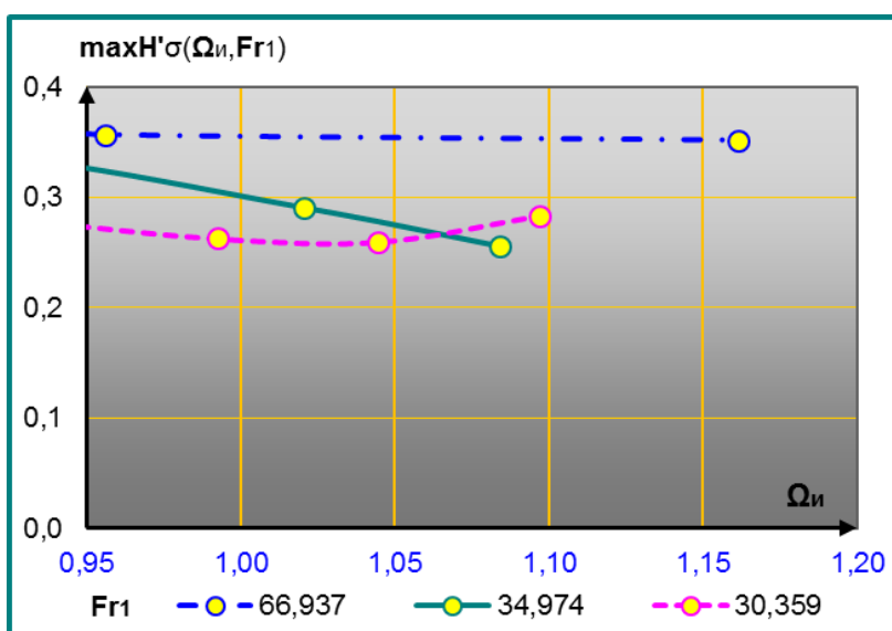
Слика 4.92 Промена максималне хоризонталне силе у уклештењу зида услед пулзација у зависности од потопљености скока и Фрудовог броја на моделу ГФ-1V
