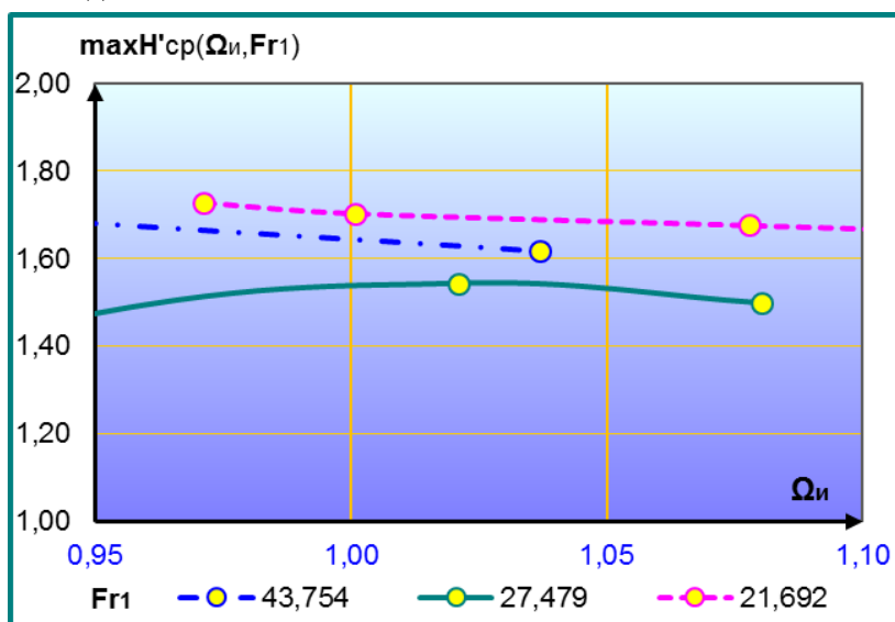
Слика 4.122 Промена максималне хоризонталне силе у уклештењу зида услед средњих притисака, у зависности од потоњености скока и Фрудовог броја на моделу ГФ-2V
