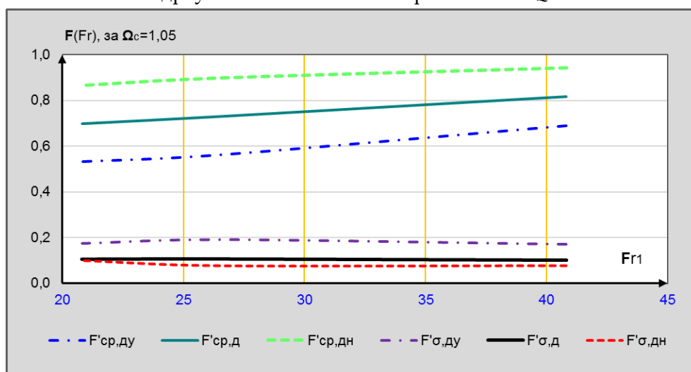
Слика 4.103 Промена утицаја у базену, при варијацији Фрудовог броја при истој потоњености хидрауличног скока у базену на моделу ГФ-2М
