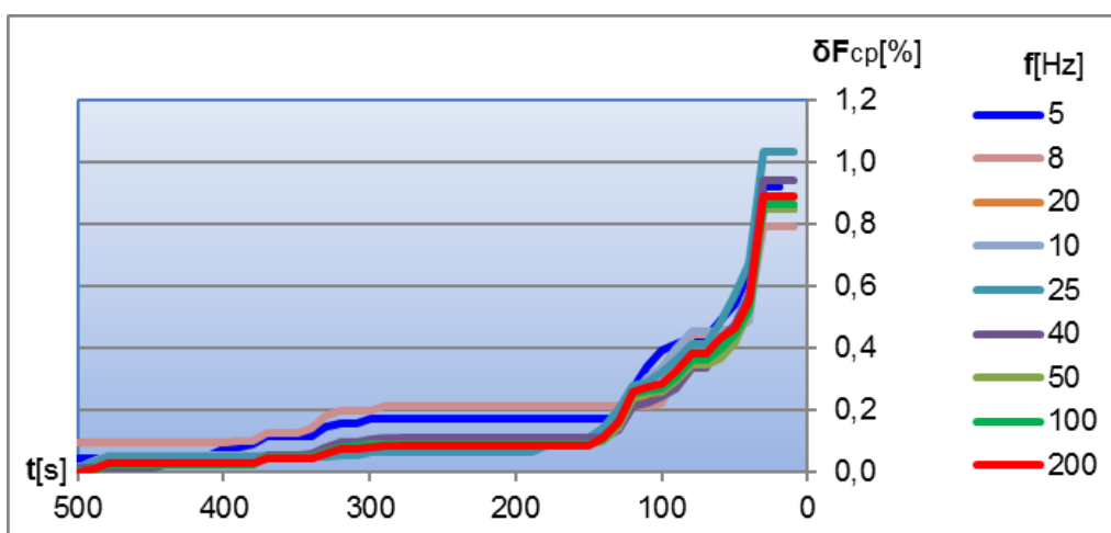
Слика 4.23 \delta F_{cp}(\Delta t) , са параметром f
