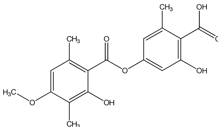
Сл. 86. Структурна формула супстанце obtusis acid
