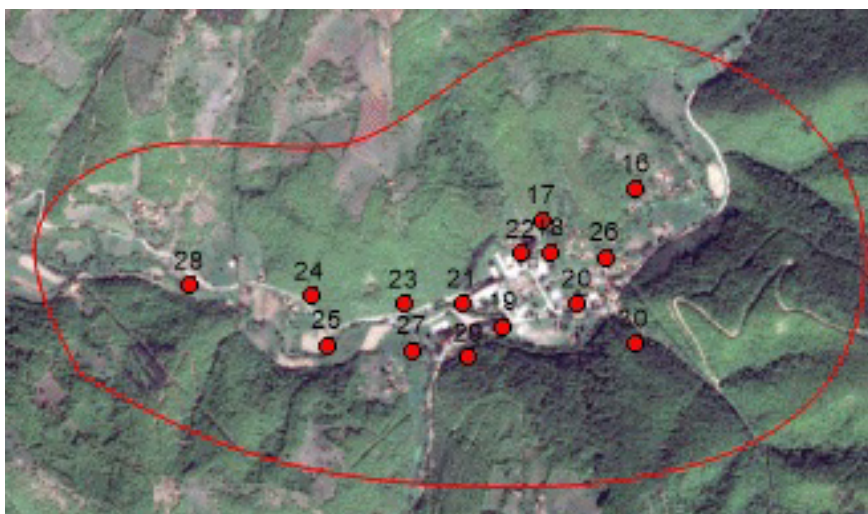
Сл. 10. Сателитски снимак истраживаног подручја Куршумлијске бање са обележеним истраживаним тачкама
