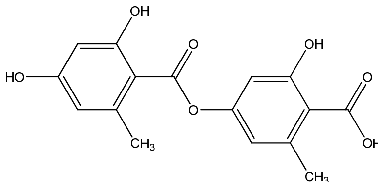
Сл. 89. Структурна формула супстанце lesanoric acid
