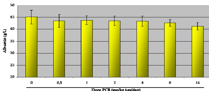
Slika 20. Uticaj različitih doza PCB na koncentraciju albumina u krvi Wistar pacova izloženih Cd tokom 28 dana. Vrednosti su predstavljene kao X_{sr} \pm SD (n=7). Vrednosti koje su označene različitim slovima se statistički značajno razlikuju (ANOVA, LSD test; P<0,05).
