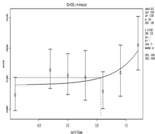
Slika 23. Analiza odnosa doza-odgovor za nivoe AST u serumu pacova tretiranih različitim dozama PCB. Podaci su fitovani korišćenjem PROAST softvera. Zadata veličina CES bila je 5% (A) odnosno 10% (B) (horizontalna tačkasta linija). Odgovarajuća doza (CED) predstavljena je vertikalnom tačkastom linijom. CEDL i CEDU predstavljaju donju i gornju granicu 95% intervala pouzdanosti. Doze PCB predstavljene su kao log 10 .
