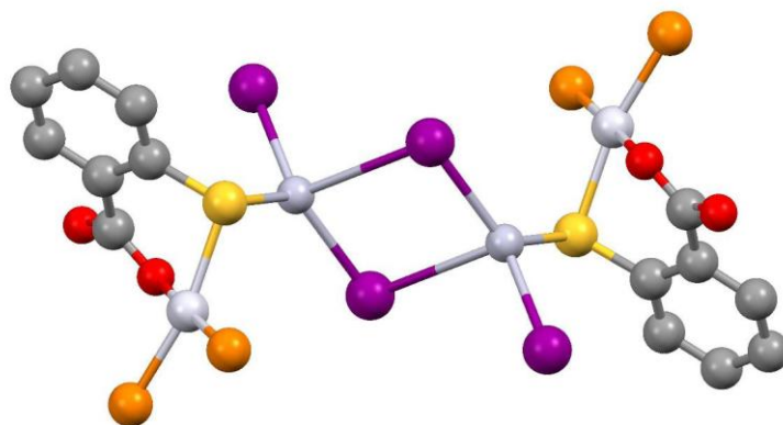
Слика 14. Кристална структура језгра комплекса [\text{Pt}(\text{SC}_6\text{H}_4\text{CO}_2)(\text{PPh}_3)_2 \cdot \text{HgI}_2]_2
