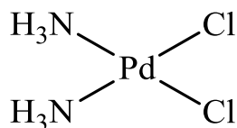
Слика 28. Структура комплекса cis -диаминдихлоридопаладијум(II), cis-[PdCl_2(NH_3)_2] ;
