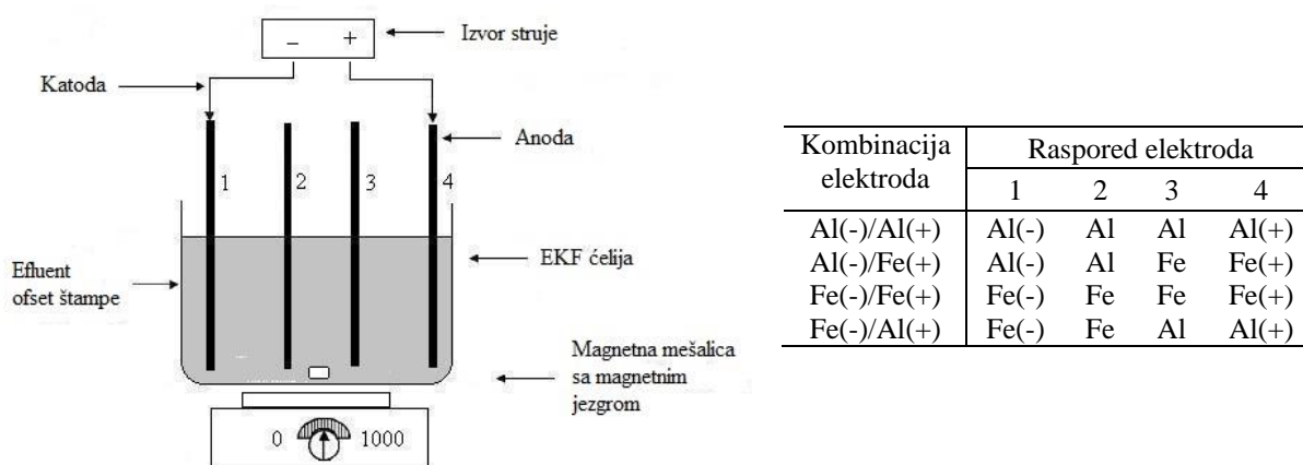
Slika 13. Šematski prikaz šaržnog EKF reaktora za tretman efluenata ofset štampe sa četiri različite kombinacije elektroda povezanih u bipolarnom serijskom modu
