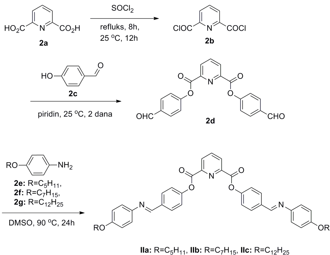
Šema 2. Reakcioni niz sinteze di[4-(4- n -alkiloksifeniliminometil)fenil]piridin-2,6-dikarboksilata ( IIa–IIc )
