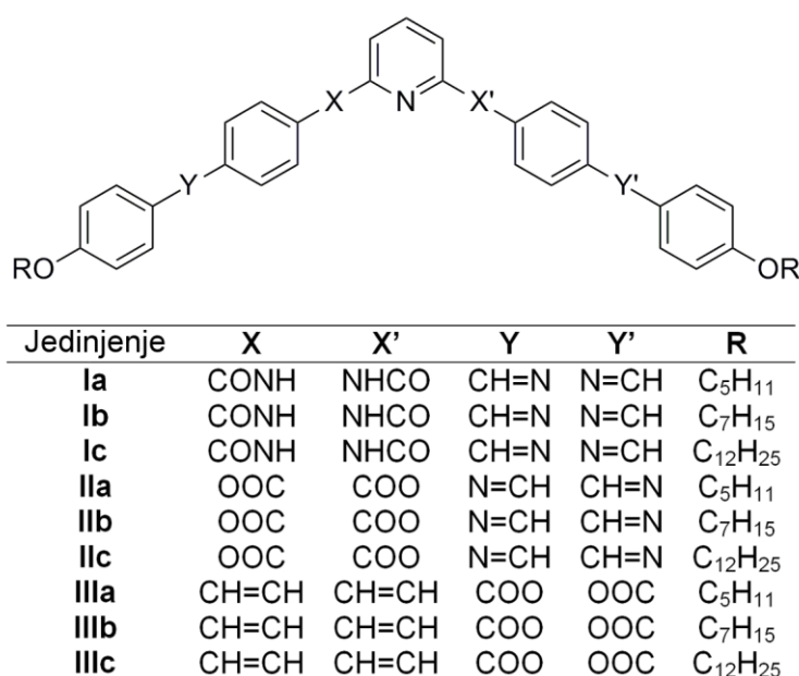
Slika 41. Hemijske strukture proučavanih tečnih kristala oblika banane sa piridinom kao centralnim prstenom
