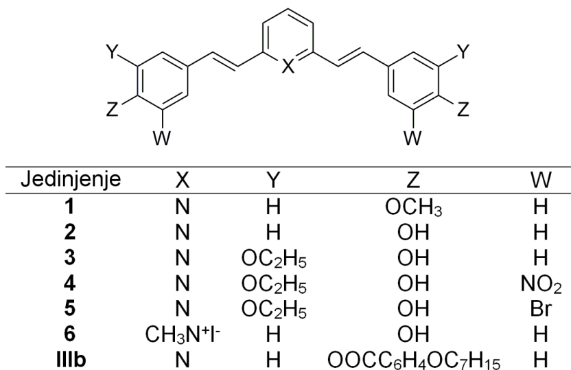
Slika 52. Hemijske strukture proučavanih derivata 2,6-distirilpiridina
