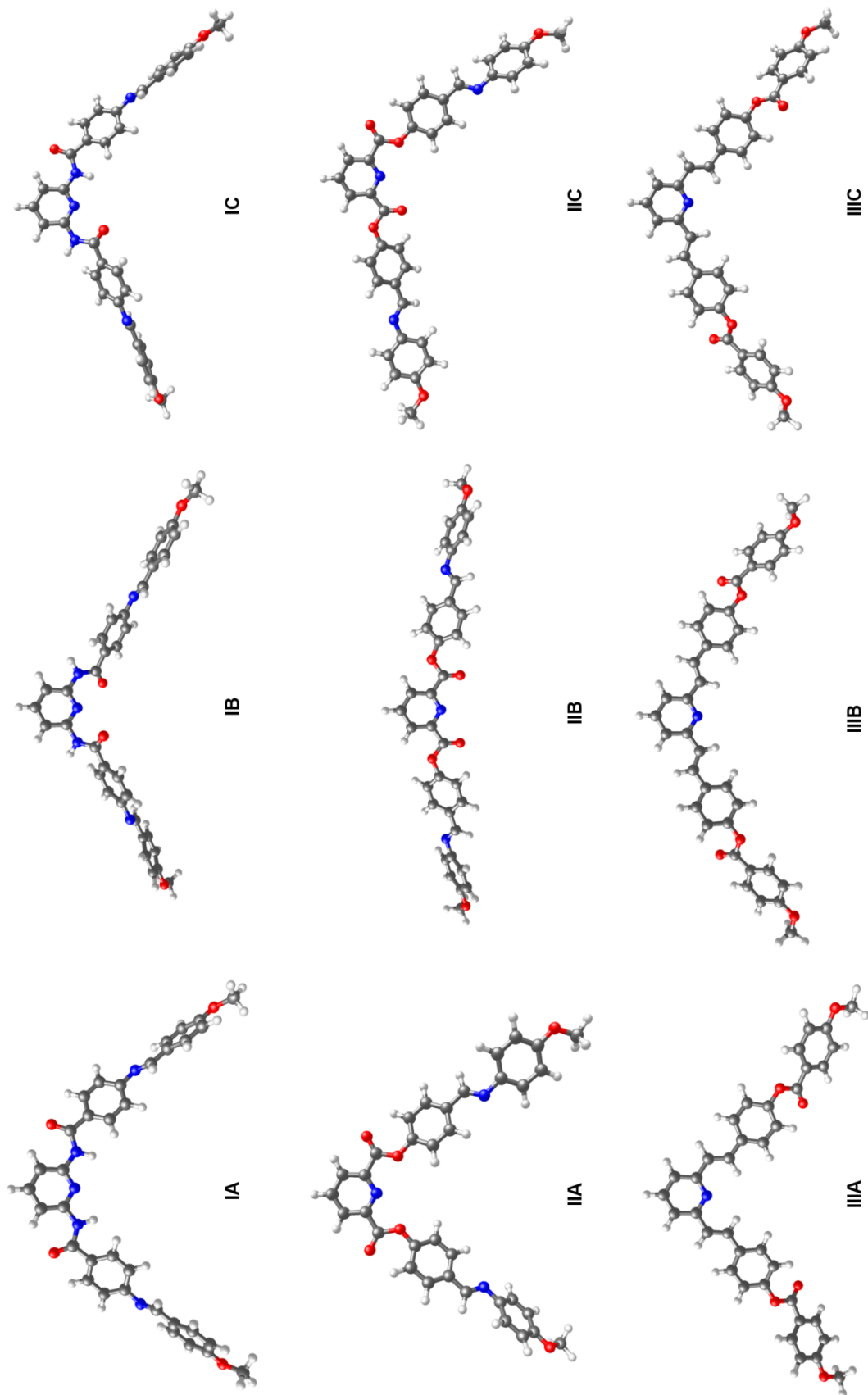
Slika 49. Stabilni konformeri uprošćenih sistema I, II i III
