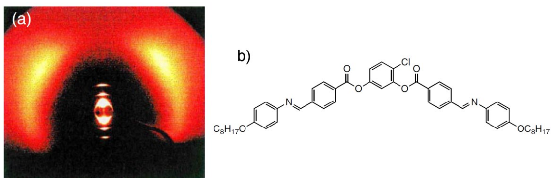
Slika 17. a) 2D difraktogram B2 mezofaze jedinjenja prikazanog pod b) [14]
