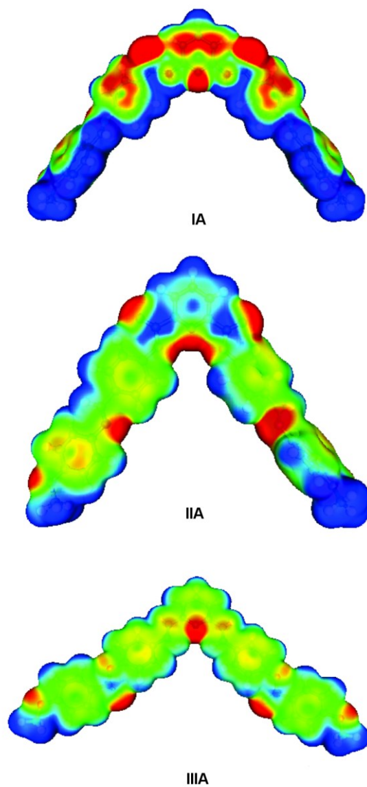
Slika 50. Površine elektrostatičkog potencijala najstabilnijih konformera za svaki od navedenih sistema I , II i III (plava boja – pozitivan deo, zelena boja – neutralan deo, crvena boja – negativan deo molekula)
