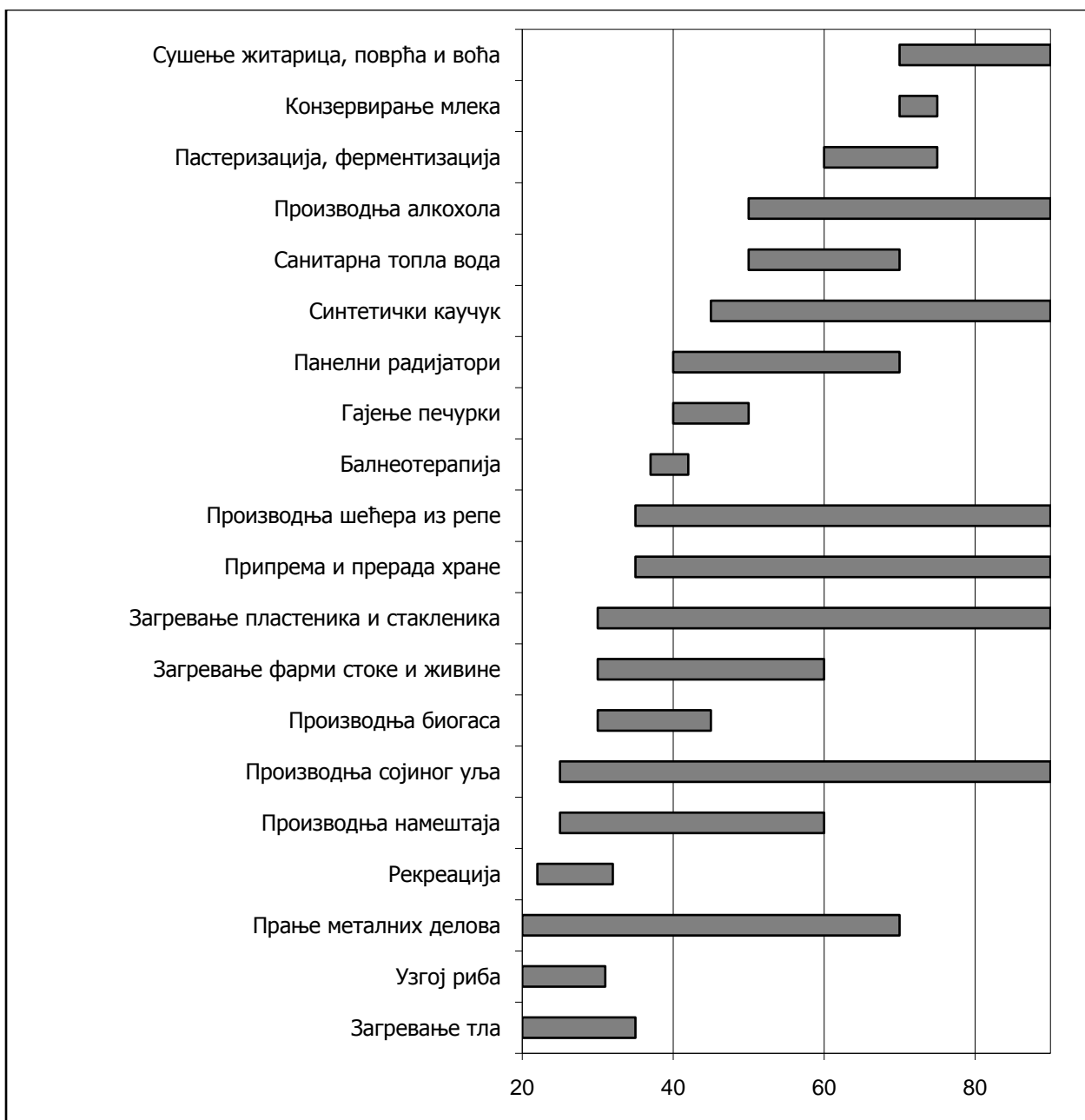
Слика 2. Линдалов дијаграм [61]
