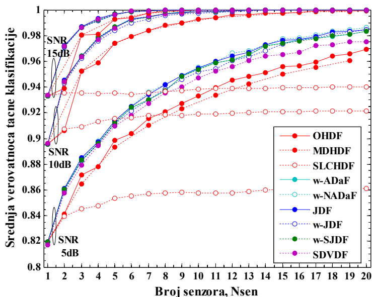
Sl.4.10 - Poređenje AMC performansi rešenja za kooperativnu AMC za AWGN kanal u slučaju SGS scenarija za SNR_g \in \{5dB, 10dB, 15dB\} pri primeni HDF, SDF i DaF metoda, za N_{sim} = 500 .
