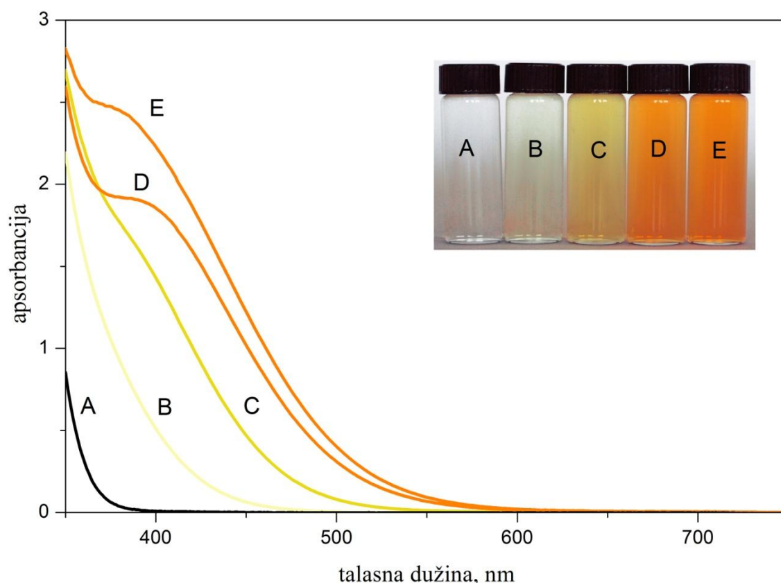
Slika 3.19. ApSORPCIONI spektri površinski modifikovanih \text{TiO}_2 ( 45 \text{ \AA} ) nanočestica (20 mM, u rastvoru metanol/voda=90/10, pH 2) sa različitim ligandima (0,33 mM). A: čist \text{TiO}_2 ; B: 2HBA; C: 3H2NA; D: 3,5DH2NA; E: 3,7DH2NA. Molekulske strukture liganada su predstavljene u Tabeli 3.5.
