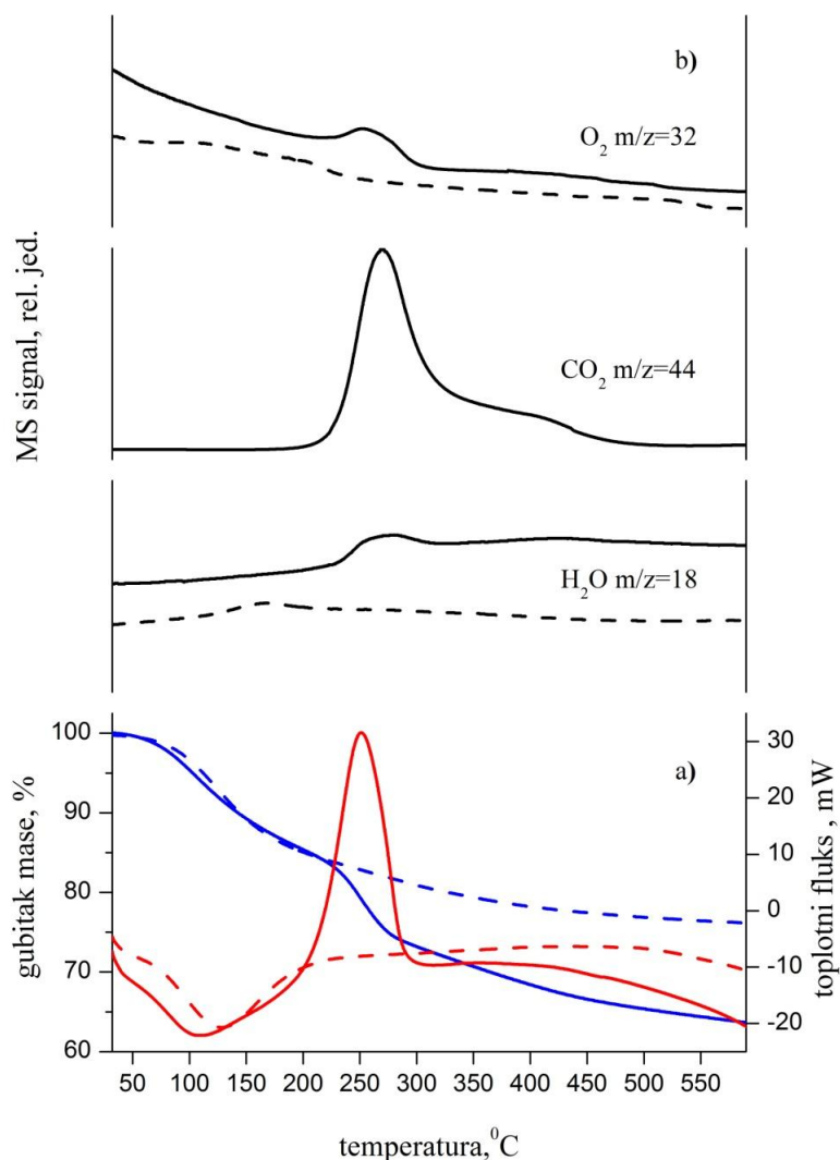
Slika 3.41. TG i DSC krive nanočestica \text{TiO}_2 (isprekidana linija) i nanočestica \text{TiO}_2 modifikovanih 2HBA (puna linija) snimljene pri brzini zagrevanja od 10\text{ }^\circ\text{C}/\text{min} u struji helijuma a) (TG-plava linija; DSC-crvena linija). MS signali molekulskih vrsta i njihovo izdvojanje sa temperaturom b).
