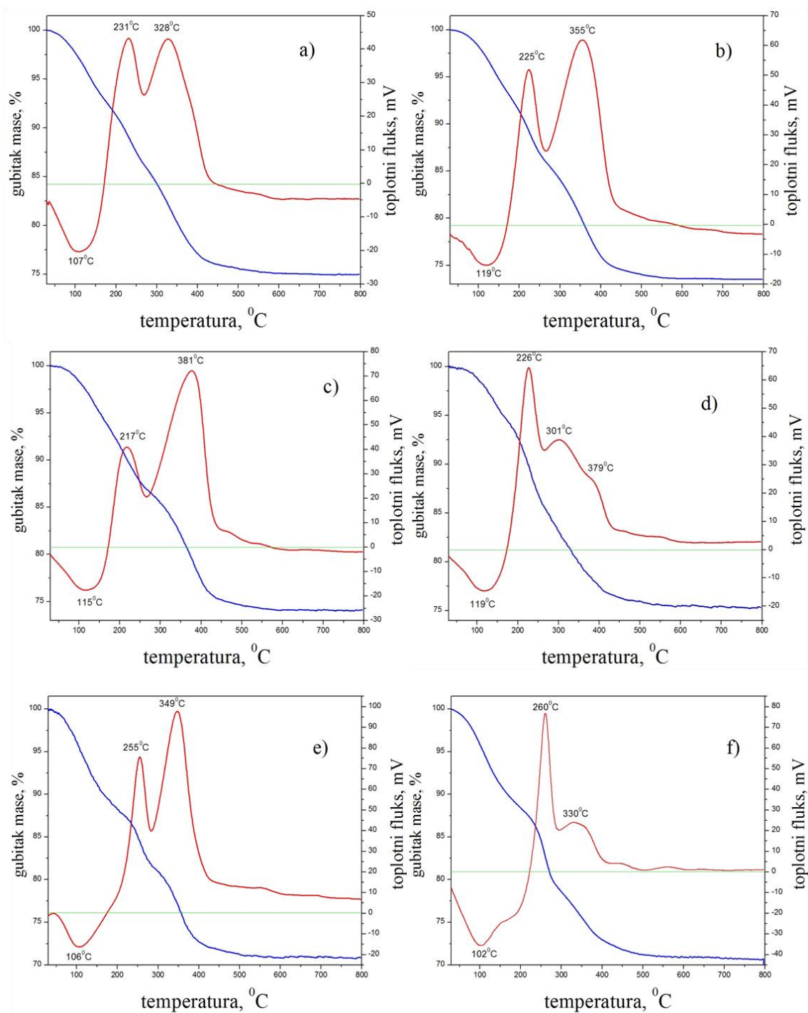
Slika A8. TG (plave linije) i DSC (crvene linije) krive nanočestica TiO 2 modifikovanih a) CAT, b) 3MetCAT, c) 4MetCAT, d) 3MethoxyCAT, e) 3,4DHBA i f) 4NitCAT snimljene pri brzini zagrevanja od 20 °C/min u struji vazduha.
