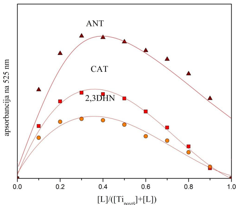
Slika 3.4. Džbove krive ekvimolarnih rastvora za \text{TiO}_2 - ligand komplekse; [\text{Ti}_{\text{površ}}] + [\text{L}] = \text{konstantno (1 mM)} .
