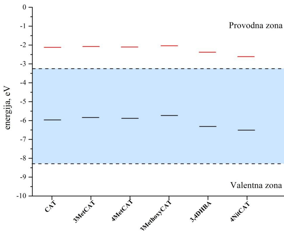
Slika 3.16. Položaji HOMO (crne linije) i LUMO (crvene linije) energetske nivoa za razmatrane CT komplekse u odnosu na energetski procep klastera \text{Ti}_2\text{O}_3(\text{OH})_2 .
