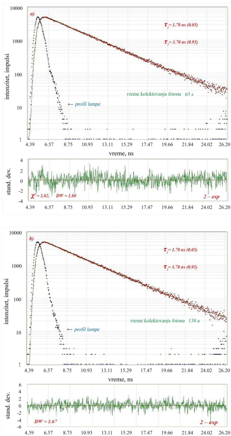
Slika A19. Kriva zavisnosti gašenja fluorescencije u vremenu za 50 \mu\text{M} 1,4DH2NA (a) i 50 \mu\text{M} 1,4DH2NA + 130 \mu\text{M} Ti_{\text{površ}} (b) u rastvorima metanol/voda=90/10 na pH 2. Emisija je merena na 450 nm nakon ekscitacije talasnom dužinom od 342 nm. Parametri analiziranja bieksponecijalne krive (distribucija reziduala, \chi^2 i DW parametar) dati su na slici.
