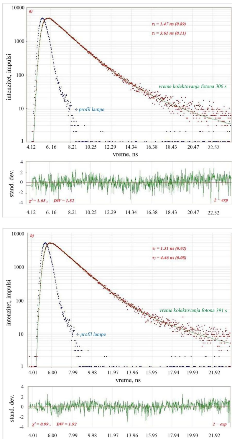
Slika 3.26. Kriva zavisnosti gašenja fluorescencije u vremenu za 50 \mu\text{M} 3\text{H}_2\text{NA} (a) i 50 \mu\text{M} 3\text{H}_2\text{NA} + 20 \mu\text{M} \text{Ti}_{\text{površ}} (b) u vodenim rastvorima na pH 3. Emisija je merena na 520 nm nakon ekscitacije talasnom dužinom od 342 nm. Parametri analiziranja bieksponencijalne krive (distribucija reziduala, \chi^2 i DW parametar) dati su na slici.
