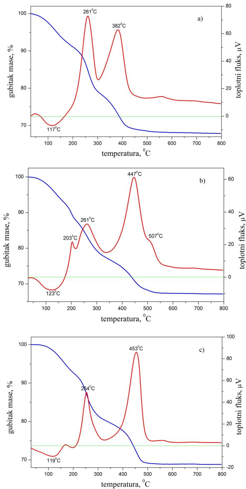
Slika A20. TG (plave linije) i DSC (crvene linije) krive nanočestica \text{TiO}_2 modifikovanih a) 2HBA, b) 1H2NA i c) 1,4DH2NA snimljene pri brzini zagrevanja od 20\text{ }^\circ\text{C}/\text{min} u struji vazduha.
