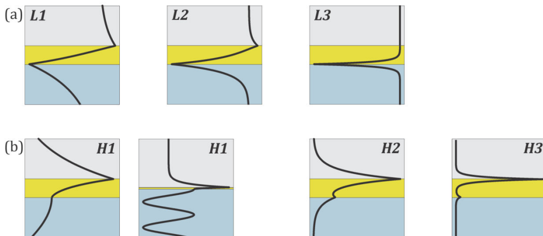
Slika 1.4: Raspodela magnetskog polja H_y za (a) asimetrične ( L1, L2, L3 ) i (b) simetrične ( H1, H2, H3 ) modove u asimetričnoj IMI strukturi.
