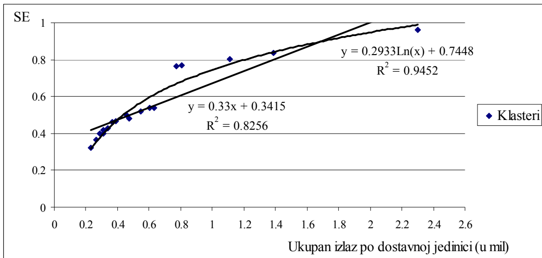
Slika 6.3 Veza između SE i ukupnog izlaza razmatrajući klaster
