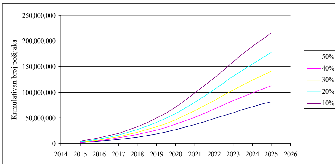
Slika 7.6 Prognoziran kumulativan broj pošiljaka nove usluge (2015-2025)
