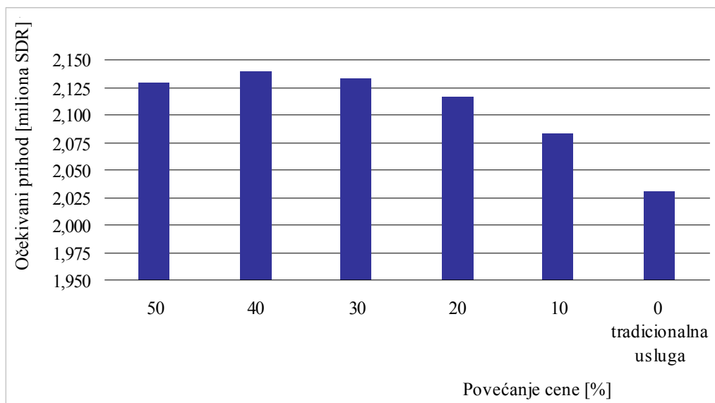
Slika 7.7 Prognozirani ukupan prihod JP "Pošta Srbije" (2015-2025)
