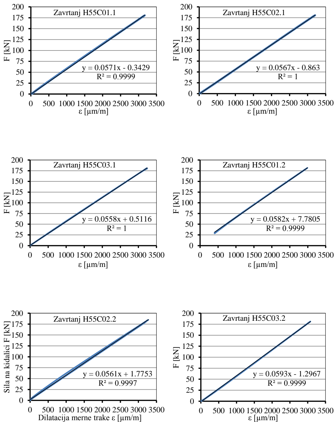
Slika C.18: Kalibracione krive za HBT zavrtnejeve ugrađene u uzorke H12 i H13
