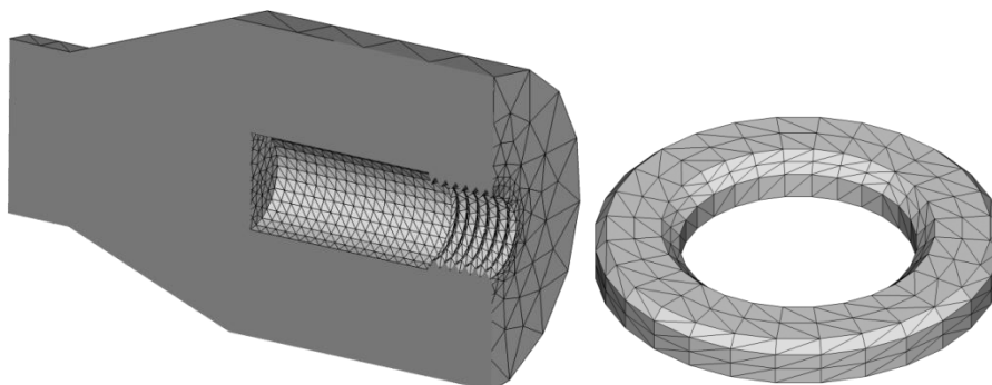
a) Alat za unošenje sile prednaprezanja b) Podloška za zavrtnjeve tipa HV
