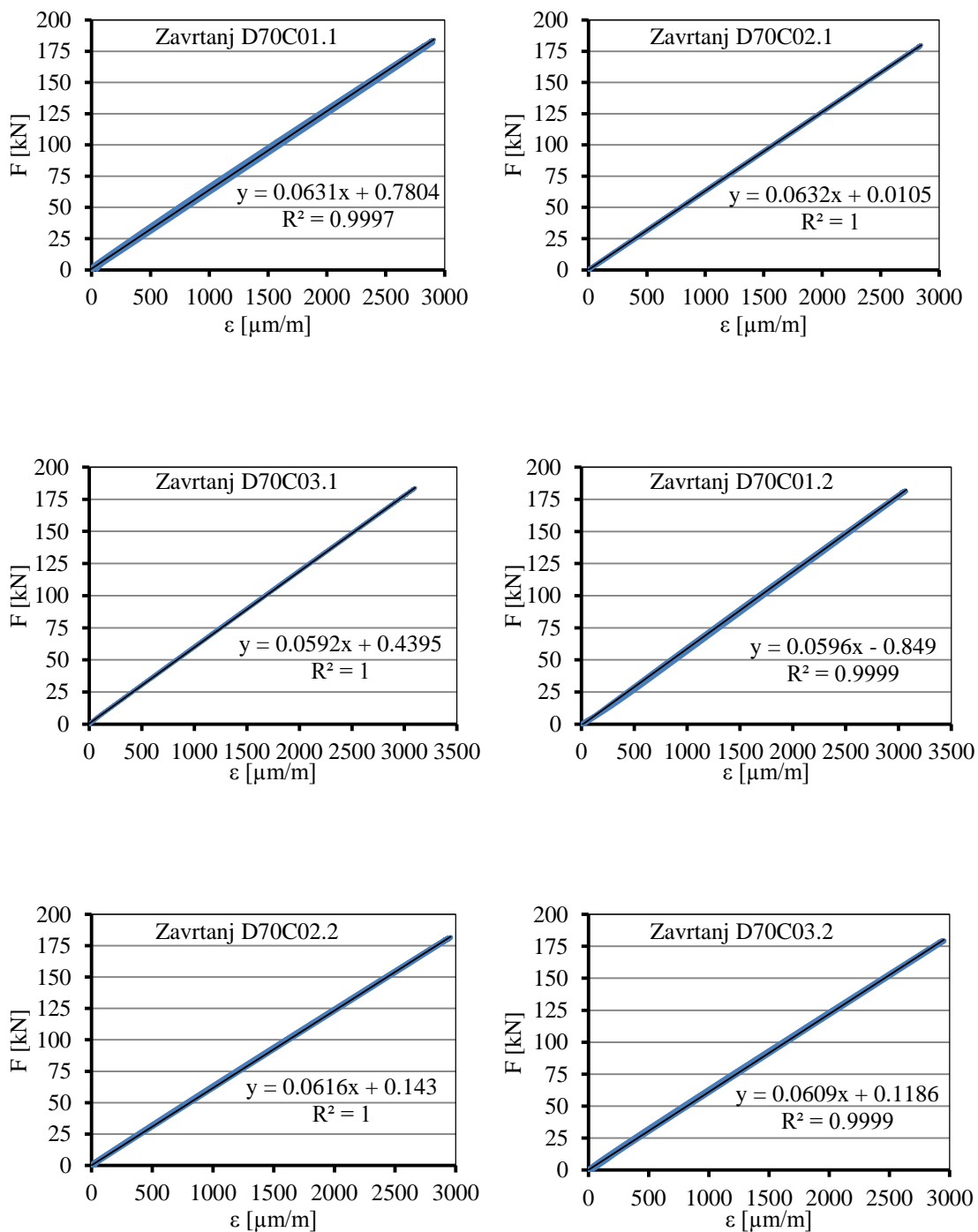
Slika C.14: Kalibracione krive za HV zavrtnjeve ugrađene u uzorke D16 i D17
