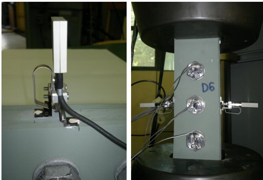
Slika 3.51: Fiksiranje alata za uzorak i ugradnja ekstenzometara
