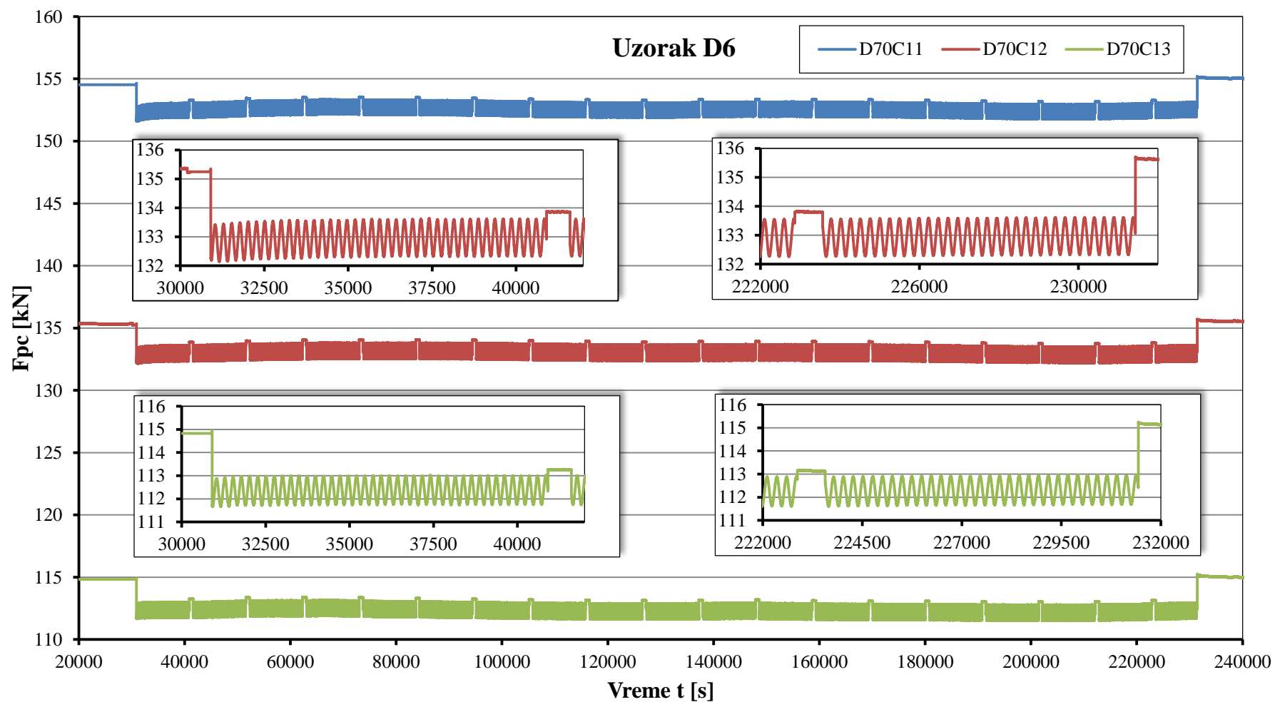
Slika 5.11: Promena sile prednaprezanja u zavrteljima uzorka D6 u toku delovanja dinamičkog opterećenja
