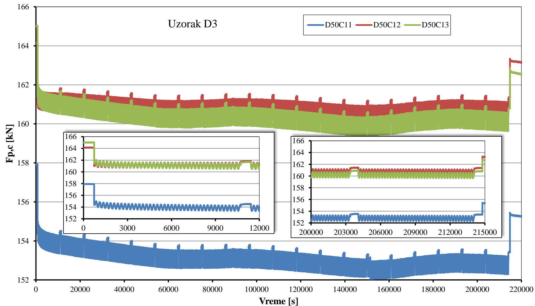
Slika 5.9: Promena sile prednapreznja u zavrtnjevima uzorka D3 u toku delovanja dinamičkog opterećenja
