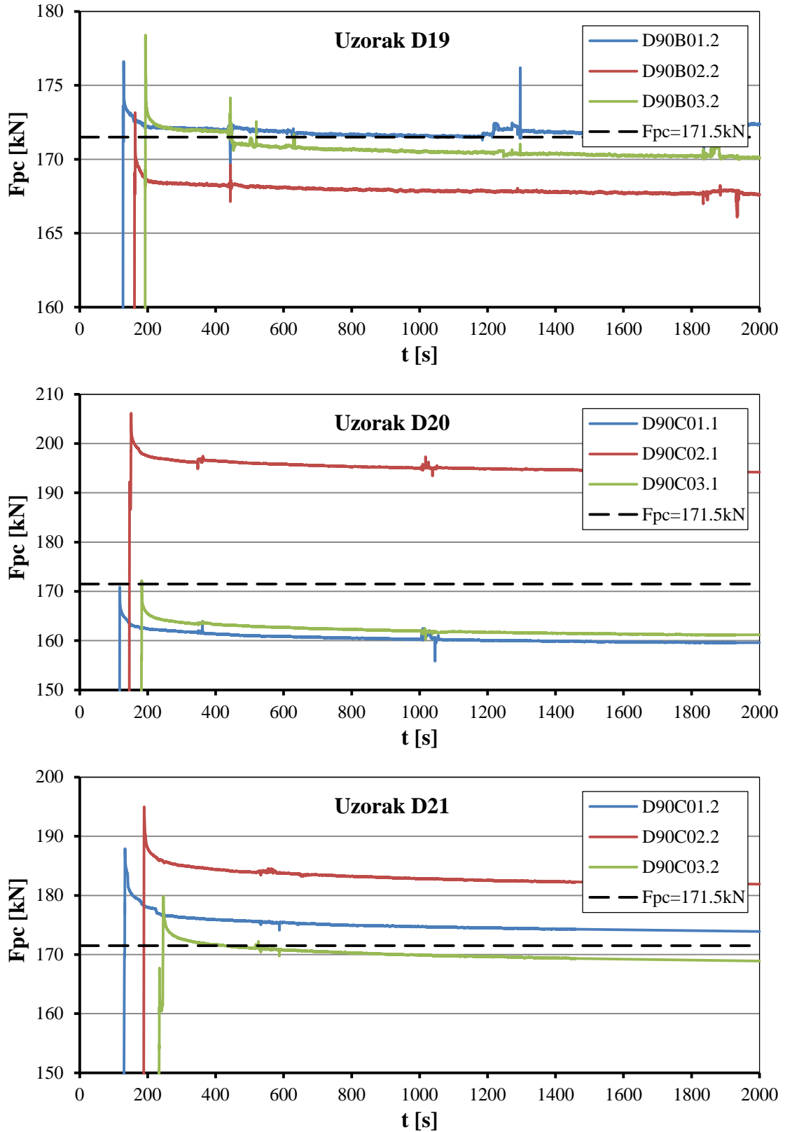
Slika D.7: Inicijalni gubici sile prednaprezanja u uzorcima D19, D20 i D21
