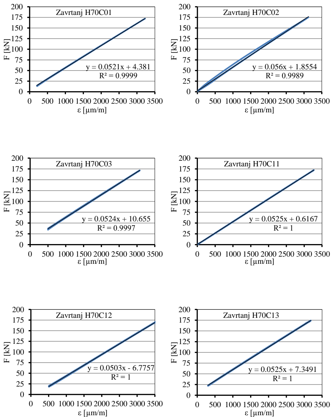
Slika C.8: Kalibracione krive za HBT zavrtanje ugrađene u uzorke H5 i H6
