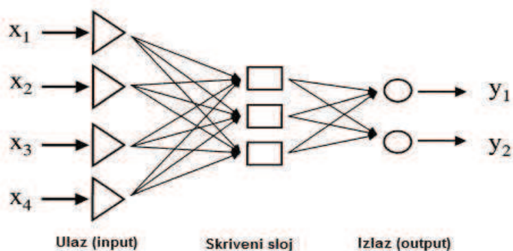
Slika 27. Višeslojna nerekurventna mreža 199
