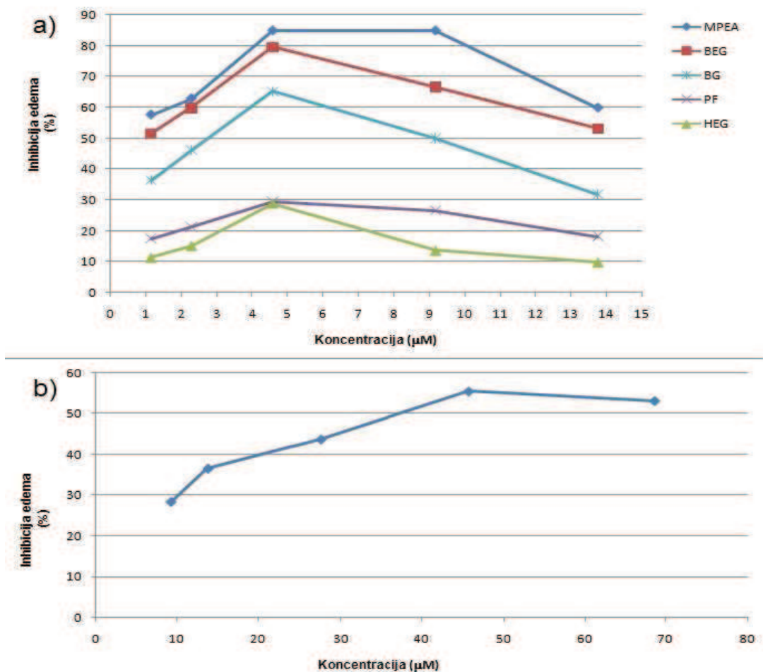
Slika 38. Krive zavisnosti inhibicije edema od primenjene koncentracije za a) MPEA, BEG, BG, PF, HEG i b) deksametazon
