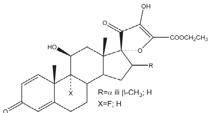
Slika 17. Spiroenonski derivati glukokortikoida
