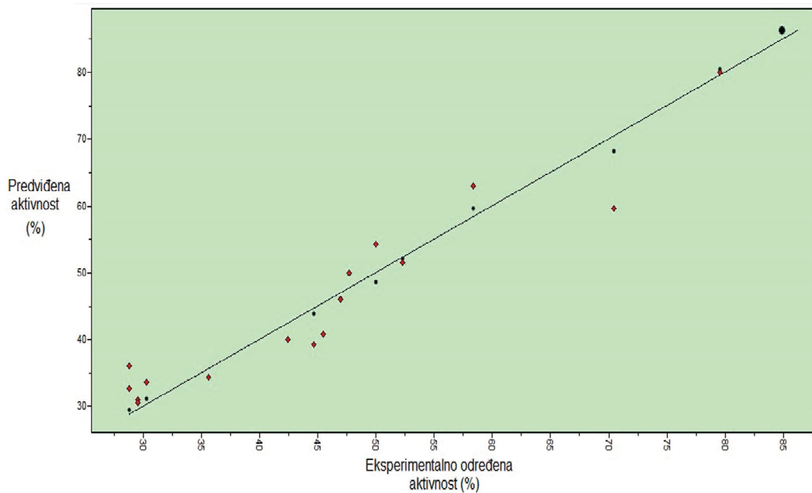
Slika 39. Zavisnost eksperimentalno određenih i predviđenih vrednosti maksimalne inhibicije edema (%) za jedinjenja iz trening seta (crveni rombovi) i test seta (crni kružići)
