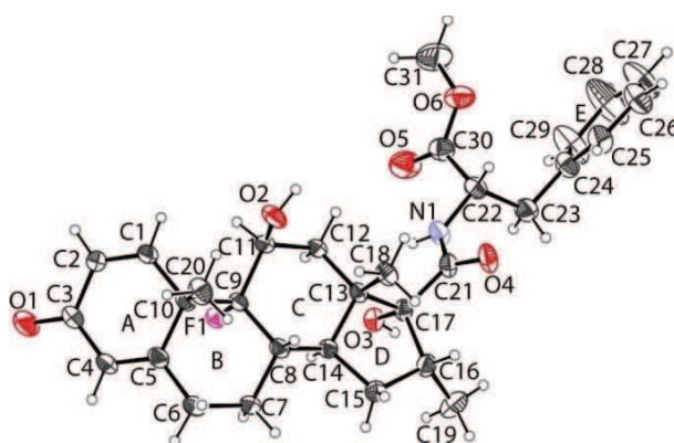
Slika P1. Molekulska struktura DF
