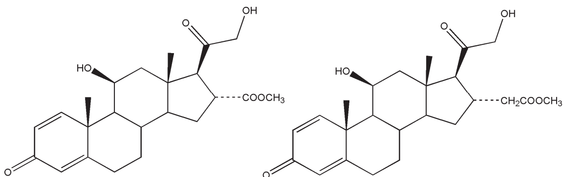
Slika 10. C16 karboksilatni estri
