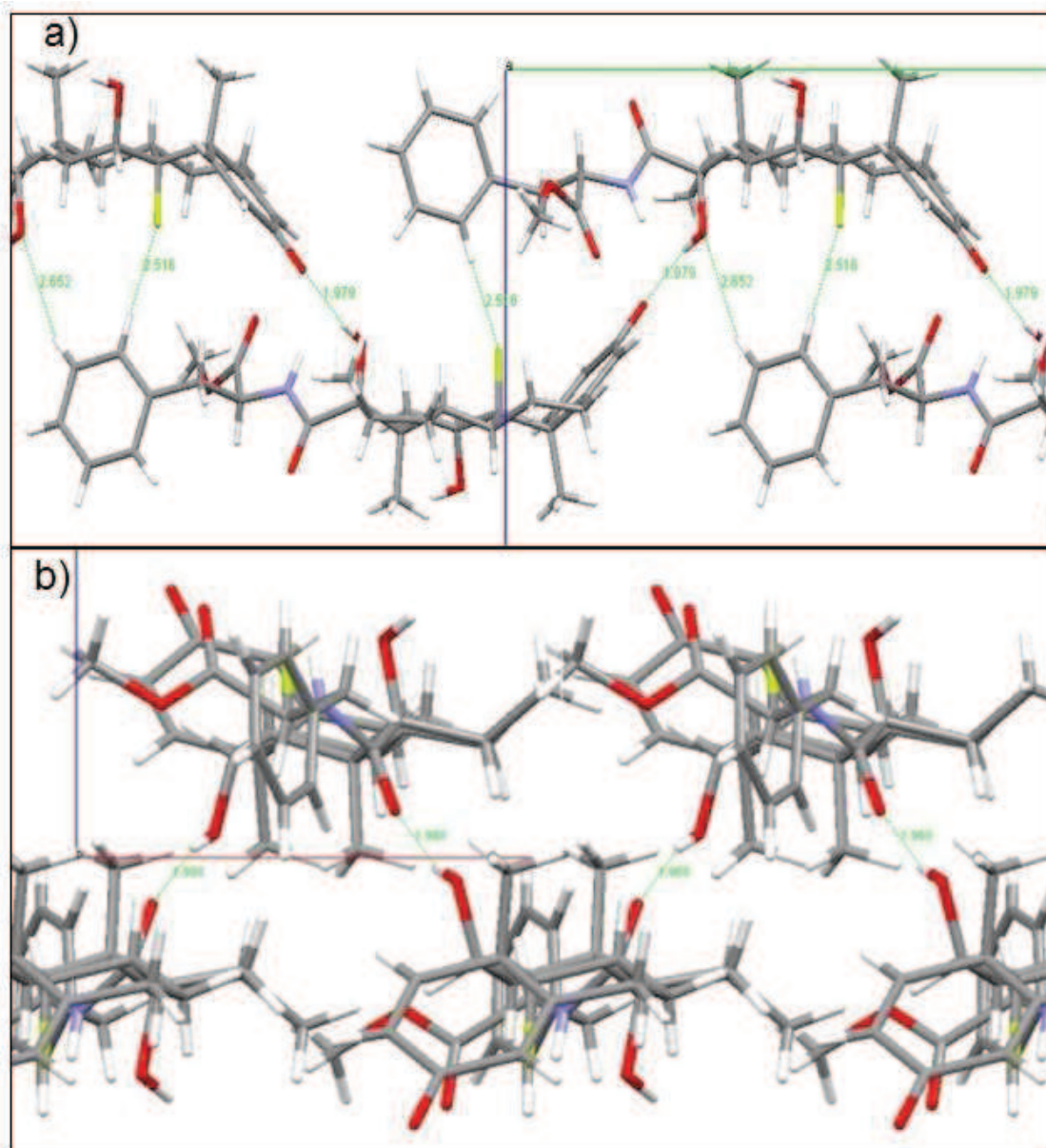
Slika P2. Kristalna struktura derivata DF: a) [100] O3–H...O1, C28–H...O3 i C29–H...F1 vodonične veze, i b) [010] O2–H...O4 vodonične veze. Vodonične veze su prikazane u obliku zelenih isprekidanih linija.
