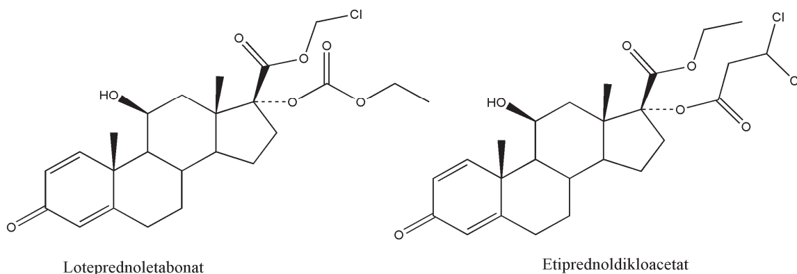
Slika 14. Loteprednoletabonat i etiprednoldikloacetat
