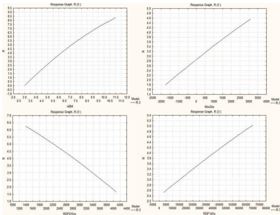
Slika 33. Grafici odgovora deskriptora koji formiraju ANN-QSPR( R ) model 231
