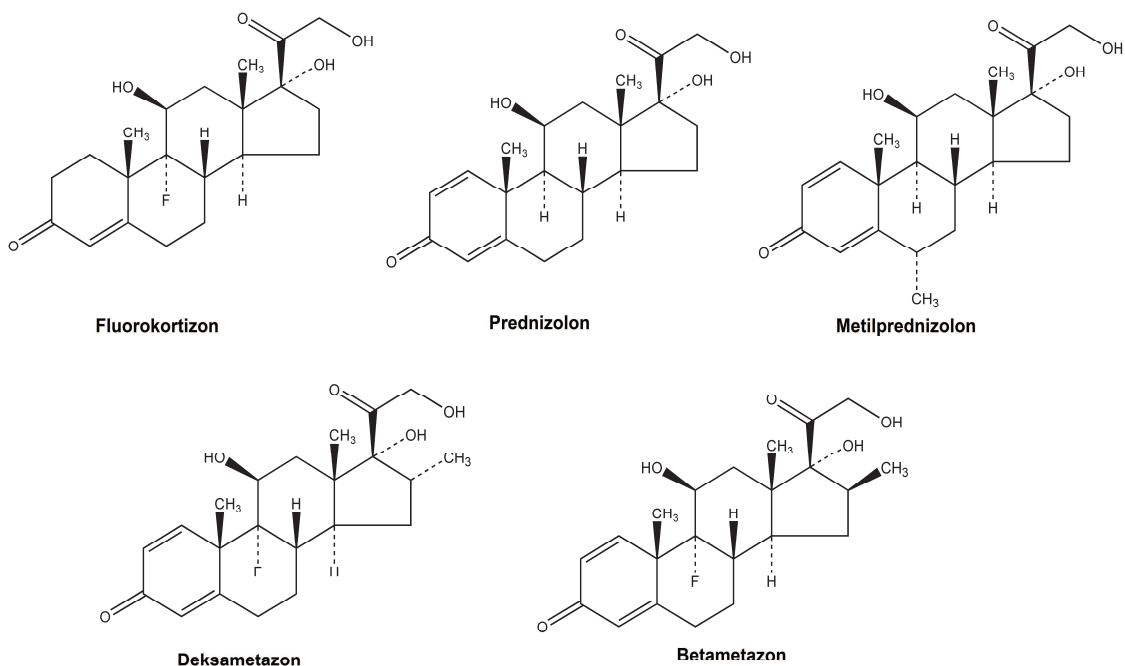
Slika 2. Strukture glukokortikoida dobijenih hemijskim modifikacijama položaja C1-C2, C6 \alpha , C9 \alpha i C16 \alpha hidrokortizona
