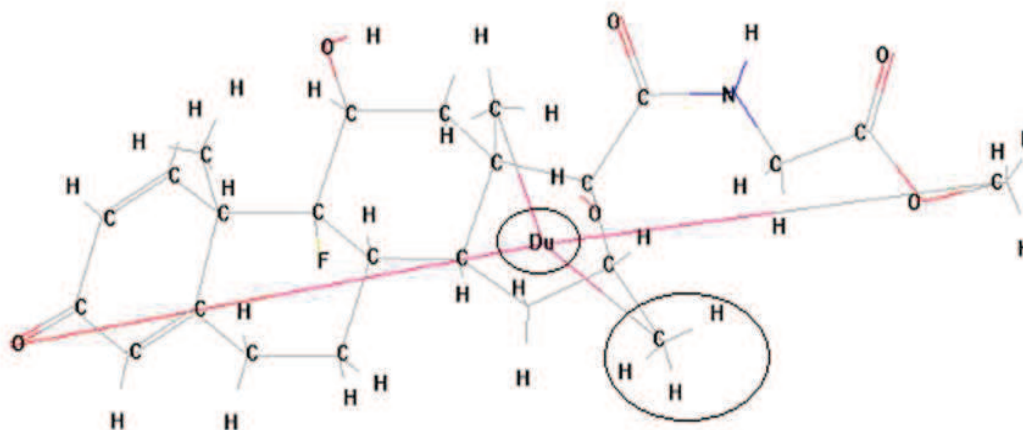
Slika 34. Trodimenzionalna struktura jedinjenja DG sa geometrijskim centrom 231
