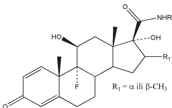
Slika 16. 17 \beta -karboksamidni derivati glukokortikoida
