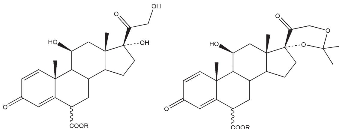
Slika 9. C6-karboksilatni estar prednizolona i odgovarajući ketal
