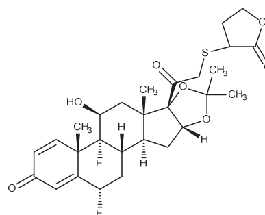
Glaxo \gamma -lakton
