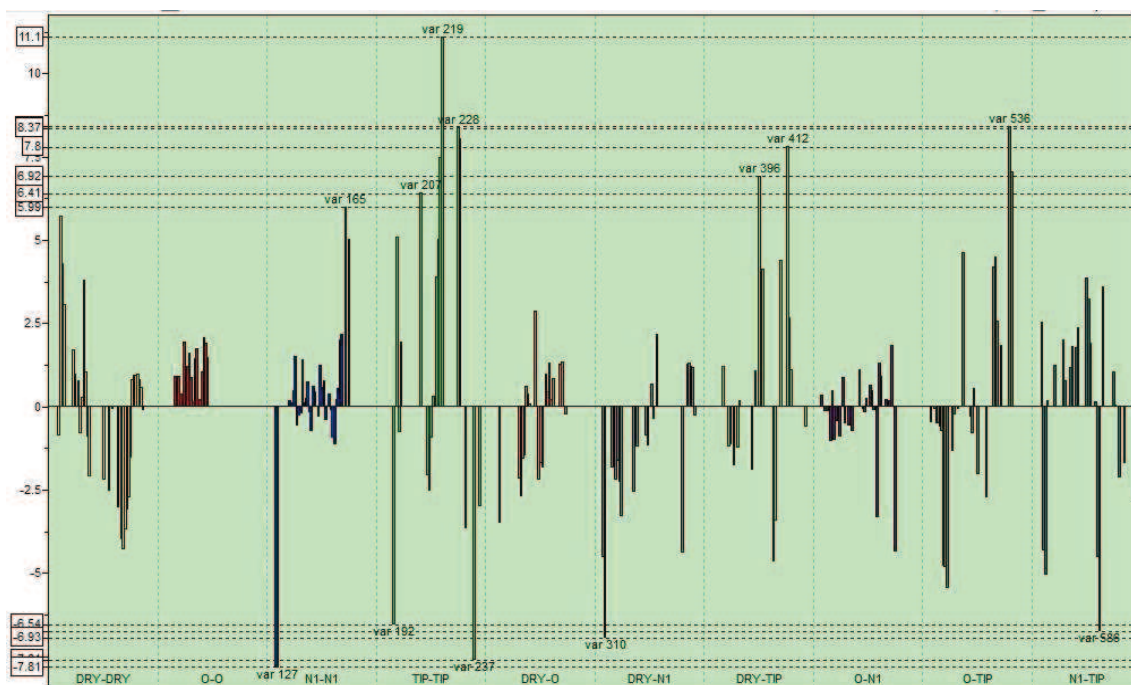
Slika 40. Grafik PLS regresionih koeficijenata najuticajnijih varijabli u 3D-QSAR modelu
