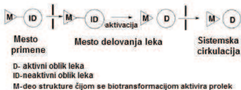
Slika 19. Šematski prikaz koncepta proleka 74
