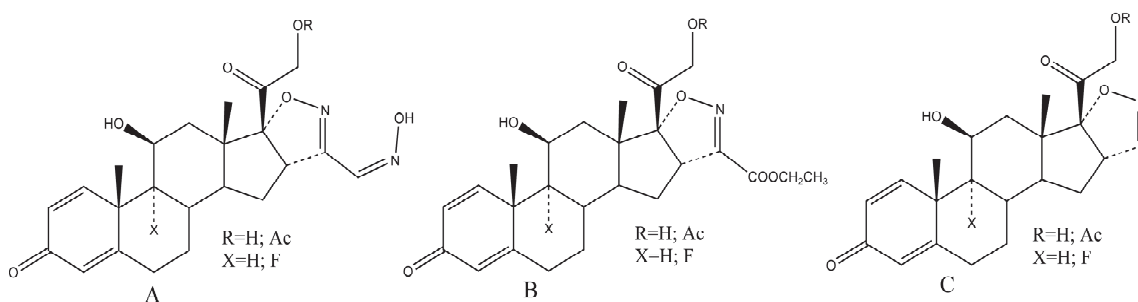
Slika 11. Izoksazolinski i oksimski derivati glukokortikoida
