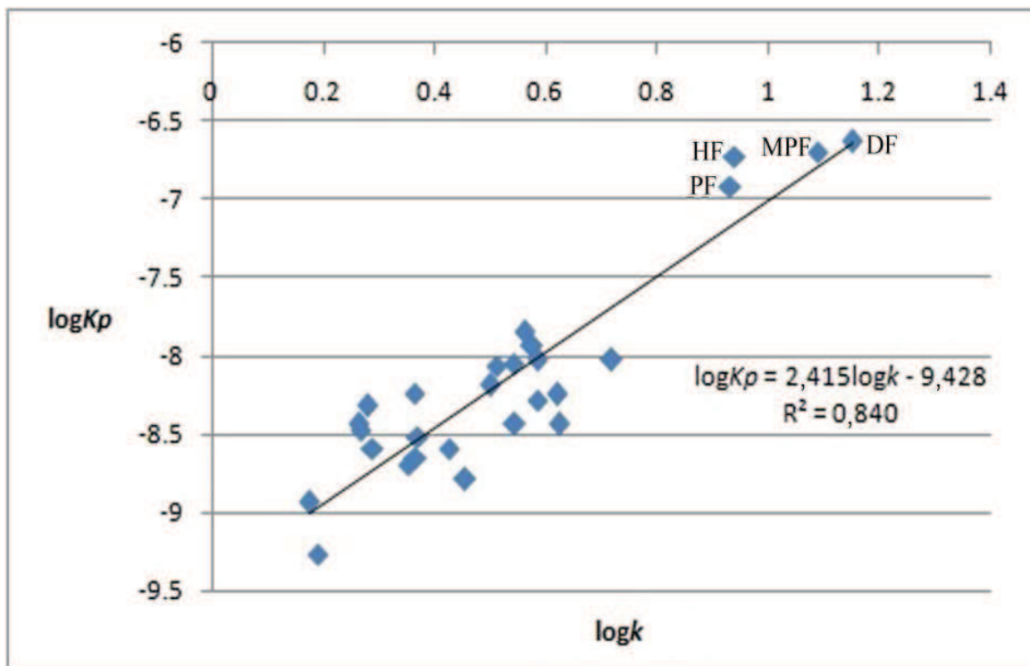
Slika 35. Korelacija između \log k i \log K_p vrednosti 223
