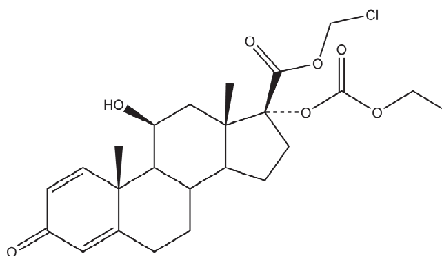
Slika 4. Hemijska struktura loteprednoletabonata
