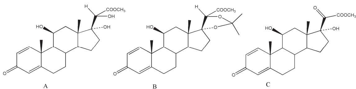
Slika 12. C21 karboksilati sa redukovanom (A i B) i neredukovanom (C) keto grupom na položaju C20
