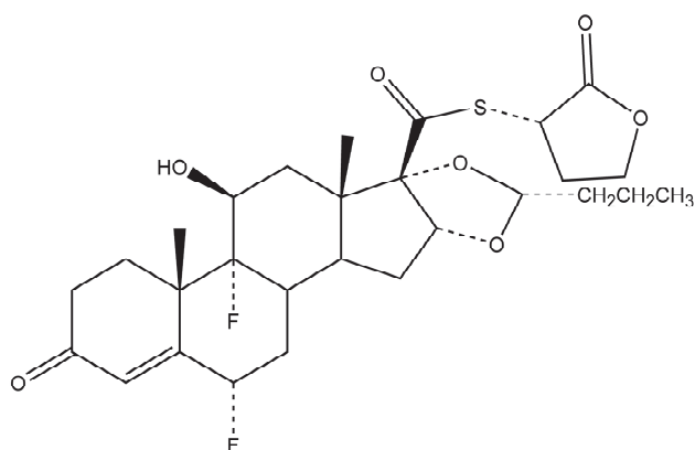
Slika 18. \gamma -butirolaktonski derivati glukokortikoida
