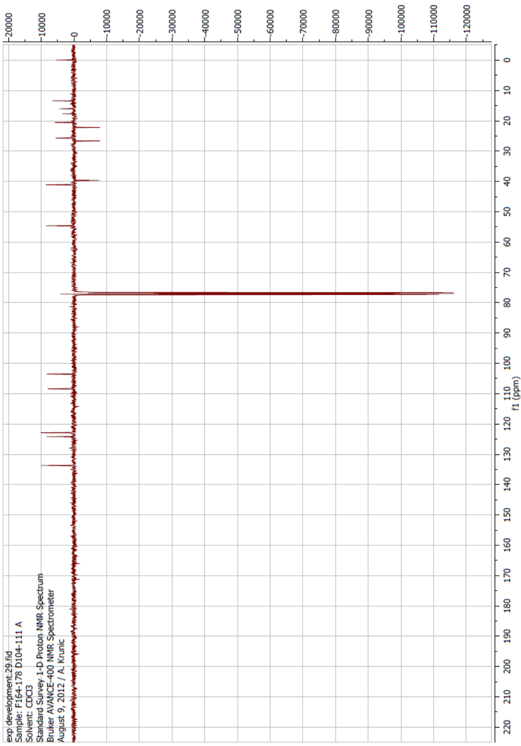
Slika 75. DEPT-Q spektar jedinjenja 8
