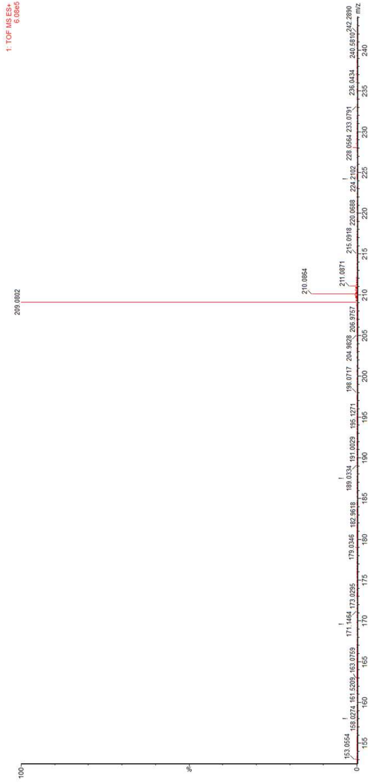
Slika 51. HR-MS spektar jedinjenja 1
