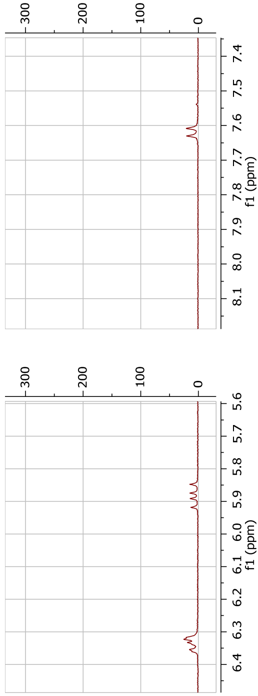
Slika 57. Prošireni detalji ^1\text{H} NMR spektra jedinjenja 3
