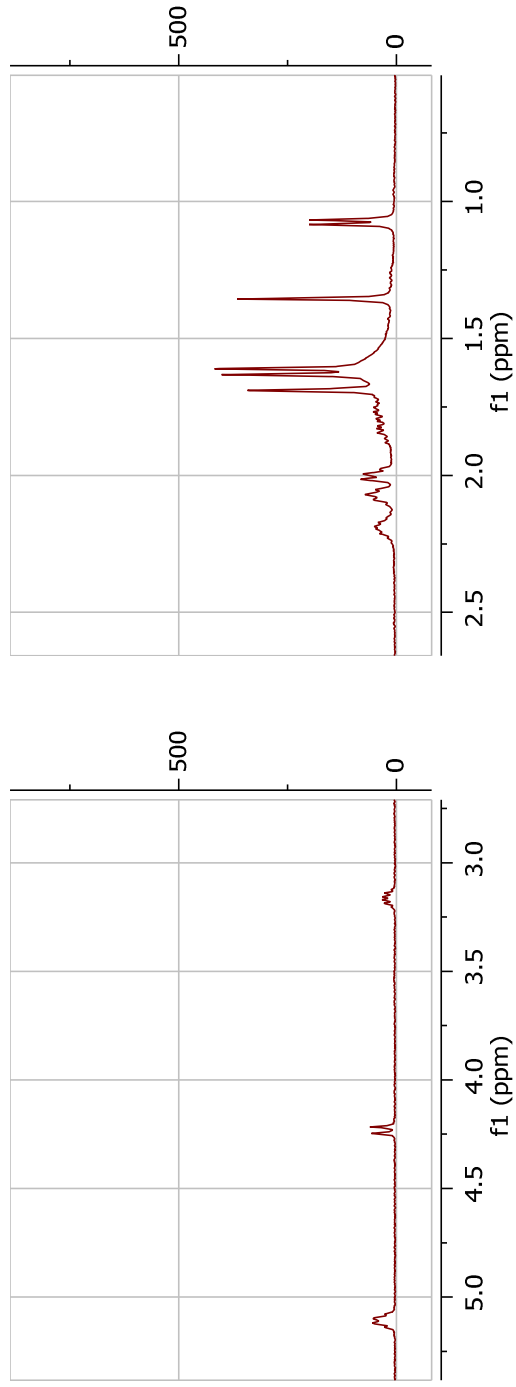
Slika 74. Prošireni detalji ^1\text{H} NMR spektra jedinjenja 8
