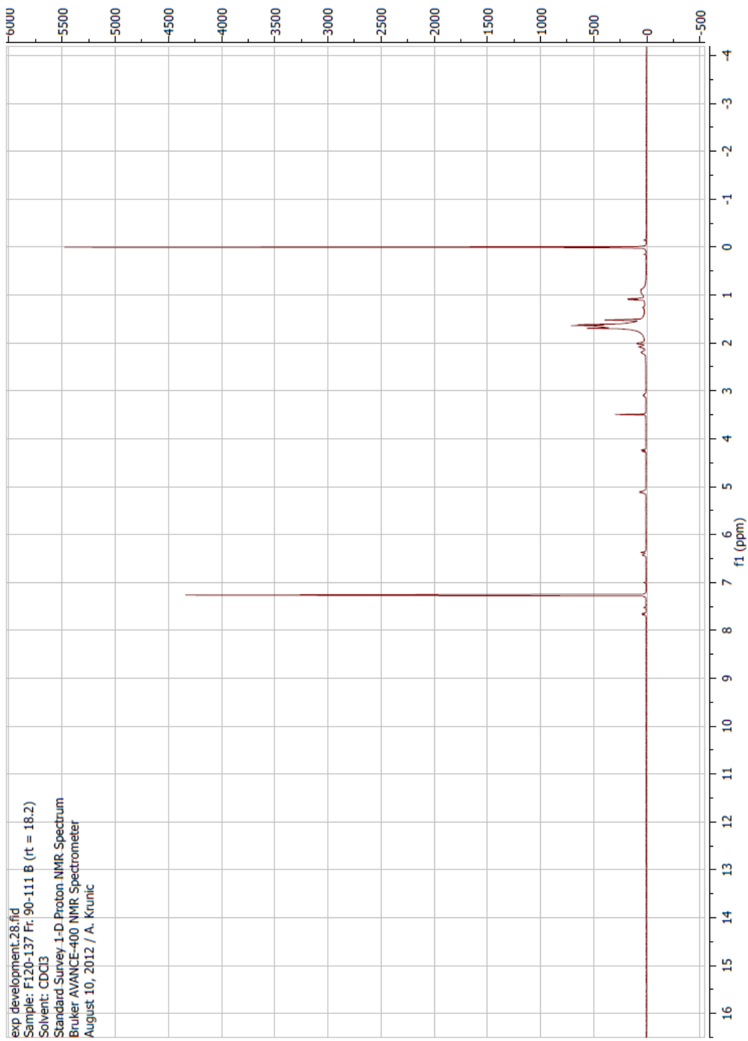
Slika 63. 1 H NMR spektar jedinjenja 5
