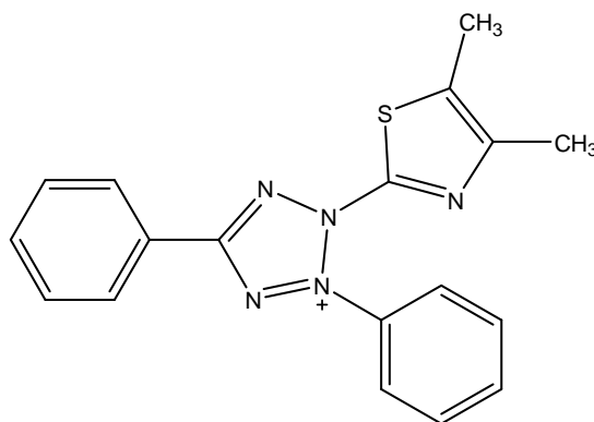
Slika 6. Hemijska struktura MTT-a
