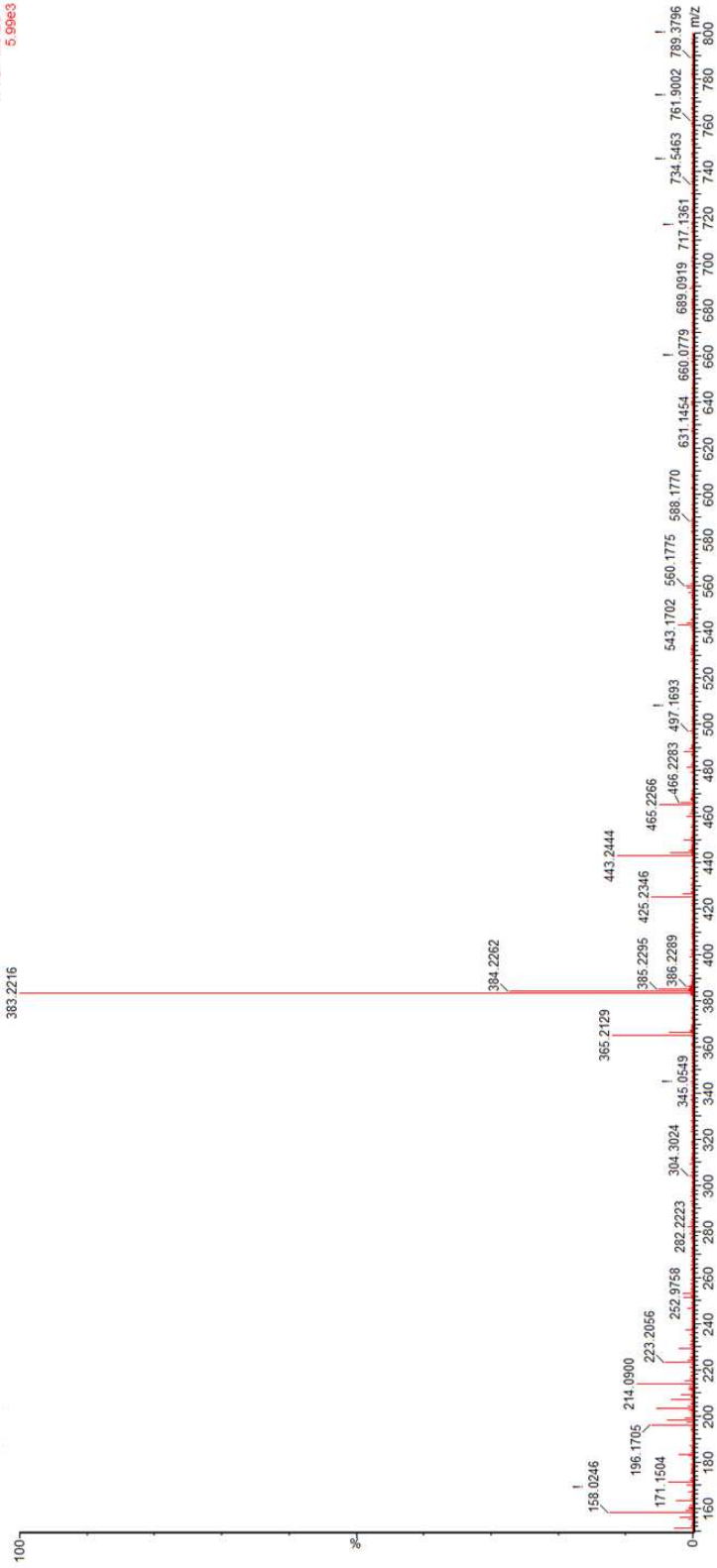
Slika 69. HR-MS spektar jedinjenja 7
