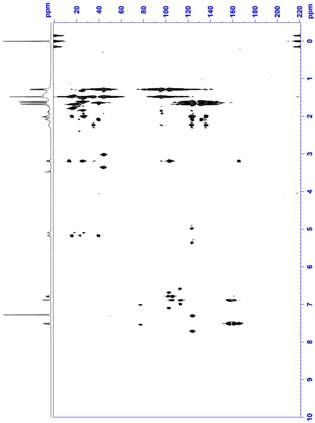
Slika 79. HMBC spektar jedinjenja 9
