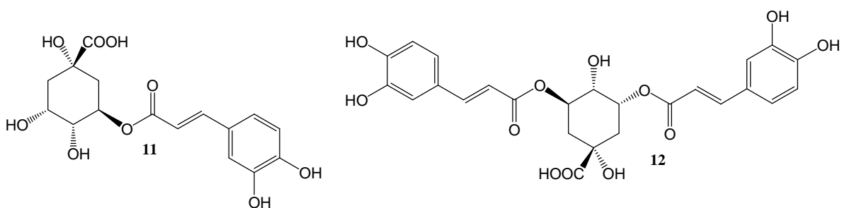
Slika 25. Hlorogenska kiselina (jedinjenje 11 ) i 3,5-dikafeoilhina kiselina (jedinjenje 12 ).
