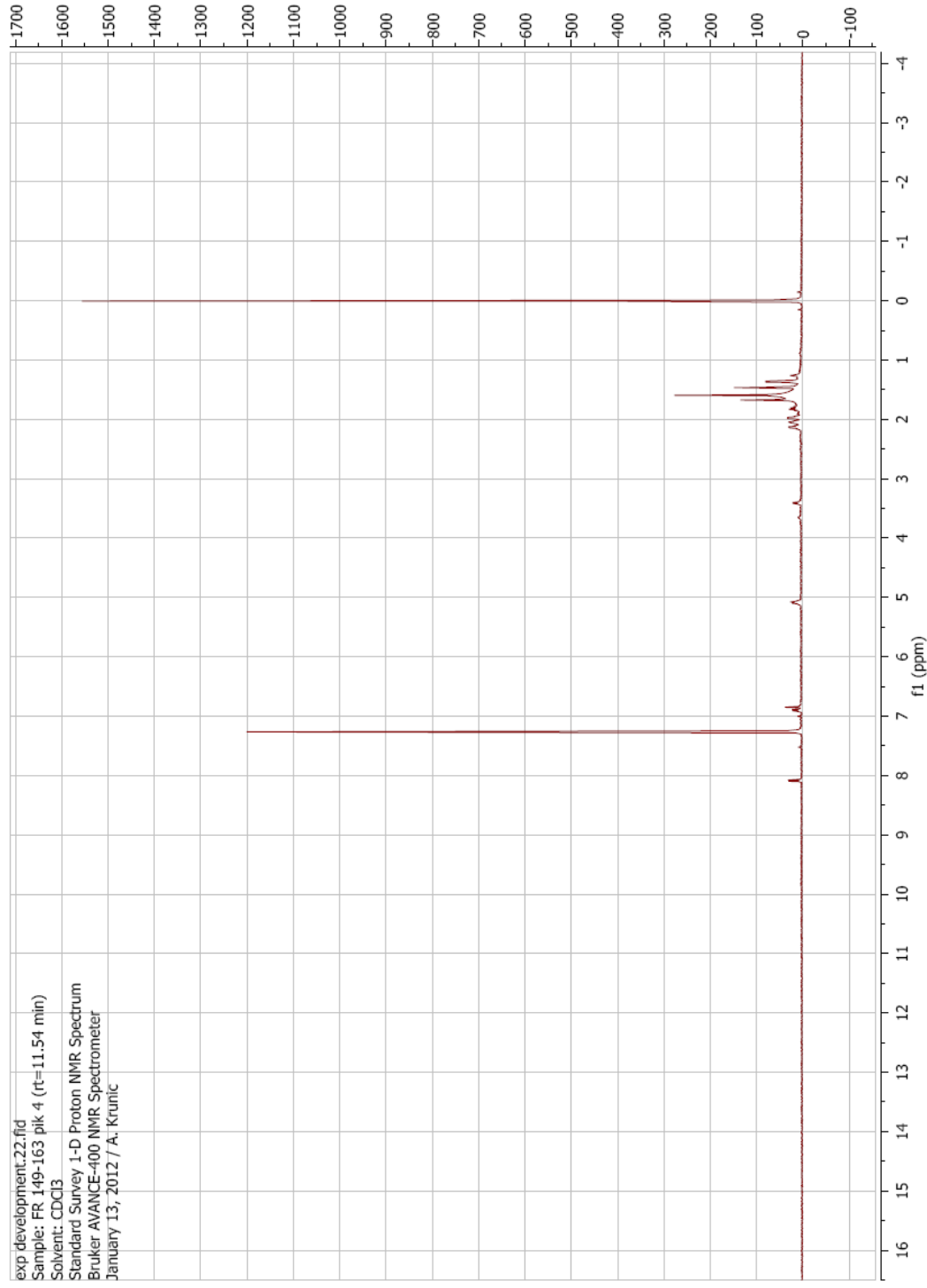
Slika 81. 1 H NMR spektar jedinjenja 10
