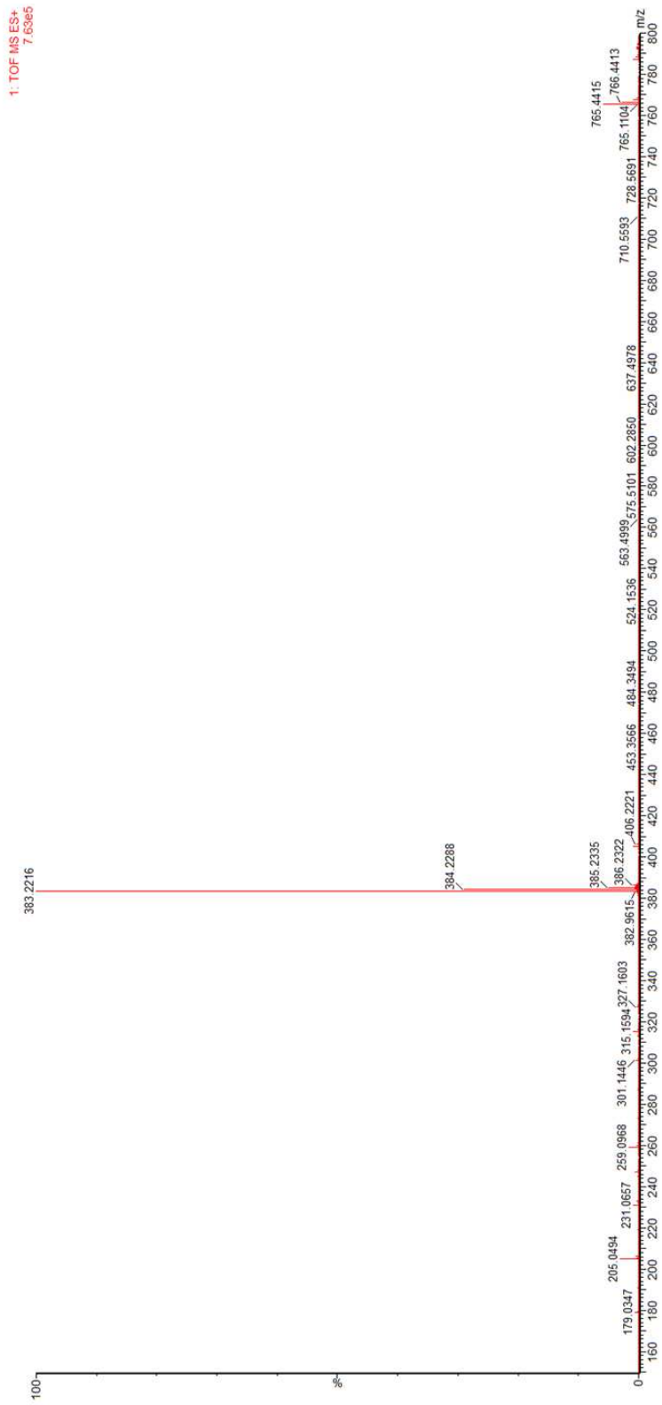
Slika 65. HR-MS spektar jedinjenja 6
