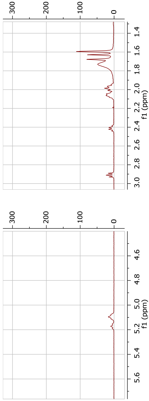
Slika 60. Prošireni detalji ^1\text{H} NMR spektra jedinjenja 4
