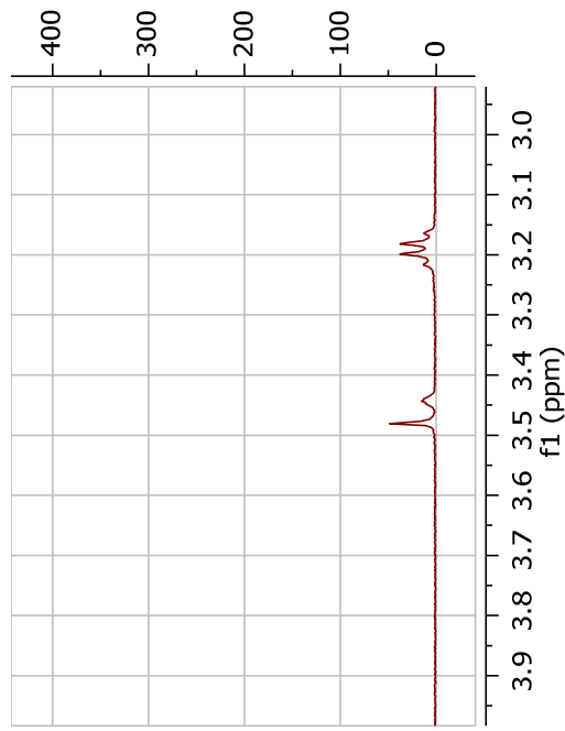
Slika 78. Prošireni detalji ^1\text{H} NMR spektra jedinjenja 9
