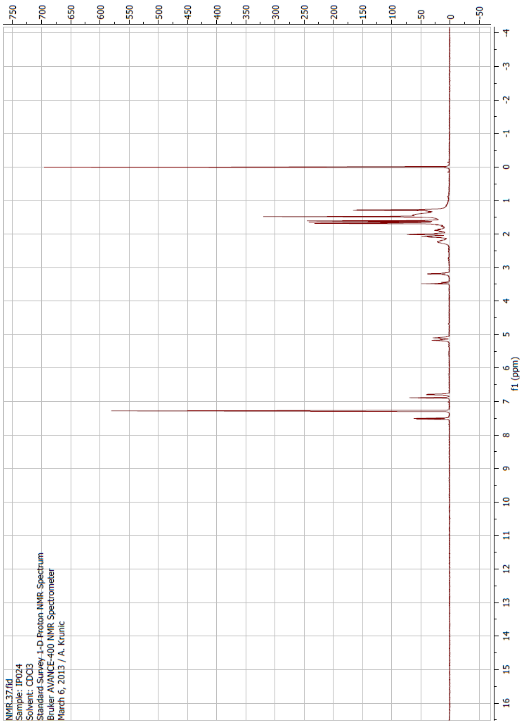
Slika 77. ^1\text{H} NMR spektar jedinjenja 9
