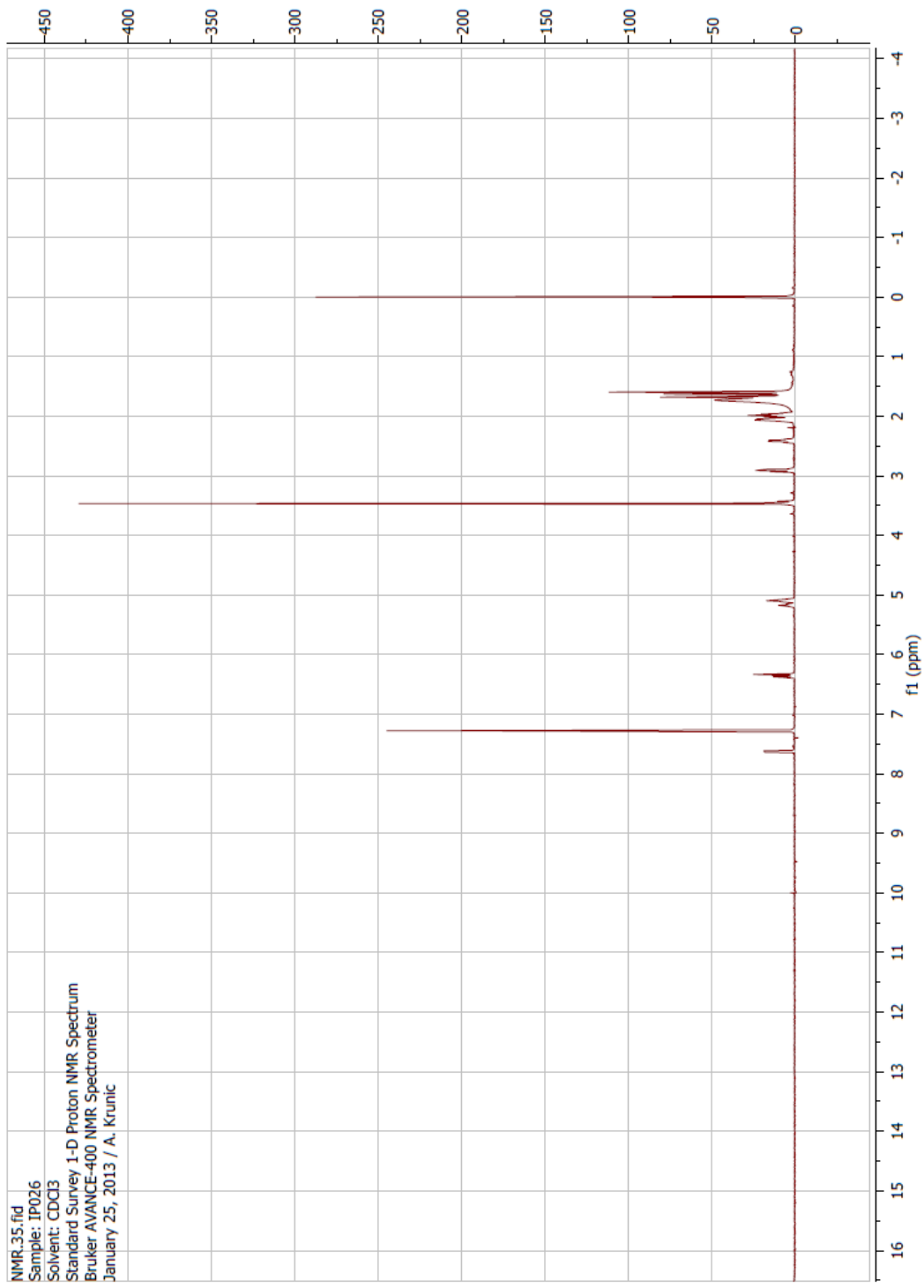
Slika 59. 1 H NMR spektar jedinjenja 4
