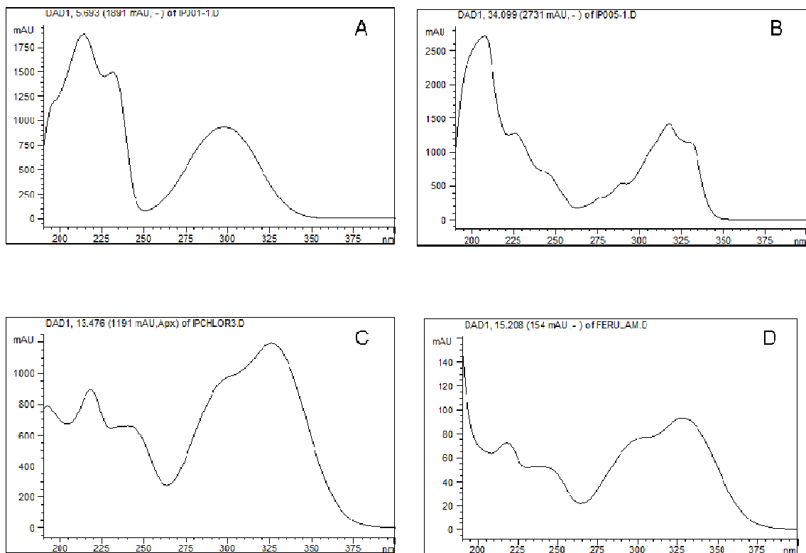
Slika 24. UV spektri jedinjenja identifikovanih u MeOH ekstraktu podzemnih organa F. heuffelii : A – jedinjenja 1 (latifolona); B – jedinjenja 6 ( 2S^*,3R^* )-2-[( 3E )-4,8-dimetilnona-3,7-dien-1-il]-2,3-dihidro-7-hidroksi-2,3-dimetilfuro[3,2- c ]kumarina); C – jedinjenja 11 (hlorogenske kiseline); D – jedinjenja 12 (3,5-dikafeoilhina kiseline).
