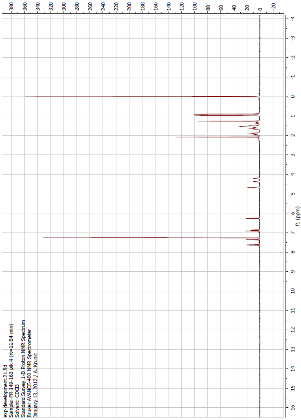
Slika 70. 1 H NMR spektar jedinjenja 7
