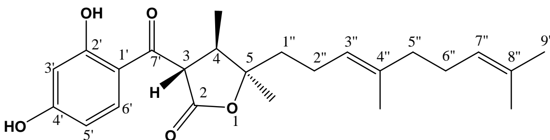
Slika 13. Jedinjenje 5 ((3 S *,4 R *,5 R *)-3-(2,4-dihidroksibenzoil)-5-[(3 E ,7 E )-4,8-dimetilnona-3,7-dien-1-il]tetrahydro-4,5-dimetilfuran-2-on)
