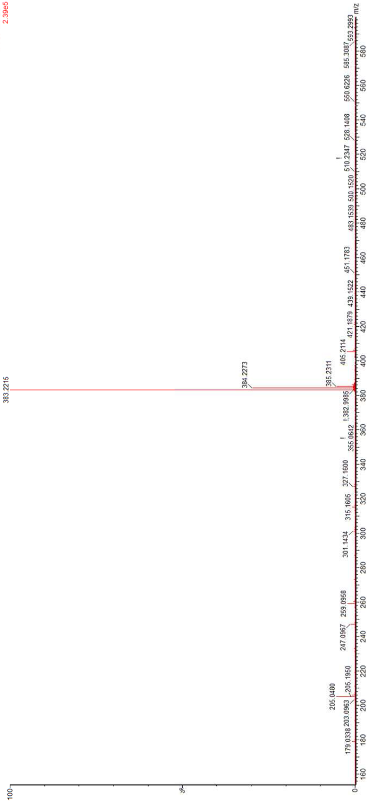
Slika 76. HR-MS spektar jedinjenja 9
