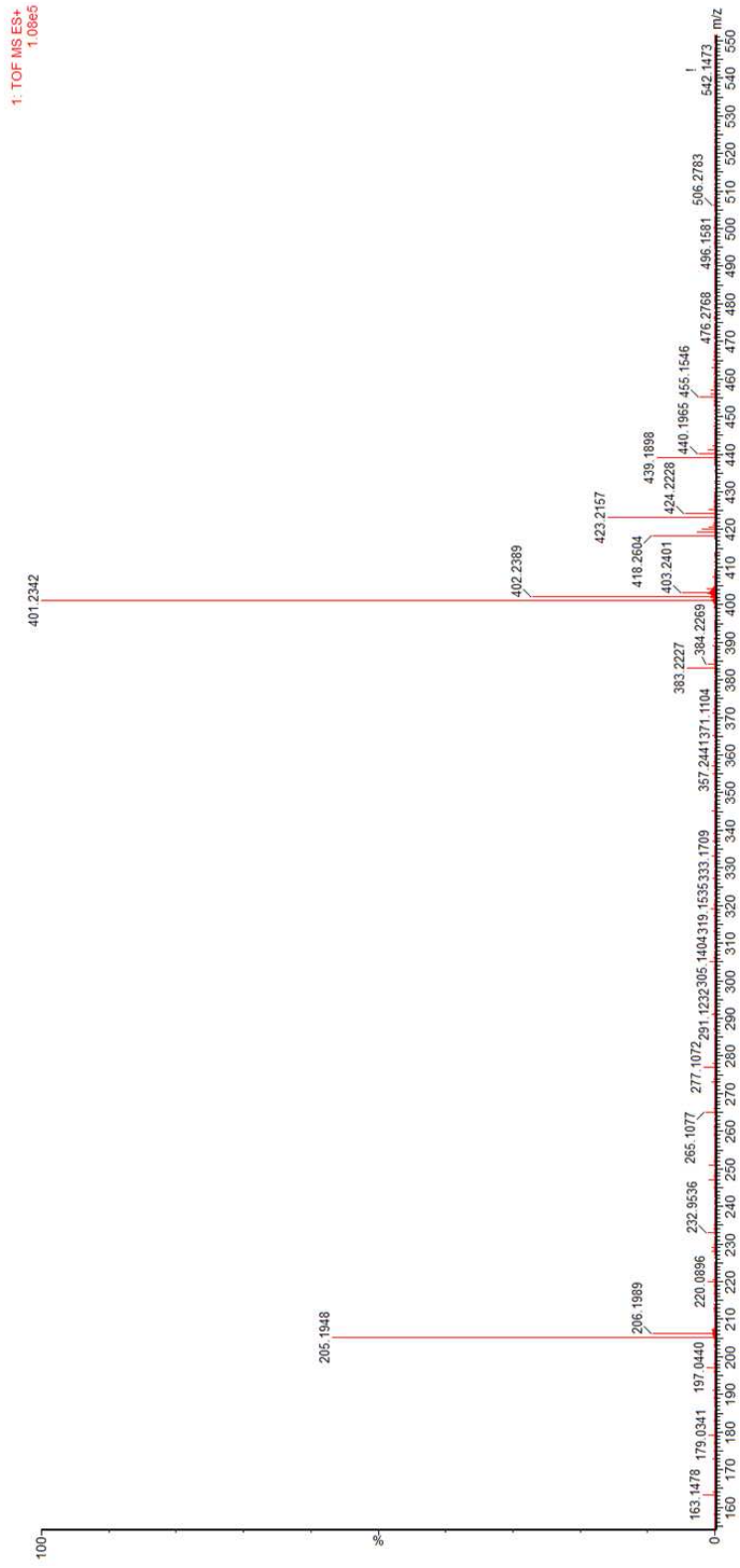
Slika 72. HR-MS spektar jedinjenja 8
