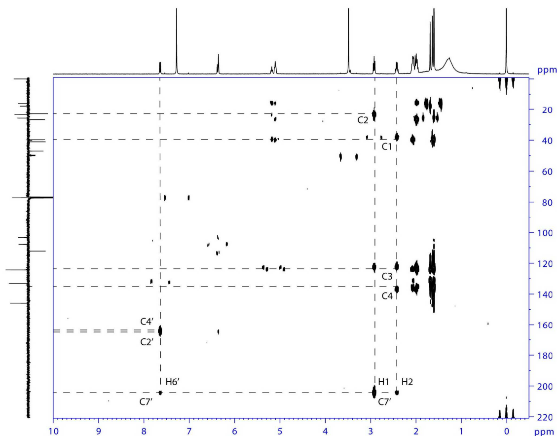
Slika 12. ^1\text{H} - ^{13}\text{C} HMBC spektar jedinjenja 4. Projekcija po F1 osi predstavlja snimljeni DEPTQ-135 spektar, a po F2 protonski spektar. Na slici su prikazane neke od važnijih korelacija.
