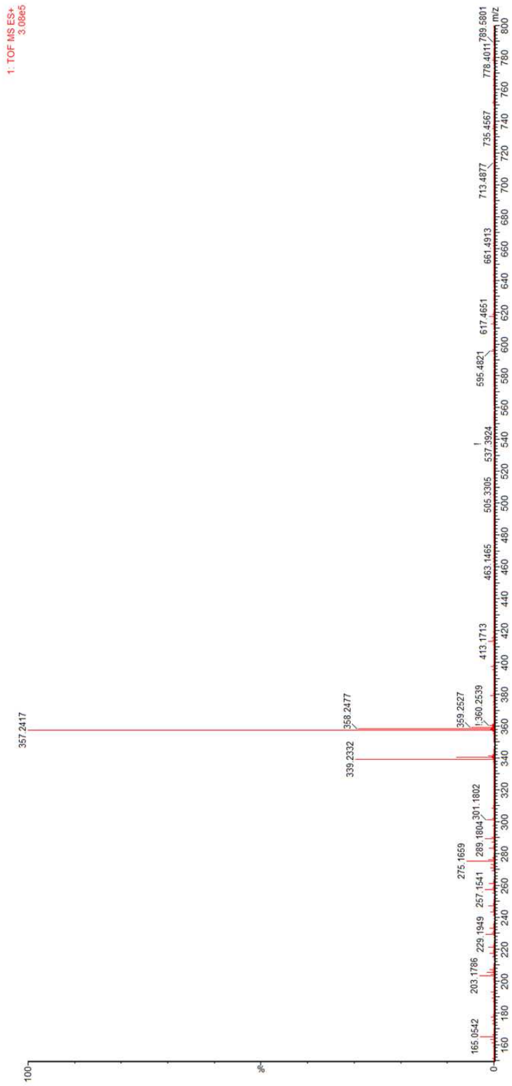
Slika 58. HR-MS spektar jedinjenja 4
