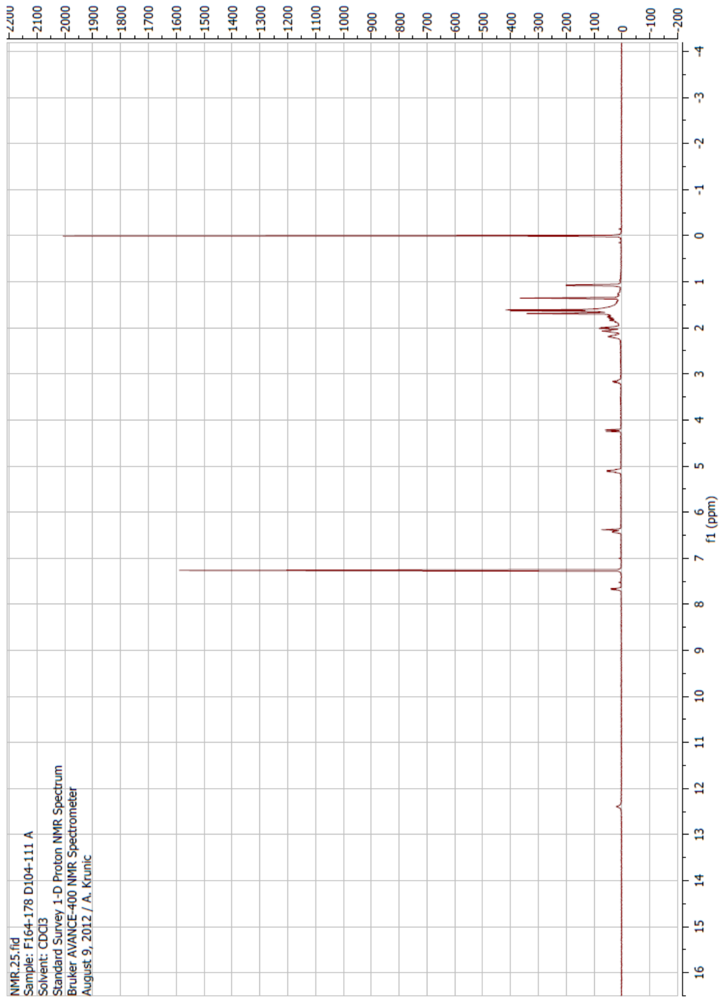
Slika 73. 1 H NMR spektar jedinjenja 8
