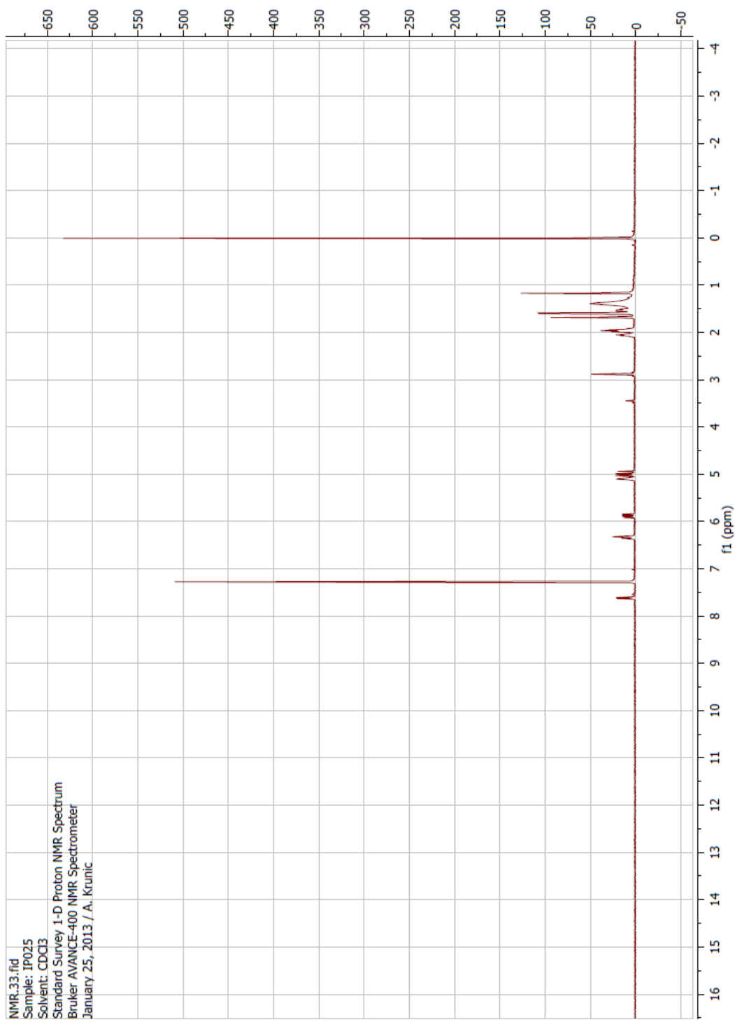
Slika 56. ^1\text{H} NMR spektar jedinjenja 3
