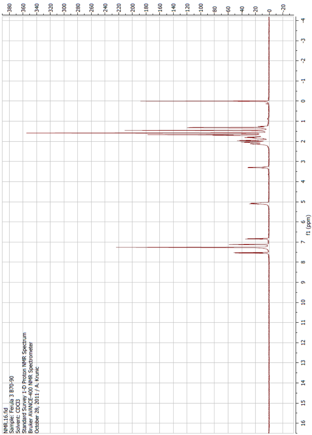
Slika 66. ^1\text{H} NMR spektar jedinjenja 6
