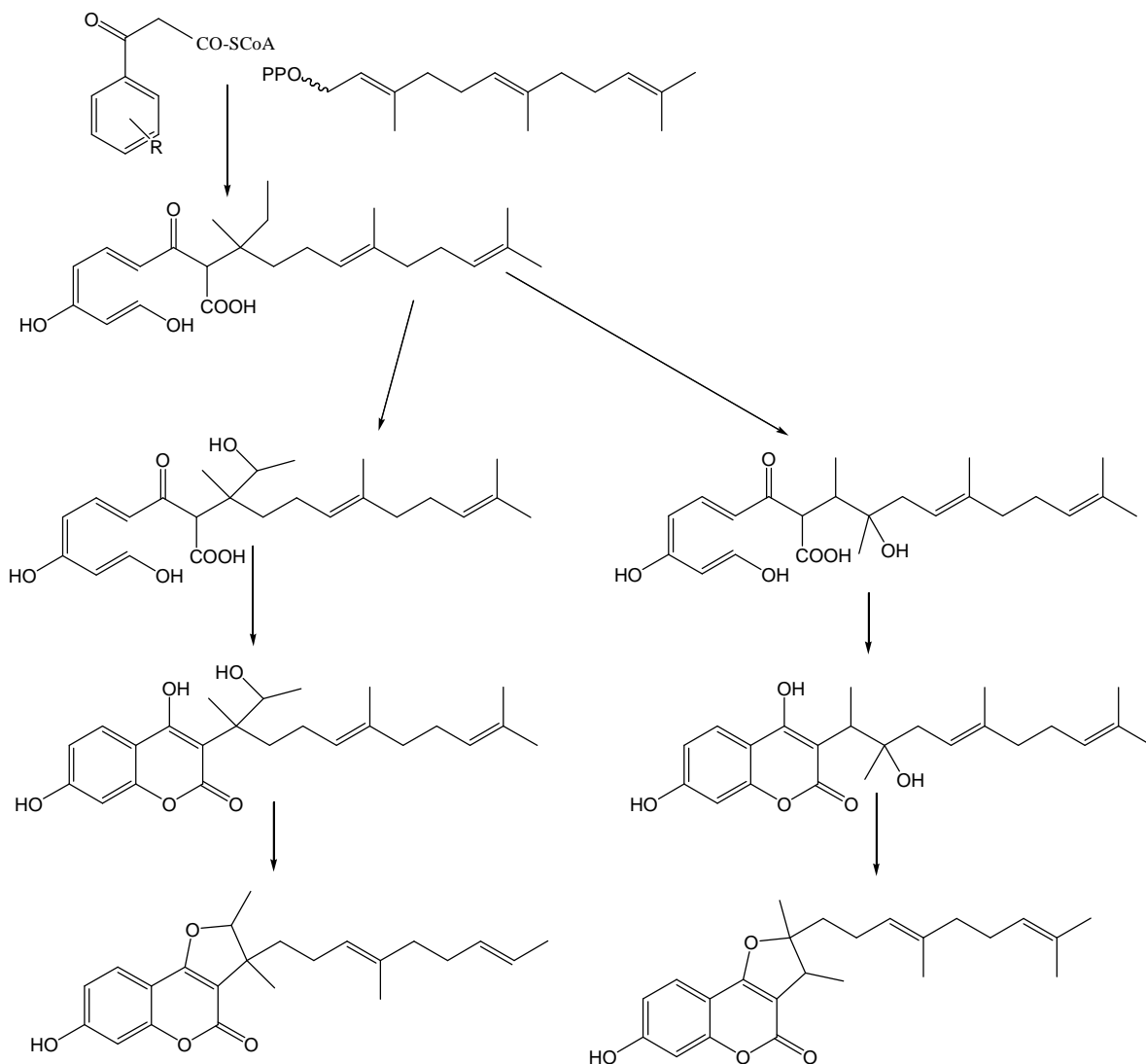
Slika 4. Potencijalni put biosinteze seskviterpena prenil-furokumarinskog tipa (Isaka i sar., 2001)
