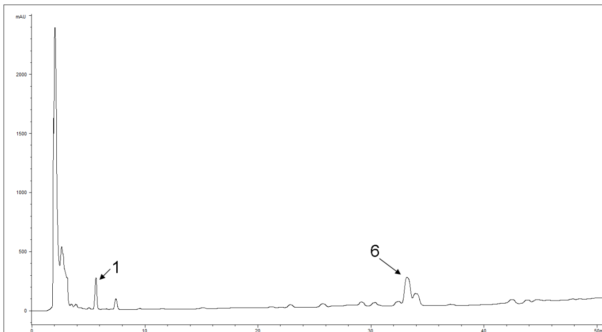
Slika 23. HPLC hromatogram korišćen za kvantifikovanje jedinjenja 1 i 6 . Binarna mobilna faza bila je: A – voda i B – smeša acetonitril:metanol (3:1), a metoda korišćena za kvantifikovanje: A:B (40:60-20:80) u toku 30 min, nakon toga u toku 5 min eluiranje je nastavljeno u izokratskim uslovima i nakon toga A:B (20:80-5:95) u toku 15 min, pri čemu je volumen injektovanja izosio 20 \mu l, temperatura 25 °C i brzina protoka 1 ml/min.
