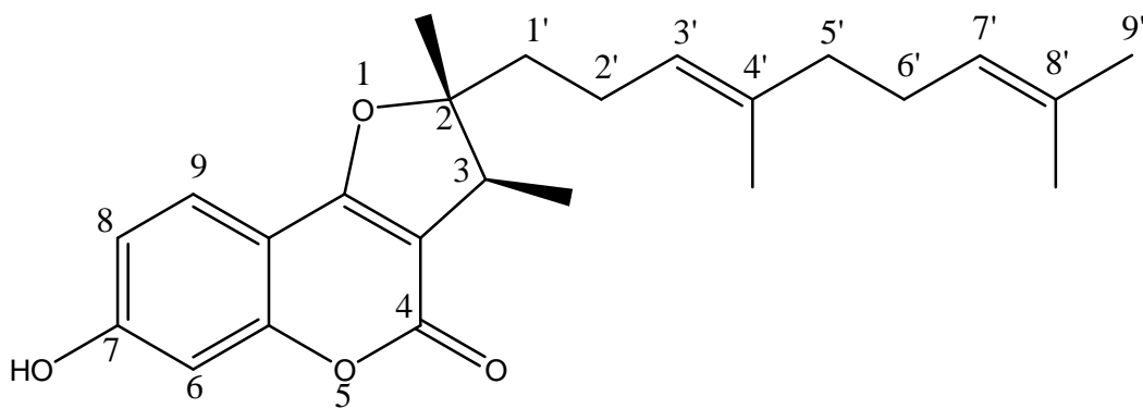
Slika 14. Jedinjenje 6 ((2 S *,3 R *)-2-[(3 E )-4,8-dimetilnona-3,7-dien-1-il]-2,3-dihidro-7-hidroksi-2,3-dimetilfuro[3,2- c ]kumarin)
