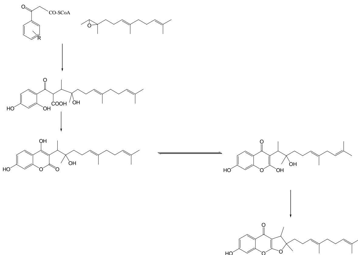
Slika 5. Mogući put biosinteze seskviterpena prenil-furohromonskog tipa (Meng i sar., 2013)
