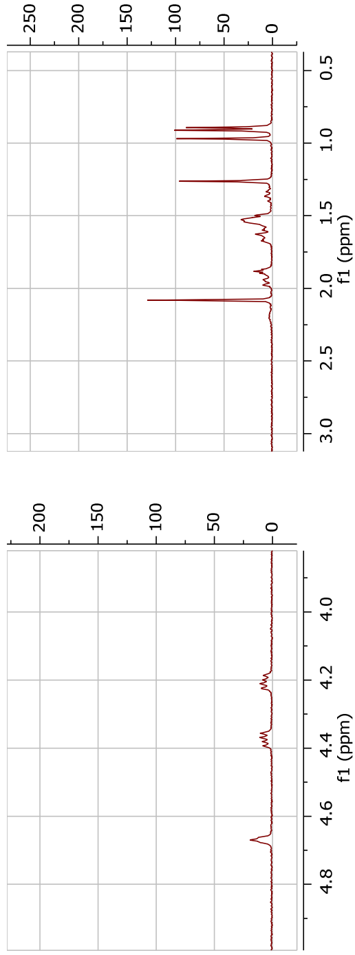
Slika 71. Prošireni detalji ^1\text{H} NMR spektra jedinjenja 7
