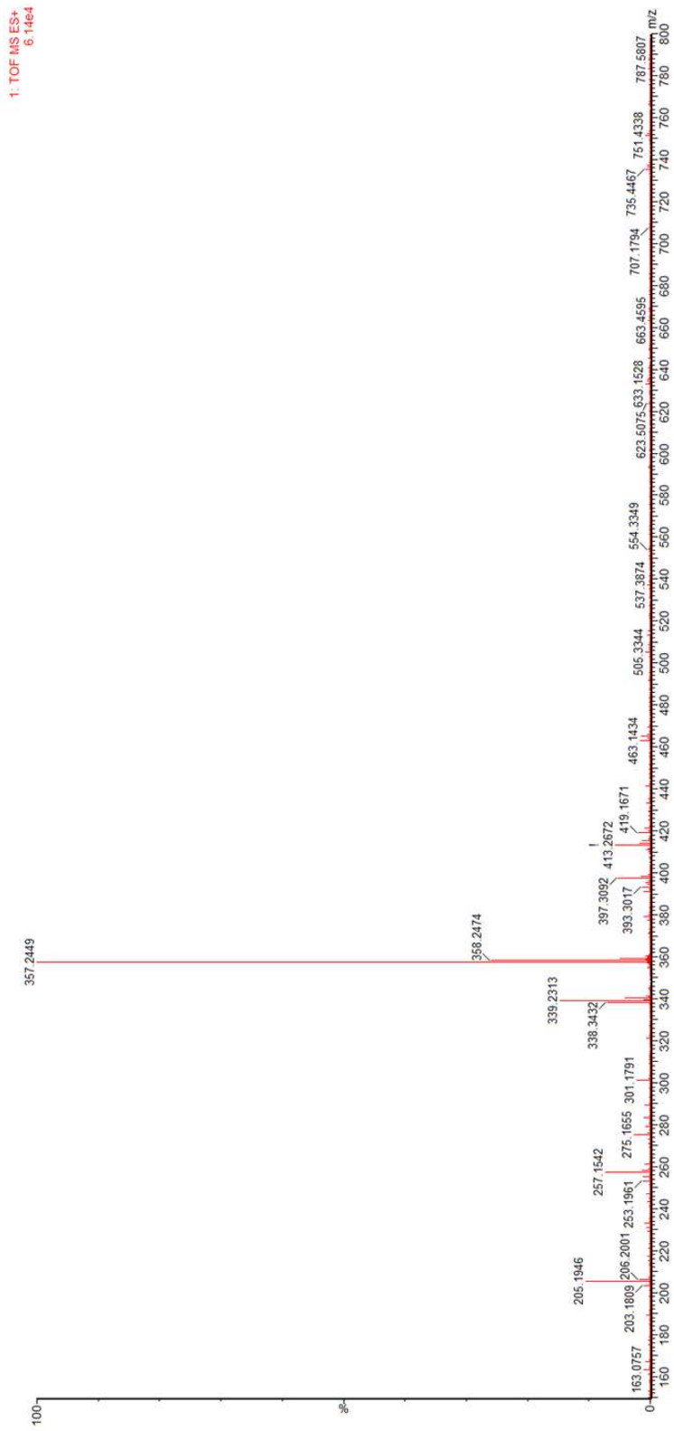
Slika 55. HR-MS spektar jedinjenja 3
