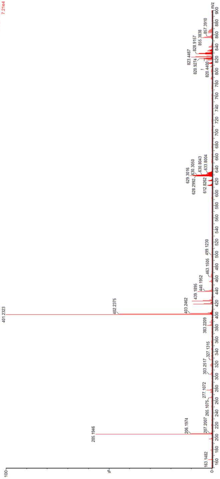
Slika 62. HR-MS spektar jedinjenja 5
