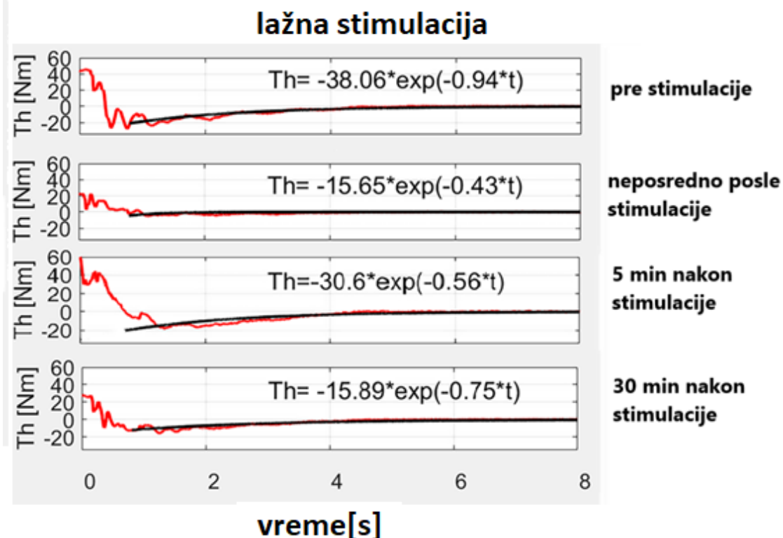
Slika 7. 4. Rezultati za prvog subjekta sa lažnom stimulacijom. Simulirani spastični moment T_h je obeležen crvenom linijom, a njegov eksponencijalni fit crnom bojom. SPAS procena kod ovog subjekta varira od 1.2 do 3.2. Preuzeto i modifikovano iz [25].
