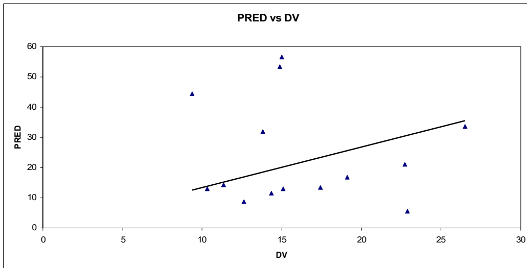
Графикон 6. Однос између предвиђених популационих (PRED) насупрот измерених серумских (DV) концентрација 25-хидрокси витамина D у коначном ПФК моделу валидационог сета
