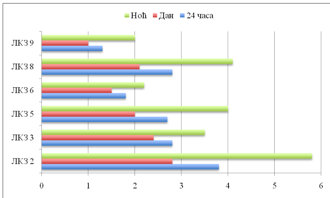
Прилог 42. Разлика у вредностима UTCI индекса између градских ЛКЗ (ЛКЗ x ) и ЛКЗ А изван града (ЛКЗ x-A ) у Новом Саду током топлотног таласа на нивоу: 24 часа, обданице и ноћи. Топлотни талас је трајао од 4. до 15. августа 2015. године
