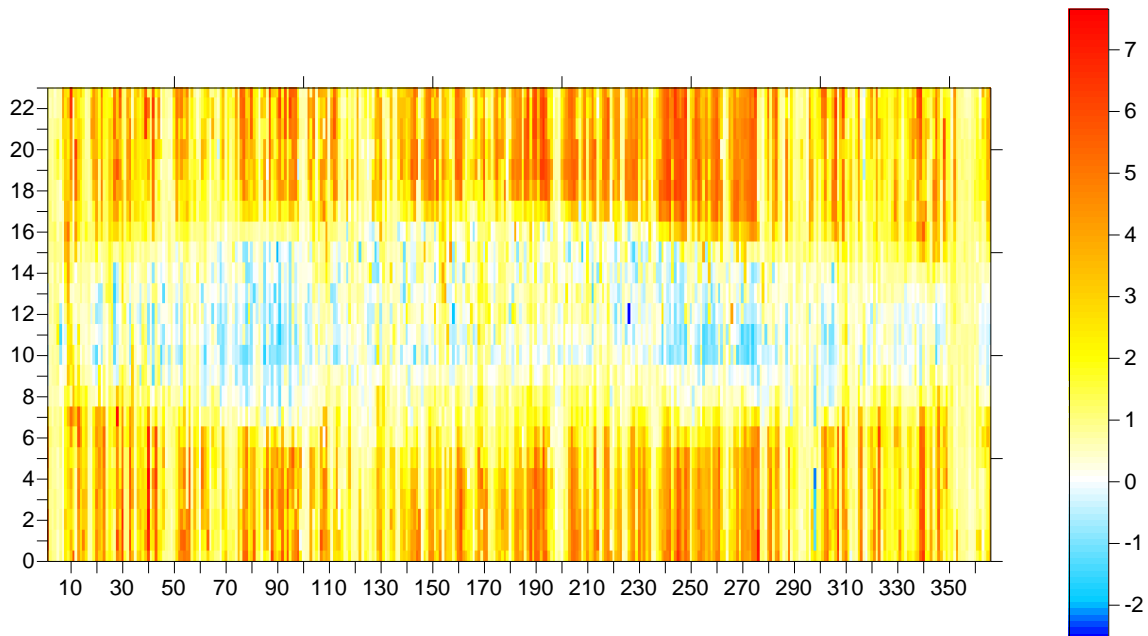
Прилог 27. Годвише и дневне разлике у T_{sr} између изграђене ЛКЗ 2 и природне ЛКЗ А у Новом Саду. На у-оси су представљени часови (у UTC), а на х-оси су представљени дани у години
