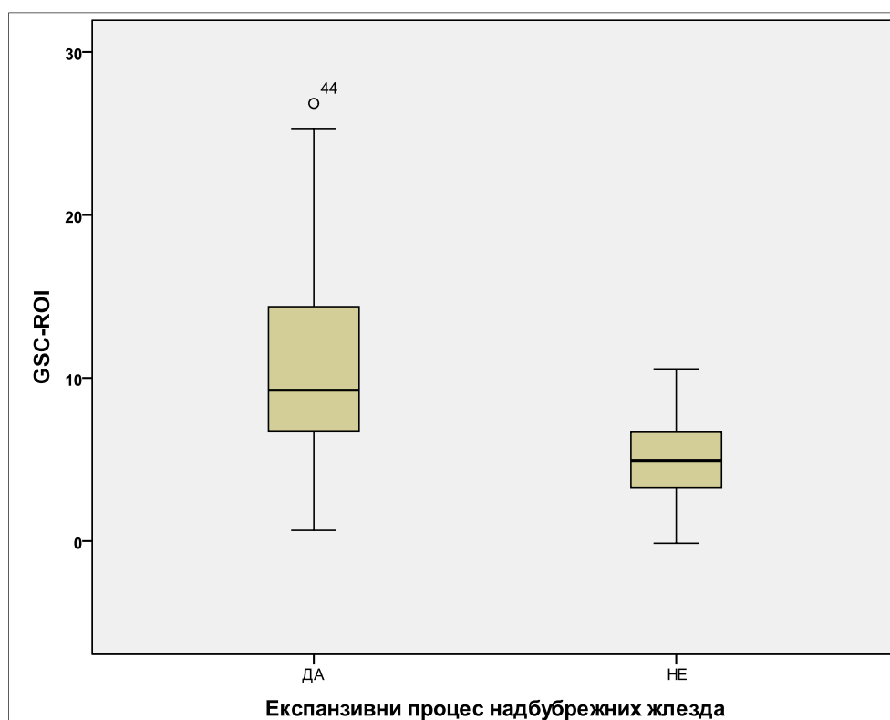
Графикон 4.25. Вредности GSC-ROI са ^{99m}\text{Tc(V)-DMSA} у испитиваној популацији у зависности од постојања тумора надбубрежних жлезда Вредности GSC-ROI са ^{99m}\text{Tc(V)-DMSA} биле су статистички значајне између групе испитаника са дијагностикованим тумором надбубрежних жлезда ( 10,56 \pm 6,74 ) у односу на испитанике без постављене дијагнозе тумора надбубрежних жлезда ( 5,08 \pm 2,53 ), анализирано Т-тестом независних узорака ( t(44) = 3,365 , p = 0,02 ; разлика између средњих вредности обележја по групама: просечна разлика = 5,47, 95% CI: 2,19 до 8,75).
