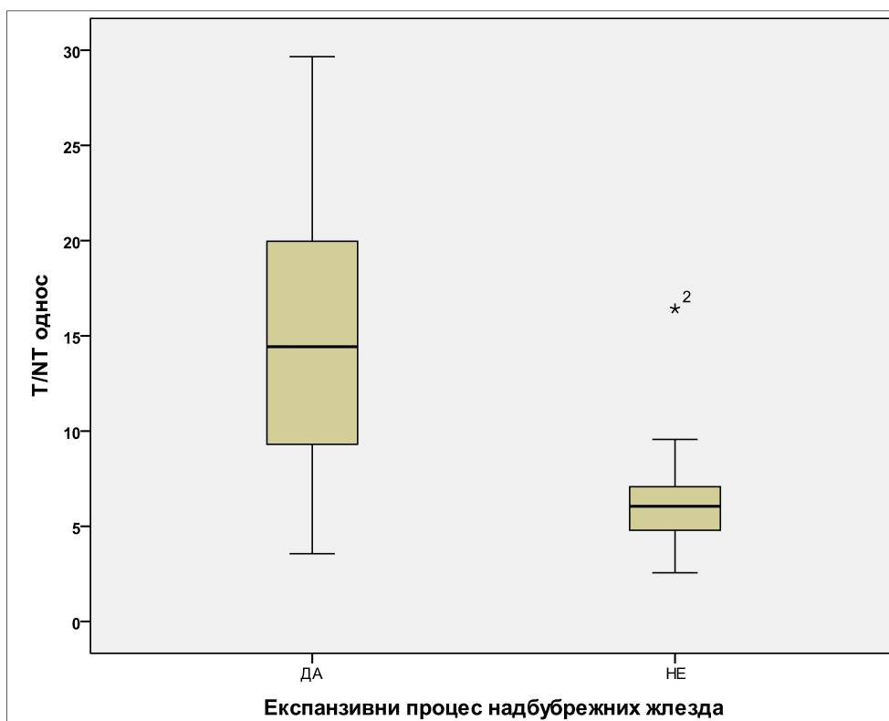
Графикон 4.23. Вредности T/NT односа са ^{99m}\text{Tc-HYNIC-TOC} у испитиваној популацији у зависности од постојања тумора надбубрежних жлезда
