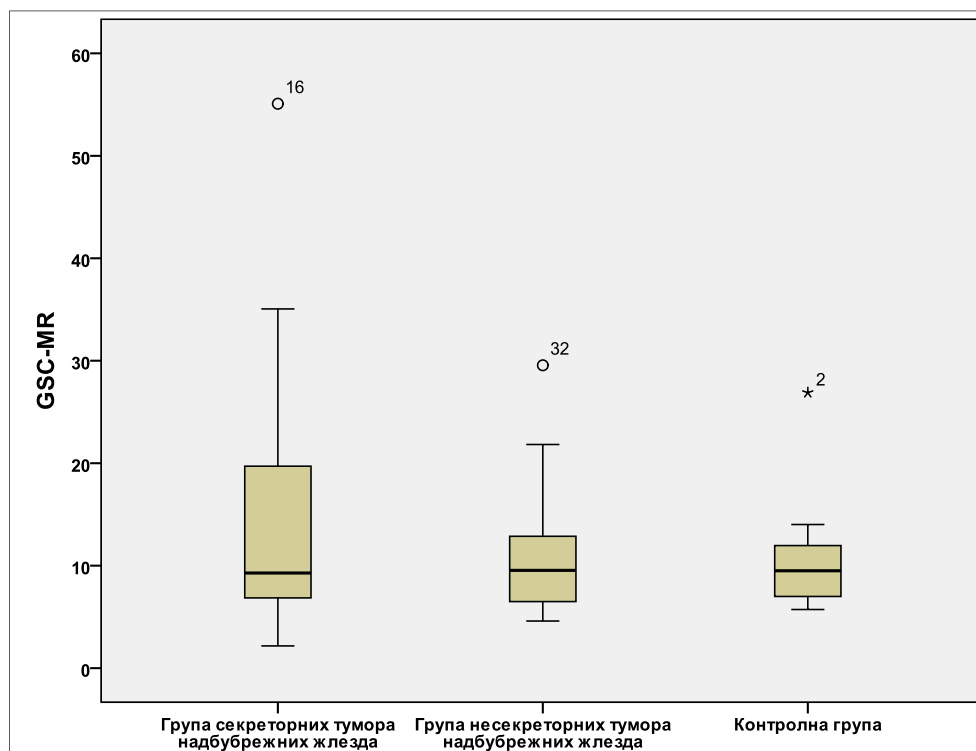
Графикон 4.38. Вредности GSC-MR са ^{99m}\text{Tc-HYNIC-TOC} у испитиваној популацији у зависности од секреторне активности тумора надбубрежних жлезда
