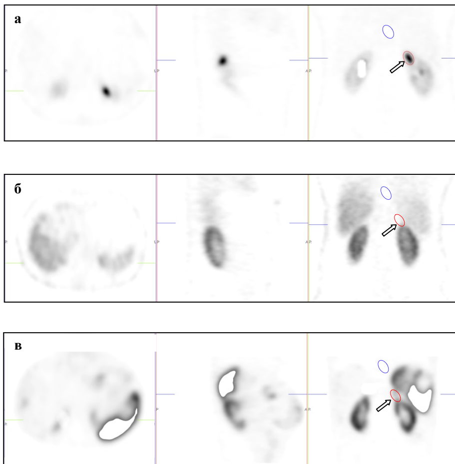
Слика 3.4. Семиквантитативна анализа експанзивних процеса надбубрежних жлезда
