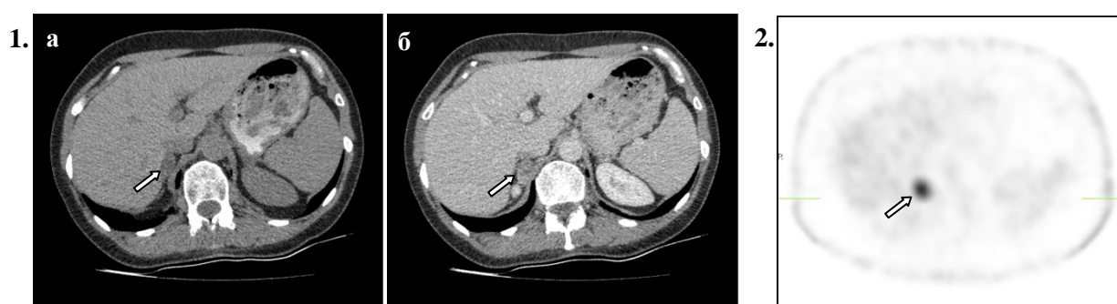
Слика 3.2. Квалитативна анализа експанзивних процеса надбубрежних жлезда
