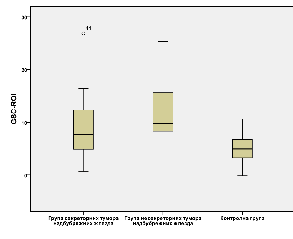
Графикон 4.34. Вредности GSC-ROI са ^{99m}\text{Tc(V)}\text{-DMSA} у испитиваној популацији у зависности од секреторне активности тумора надбубрежних жлезда
