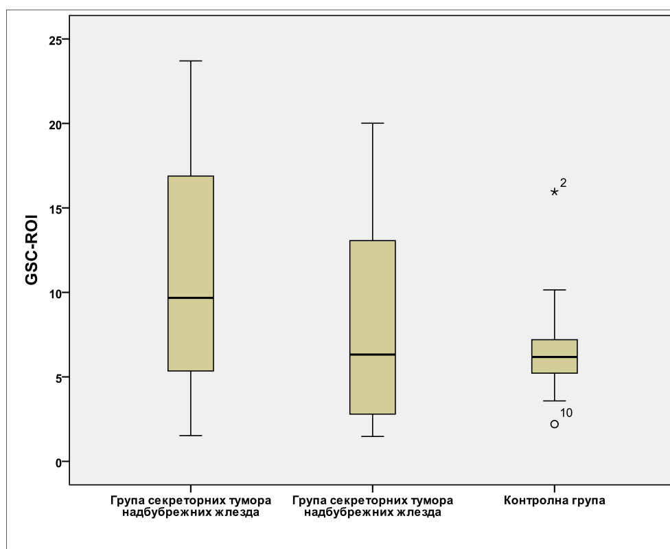
Графикон 4.33. Вредности ROI са ^{99m}\text{Tc-MIBI} у испитиваној популацији у зависности од секреторне активности тумора надбубрежних жлезда Вредности ROI са ^{99m}\text{Tc-MIBI} , у све три групе испитаника, анализирани су Kruskal-Wallis-овим тестом и није забележена статистички значајна разлика између група ( \chi^2(2, 46)=2,079 , p>0,05 ). Медијана резултата испитаника са дијагнозом секреторног тумора надбубрежних жлезда ( Md=9,67 ) била је већа у односу на медијану резултата испитаника ( Md=6,32 ) са дијагностикованим несекреторним тумором надбубрежних жлезда ( p>0,05 ), као и медијану резултата ( Md=6,17 ) контролне групе ( p>0,05 ).
