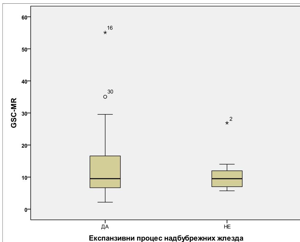
Графикон 4.29. Вредности GSC-MR са ^{99m}\text{Tc} -HYNIC-TOC у испитиваној популацији у зависности од постојања тумора надбубрежних жлезда Вредности GSC-MR са ^{99m}\text{Tc} -HYNIC-TOC нису биле статистички значајне у групи испитаника са постављеном дијагнозом тумора надбубрежних жлезда ( Md=9,51 ) у односу на испитанике без постављене дијагнозе тумора надбубрежних жлезда ( Md=9,49 ) анализирано путем Mann-Whitney-евог U-теста ( U=239,000 , z=-0,390 , p>0,05 , r=0,06 ).
