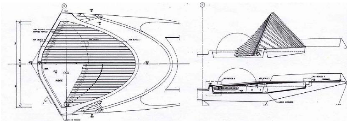
Сл.124 Цртеж улазног дела / entrance (А.Тзонис, "S. Calatrava, The Poetics of Movement", London 1999)
