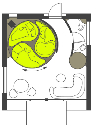
Сл.61 Grundriss Rotor- Modulhaus 121 , (Прилог преузет из књиге "Moving Architecture" ,Vienna UT / Alexander Greil, 2014:Str 76)
