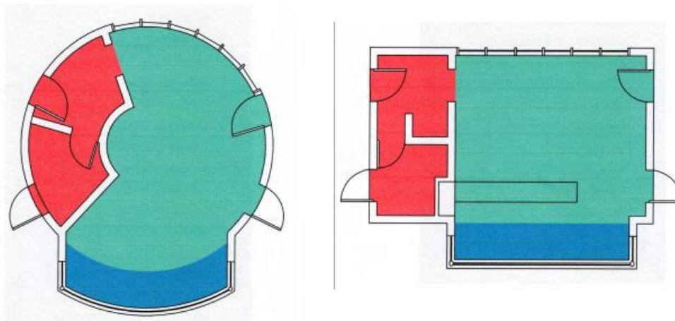
Сл.81. Приказ успоредбе кружне основе куће Омо и постојеће основе куће Омо (аутор приложеног прилога А. Фотиадоу, 2011.) 139
