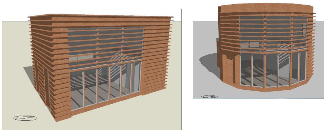
Сл. 83 показује структуру објекта у примарној форми и у новонасталој кружној форми (3Д приказ модела, А. Фотиадоу, 2011)
